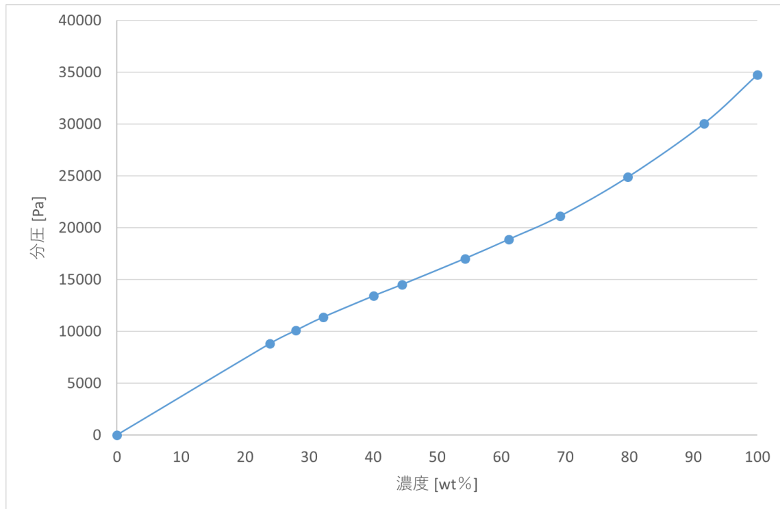
第5図 温度39.9℃におけるメタノール濃度の違いによる分圧の変化
