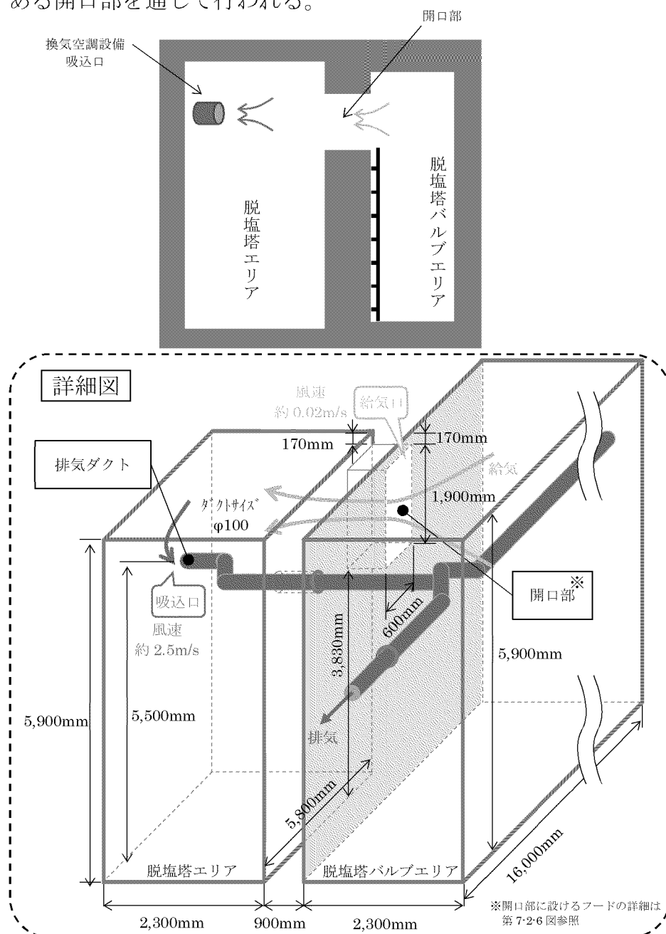
第 7-2-5 図 脱塩塔エリアの詳細図
