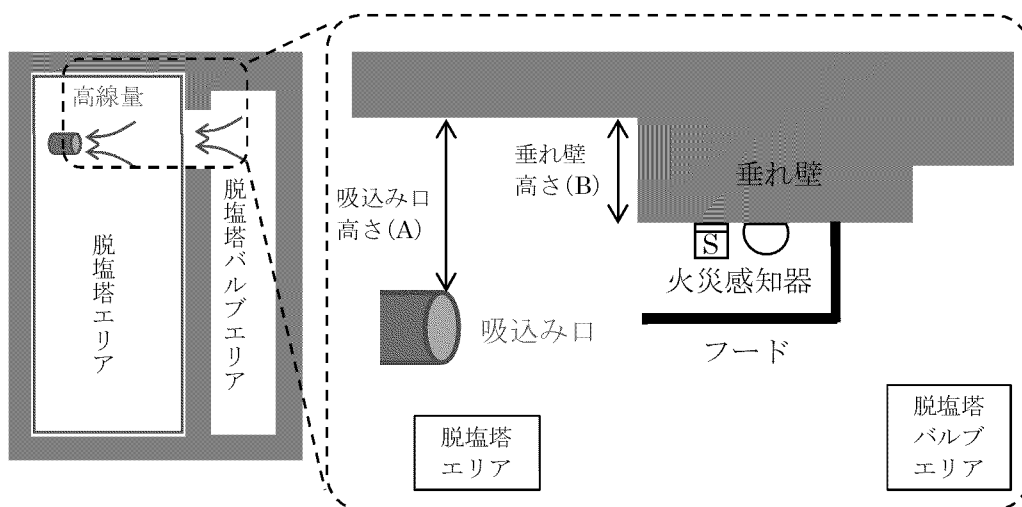
図 2 脱塩塔エリアの火災感知に係る建屋及び吸込み口の位置関係概要図
