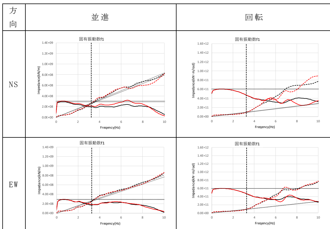
第 5.1.1-1 図 燃料加工建屋の地盤インピーダンスの比較
