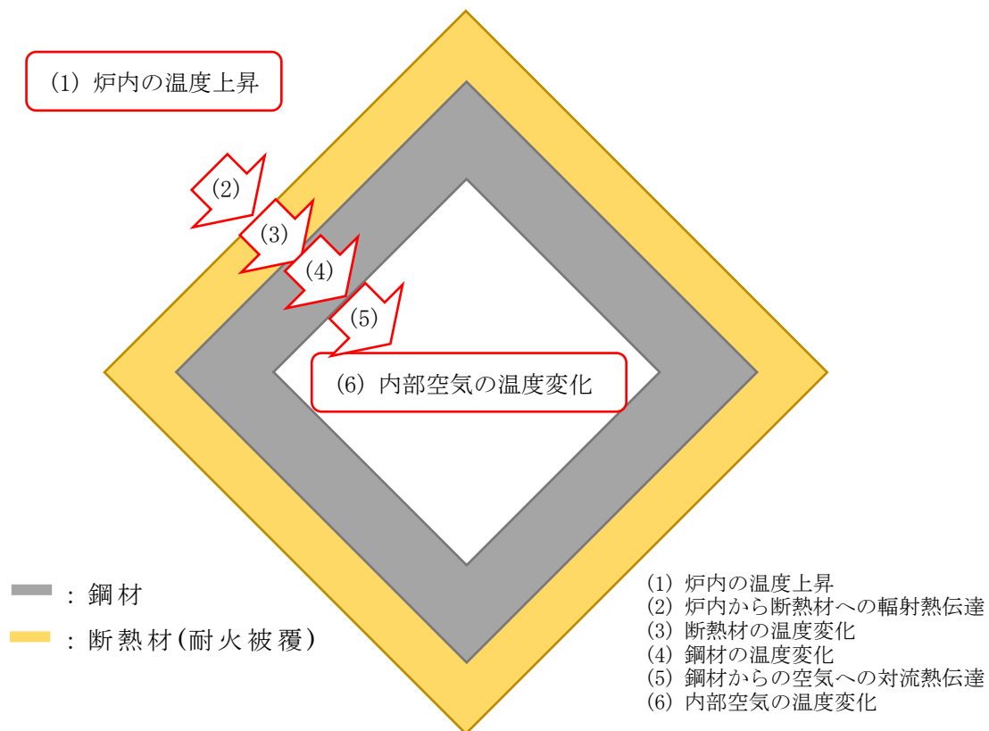
第 1 図 鋼材温度評価の評価モデル
