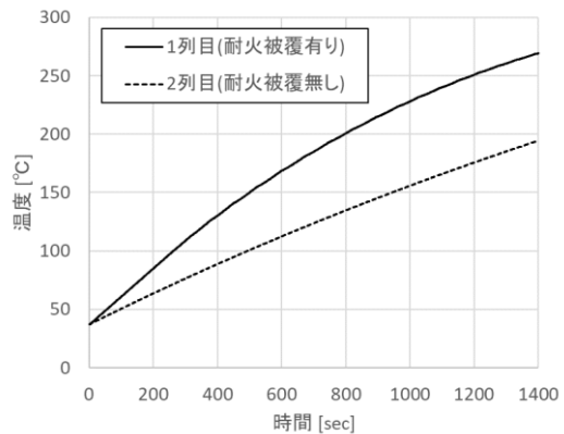
第 2-3 図 部材の温度評価結果
