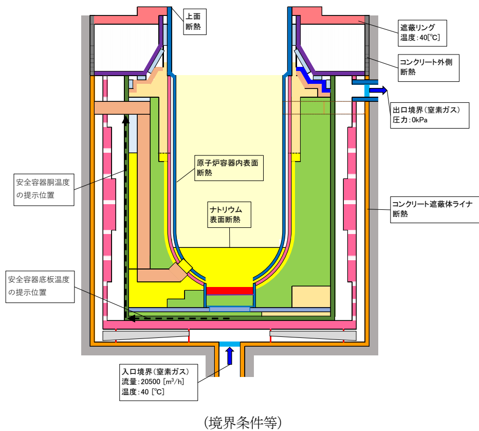
第 4.3.3.9.9 図 FLUENTにおける解析体系等
