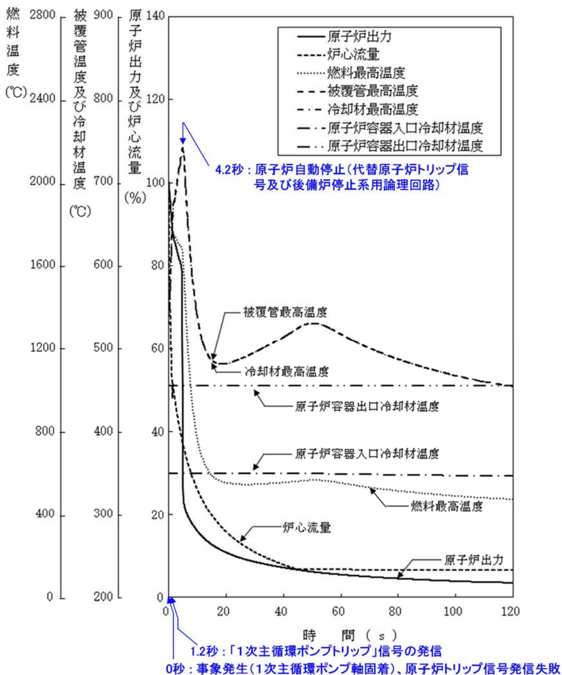
第 4.3.3.3.3 図 1 次主循環ポンプ軸固着及び原子炉トリップ信号発信失敗の重畳事故 (炉心損傷防止措置：代替トリップ信号及び後備炉停止制御棒による原子炉停止)
