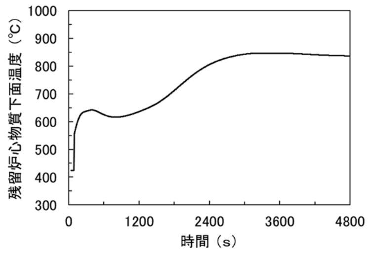
第 4. 3. 3. 3. 19 図 残留炉心物質下面の最高温度の履歴
