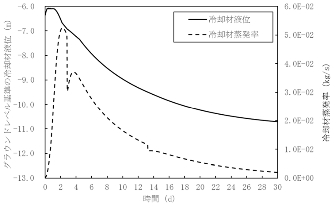
第 4. 3. 3. 13. 7 図 炉内事象推移の計算結果（原子炉容器内冷却材液位及び冷却材蒸発率の推移）
