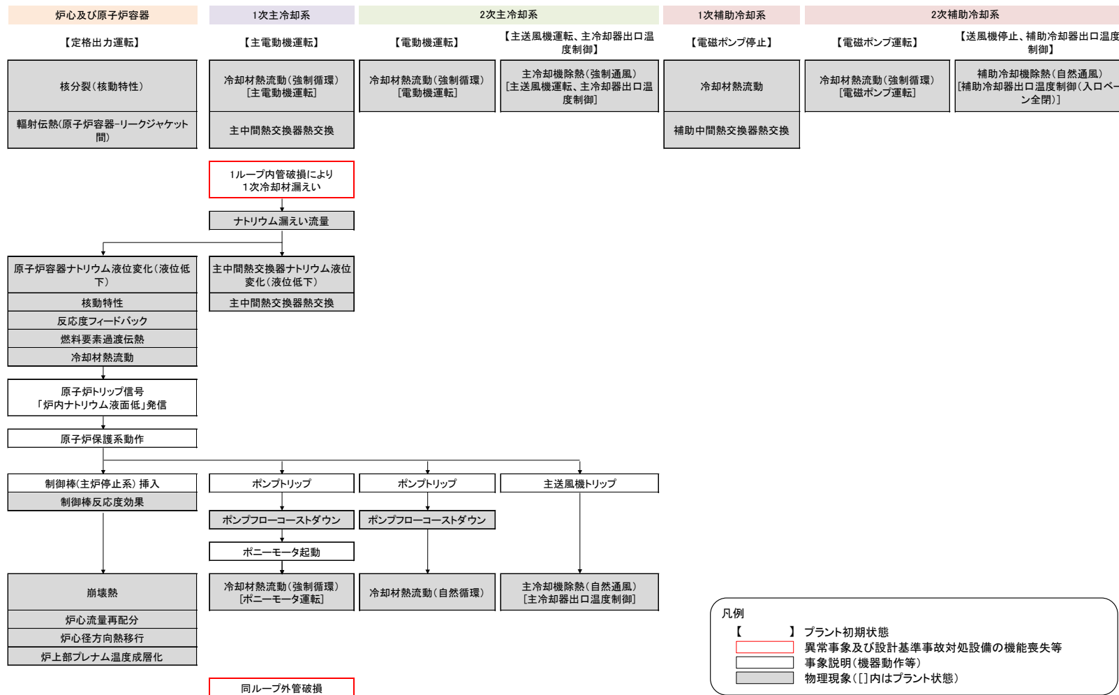
第 2. 2. 3. 2 図 格納容器破損防止措置 (LORL (ii)) の事象推移と物理現象 (1/2)
