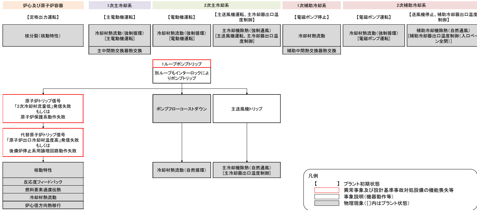
第 2. 2. 2. 1 図 格納容器破損防止措置 (ULOHS ( i ) 及び ULOHS ( ii )) の事象推移と物理現象
