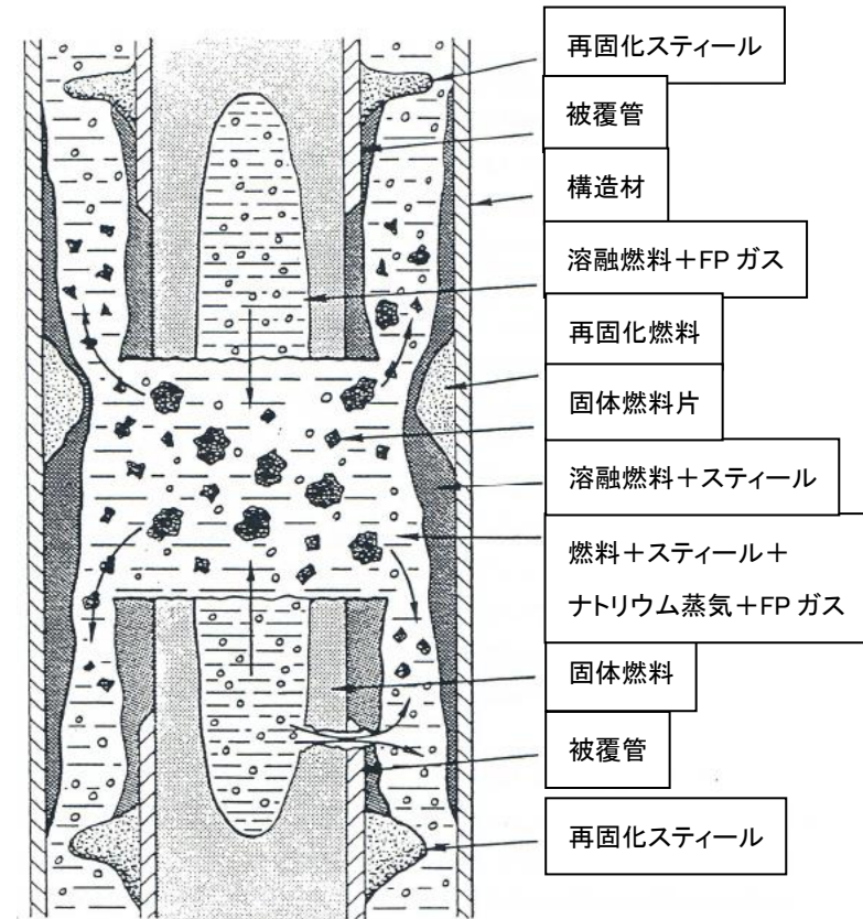
第 3.4 図 SAS4A の未沸騰時破損後挙動解析モデル（左図）と沸騰時破損後挙動解析モデル（右図）の概念 [3]
