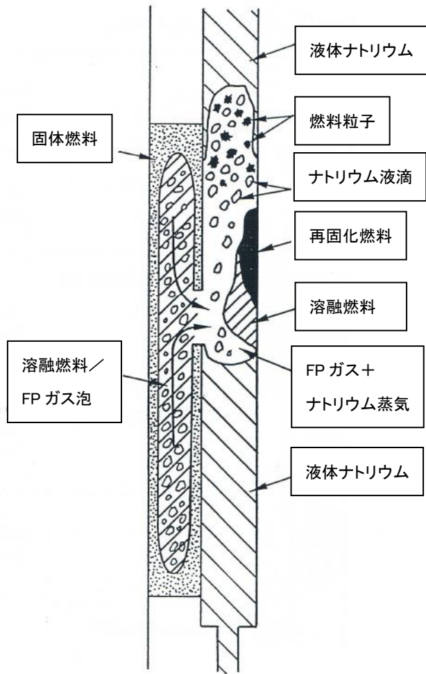
第 3.4 図 SAS4A の未沸騰時破損後挙動解析モデル（左図）と沸騰時破損後挙動解析モデル（右図）の概念 [3]
