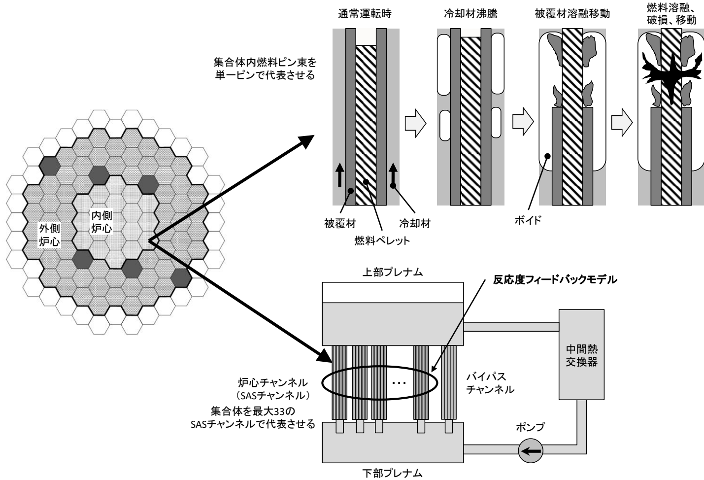
第 3.1 図 SAS 4 A の概念
