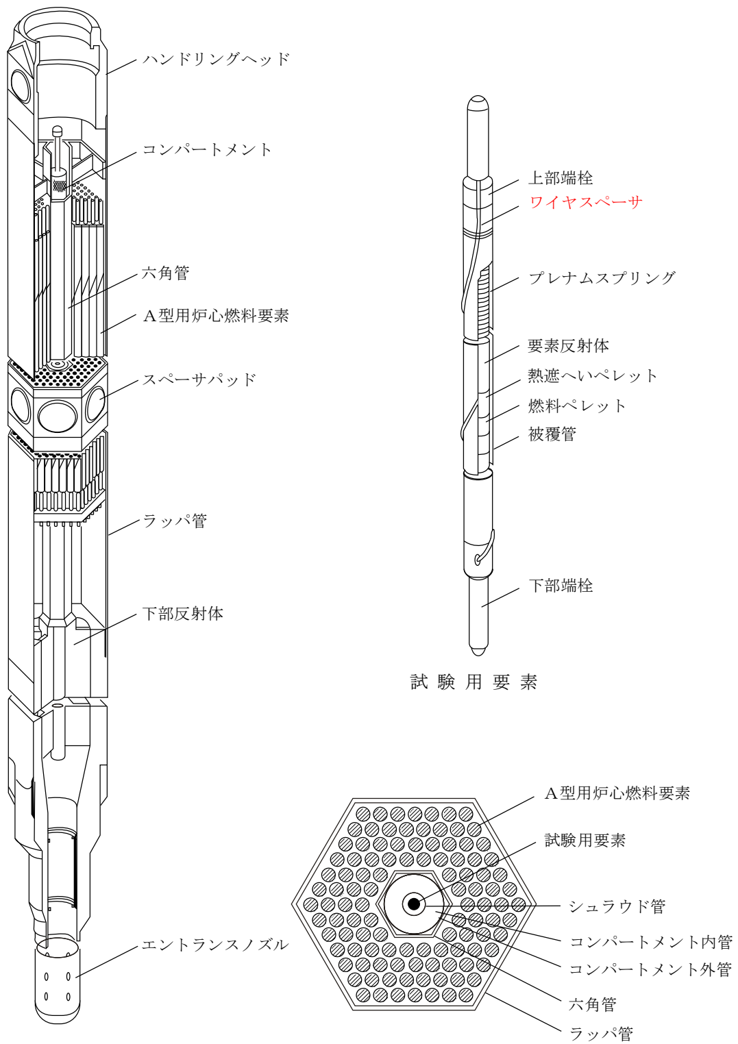
第 3.7.4 図 照射燃料集合体 (2/5) (参考用)
