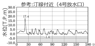
水位の時刻歴波形 (参考:汀線付近(4号放水口)) ・期望平均満潮位 T.P.+0.80mを考慮
