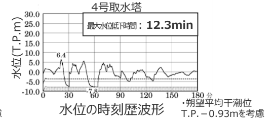
最大下降水位(T.P.m)(水位低下時間)
