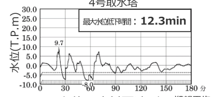
水位の時刻歴波形 (参考:汀線付近(4号放水口)) ・期望平均干潮位 T.P.-0.93mを考慮
