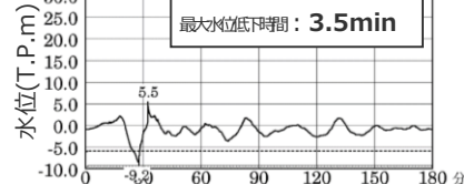
水位の時刻歴波形 ・朔望平均干潮位 T.P. - 0.93mを考慮
