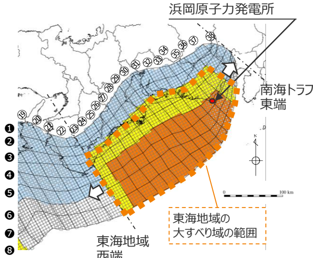
各小断層の配列 (検討波源モデルC)
