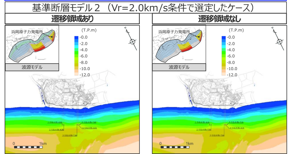
最大下降水位分布 3号取水塔
