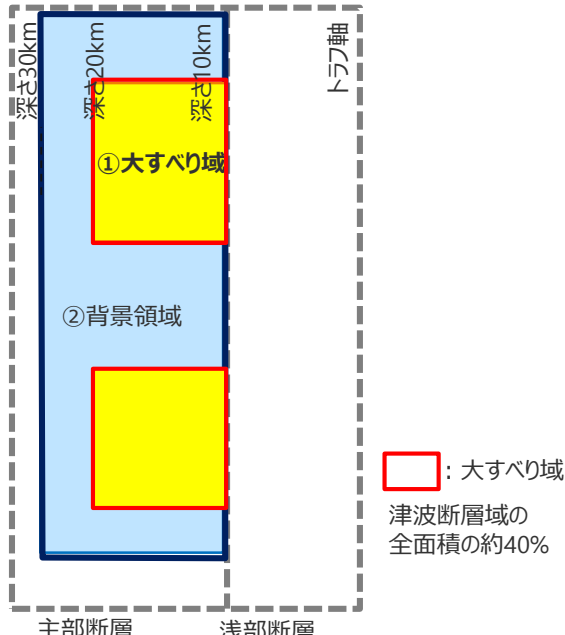
プレートの沈み込み速度を考慮したモデルの すべり量分布概念図
