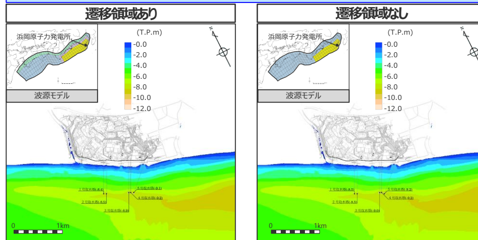
最大下降水位分布 3号取水塔
