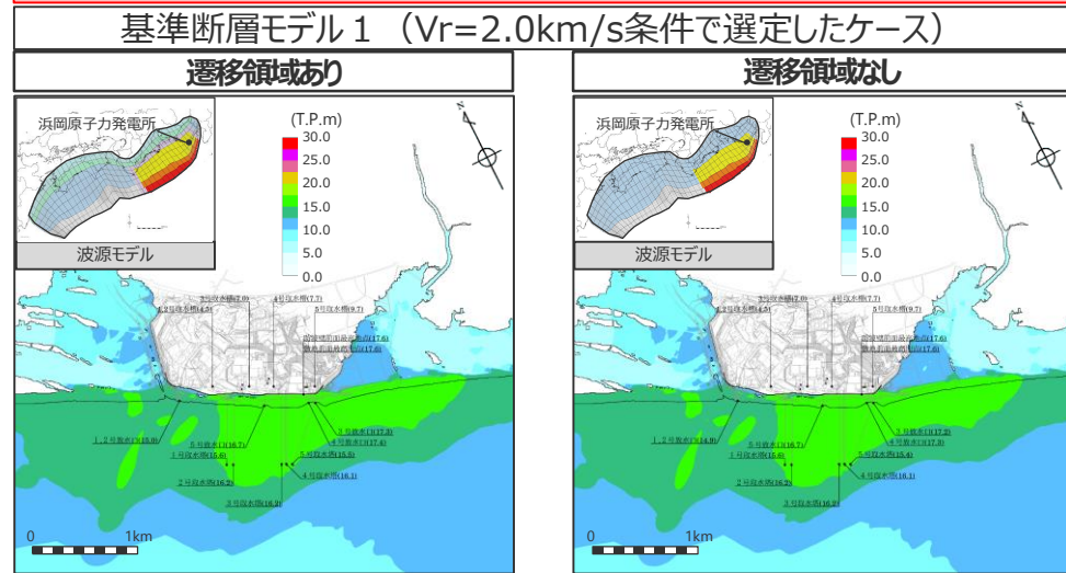
最大上昇水位分布 敷地前面
