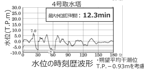
最大下降水位(T.P.m)(水位低下時間)
