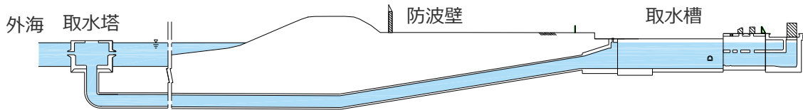
取水設備（取水塔～取水トンネル～取水槽）の縦断面図
