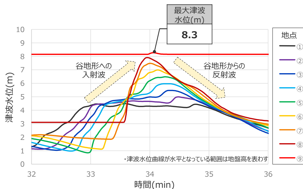
谷地形周辺（地点①～⑨）の津波水位の時間変化
