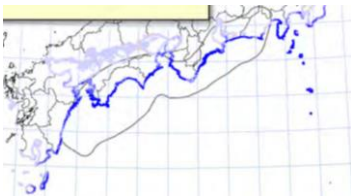
東側モデルに対して、 40分前に西側モデルが発生
