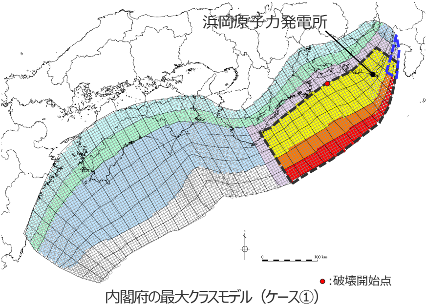
内閣府の最大クラスモデル（ケース①）と検討波源モデルAの最大ケースとの比較分析
