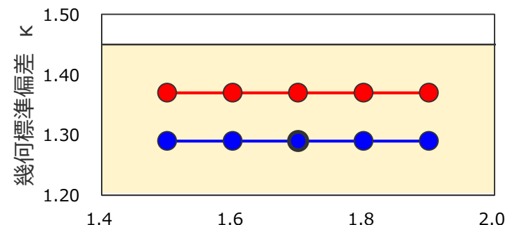
プレートの沈み込み速度を 考慮しないモデル
