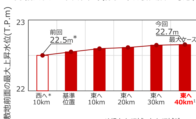
○詳細パラメータスタディ結果（破壊伝播を考慮）
