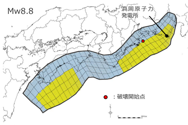
南海トラフ広域の痕跡再現モデル (特性化モデル)
