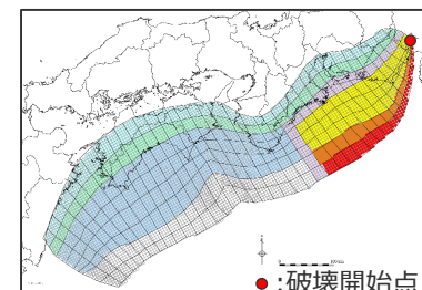
検討波源モデルAの最大ケース
