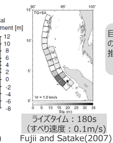
2004年スマトラ島沖地震
