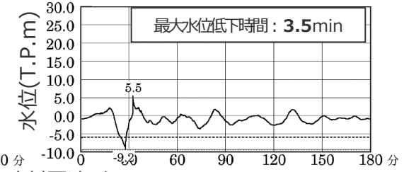
水位の時刻歴波形
