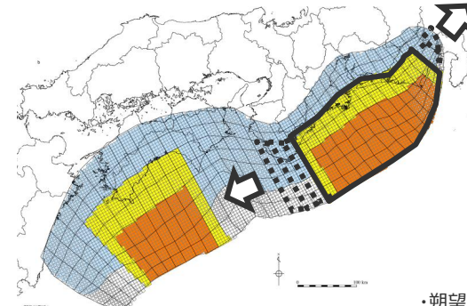
検討波源モデルC 水位上昇側
