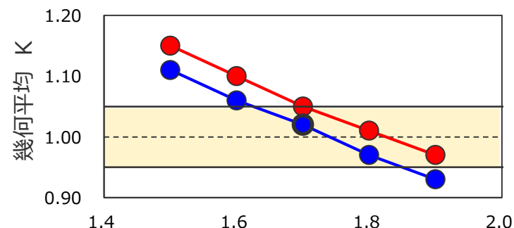
プレートの沈み込み速度を 考慮したモデル
