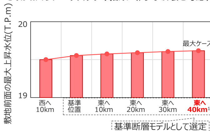
○概略パラメータスタディ結果（同時破壊を考慮）
