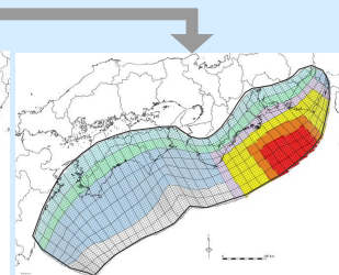
検討波源モデルD
