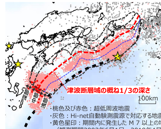
(観測期間2003年6月1日~2019年4月30日) (防災科学技術研究所(2020)を基に作成) 南海トラフの浅部超低周波地震の分布との関係
