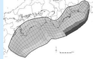
検討波源モデルA
