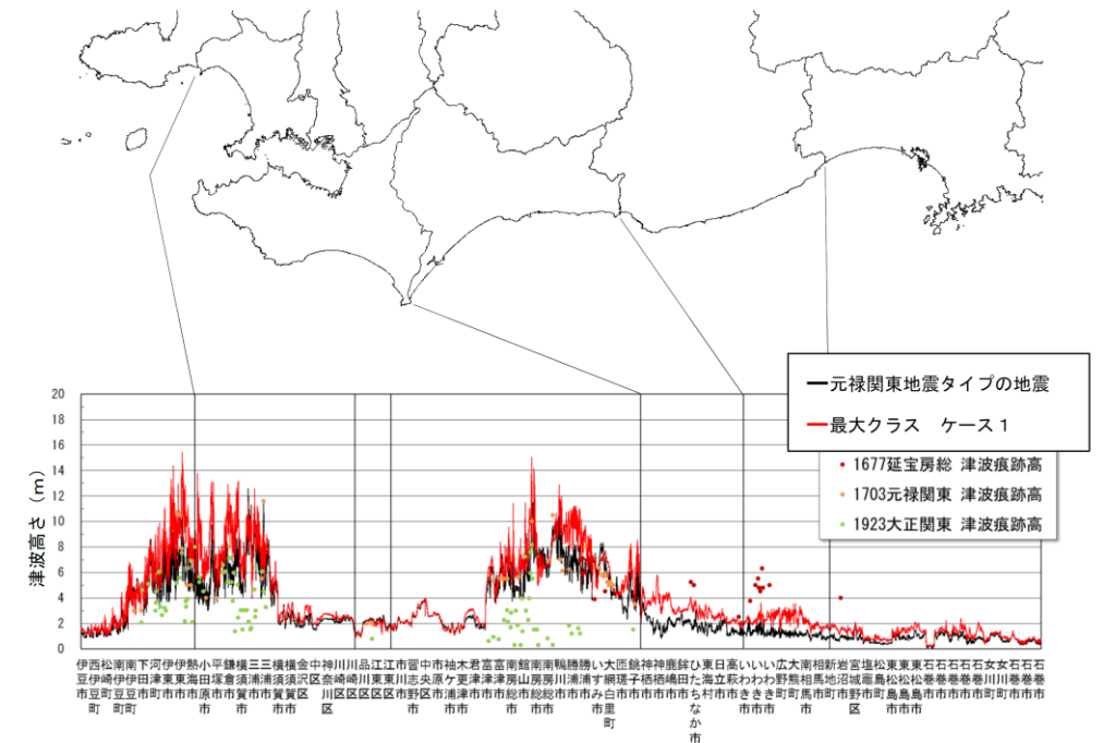
※50mメッシュ計算、津波高さには地殻変動量の沈降分を加算して表示 (内閣府(2013))
