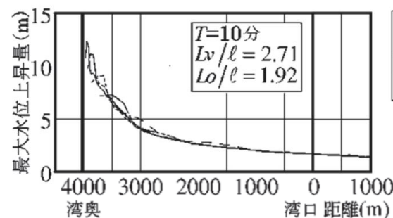
湾口～湾奥縦断沿いの最大水位上昇量分布の比較
