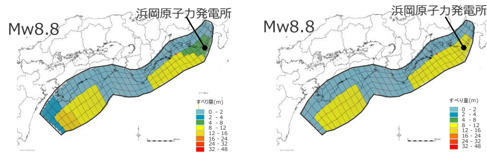
プレートの沈み込み速度を 考慮したモデル
