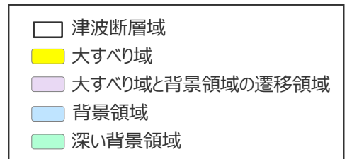
遠州灘沿岸域の痕跡再現モデル
