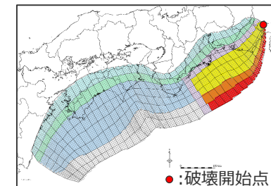
検討波源モデルAの最大ケース (破壊開始点P4)
