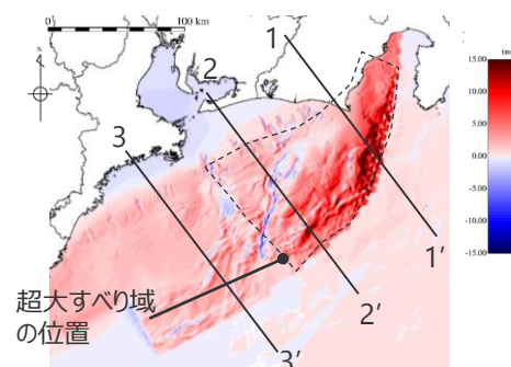
検討波源モデルDの地殻変動量分布図 および断面位置
