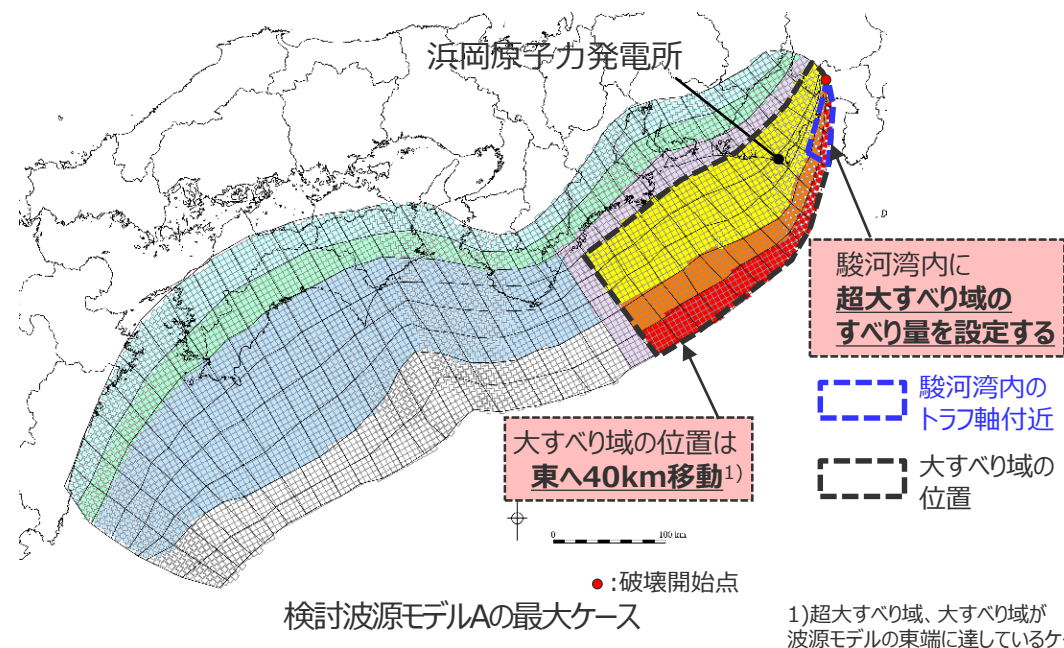
内閣府の最大クラスモデル（ケース①）と検討波源モデルAの最大ケースとの比較分析
