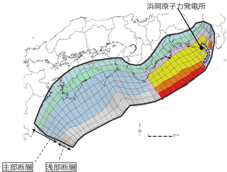
検討波源モデルB-2 (プレート境界面浅部・御前崎海脚東部の断層帯)
