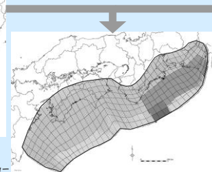
検討波源モデルB
