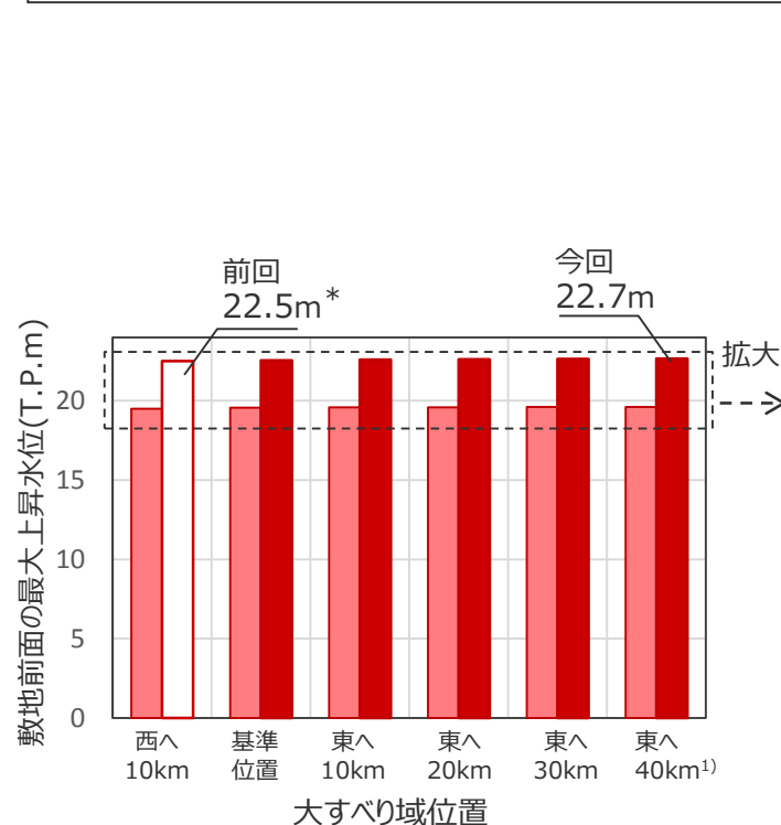
○概略パラメータスタディ結果（同時破壊を考慮）
