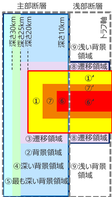
検討波源モデルDによるすべり量分布概念図
