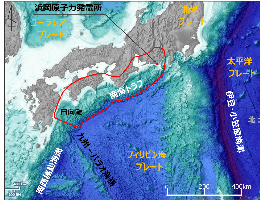
日本列島周辺の海底地形
