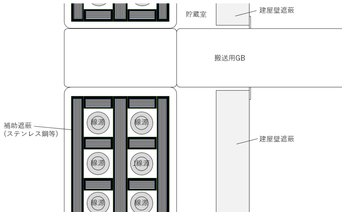
第5.-3図 機器の貫通部に対する放射線漏えい防止措置の例 (粉末一時保管室のグローブボックス貫通部の平面図)
