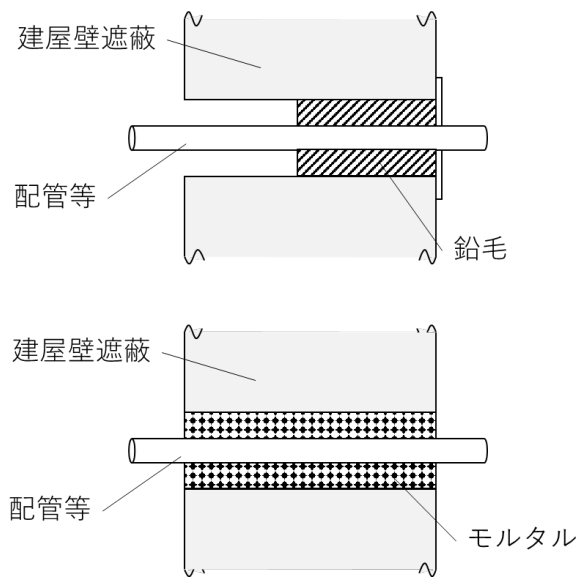
第5.-1図 配管等の貫通部と建屋遮蔽の間隙に対する放射線漏えい防止措置の例
