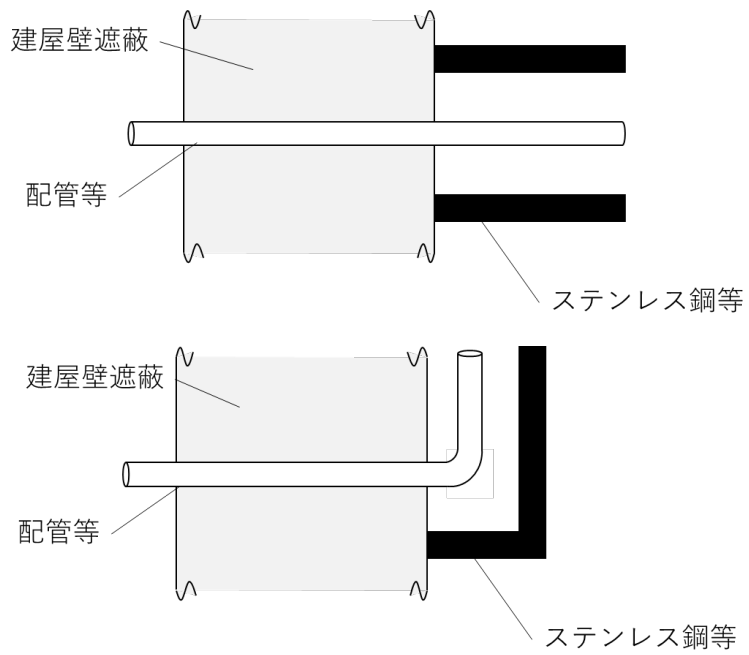
第5.-2図 配管等の貫通部に対する放射線漏えい防止措置の例
