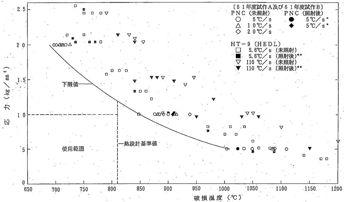
第14図 被覆管急速加熱時の破損温度
