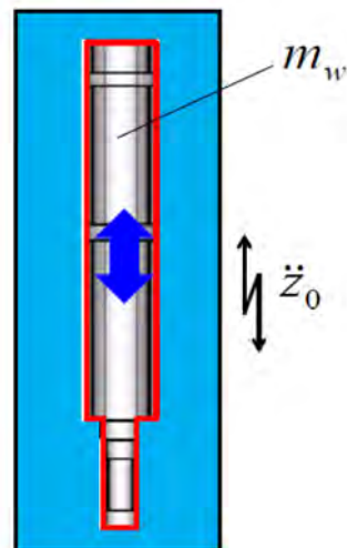
第 3 図 流体慣性力
