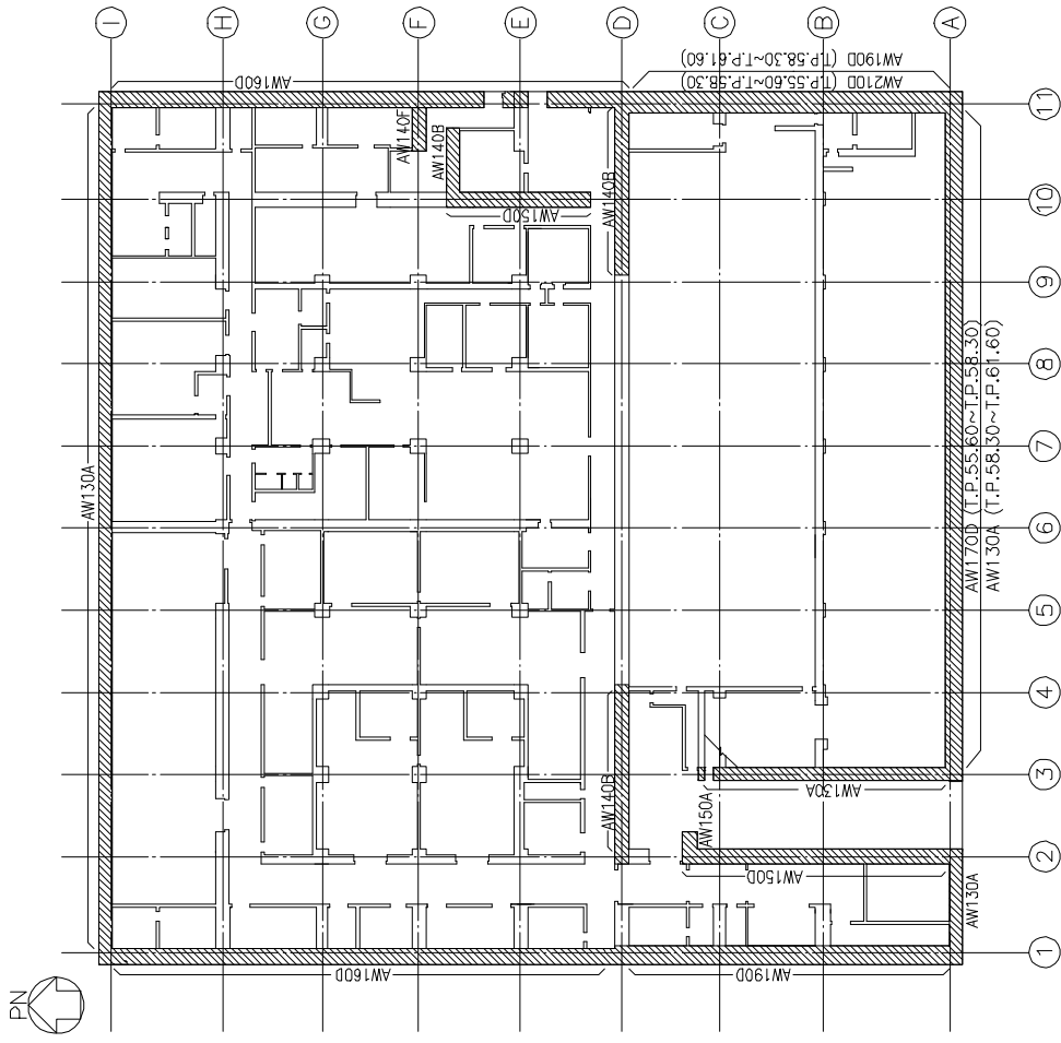
1階キープラン (T.P.55.60m)
