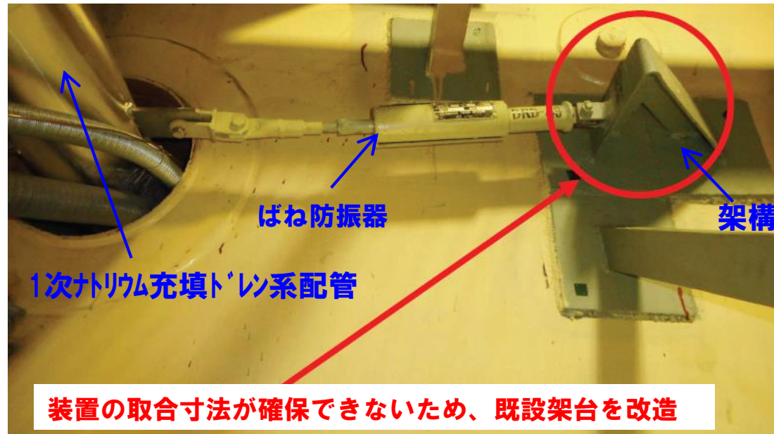
ばね防振器からメカニカル防振器への交換の例①
