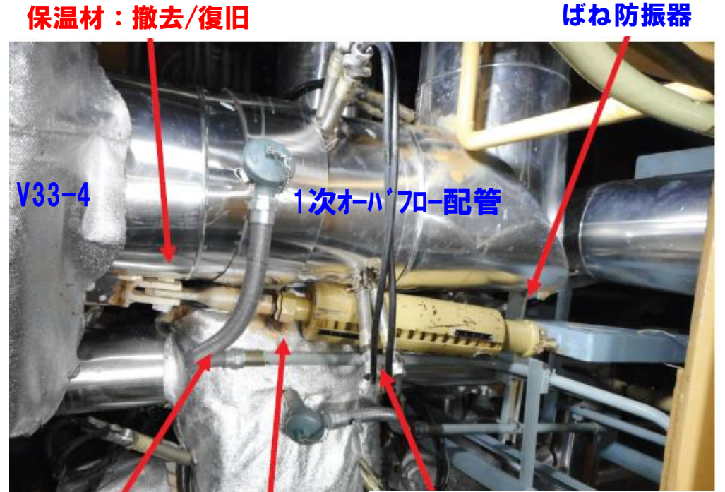
温度計：移設 保温材：改造 ヒータケーブル：移設 ばね防振器からメカニカル防振器への交換の例②
