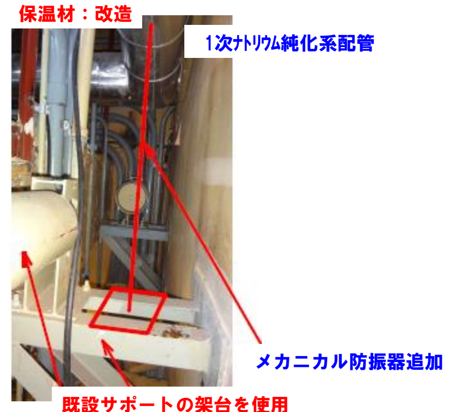
メカニカル防振器の追加の例②
