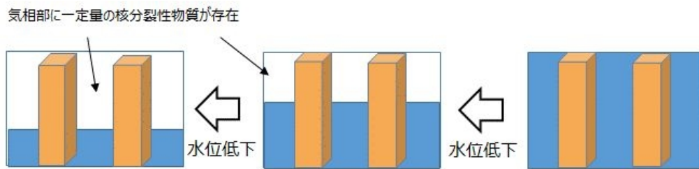
TCA 実験炉の体系概念図
