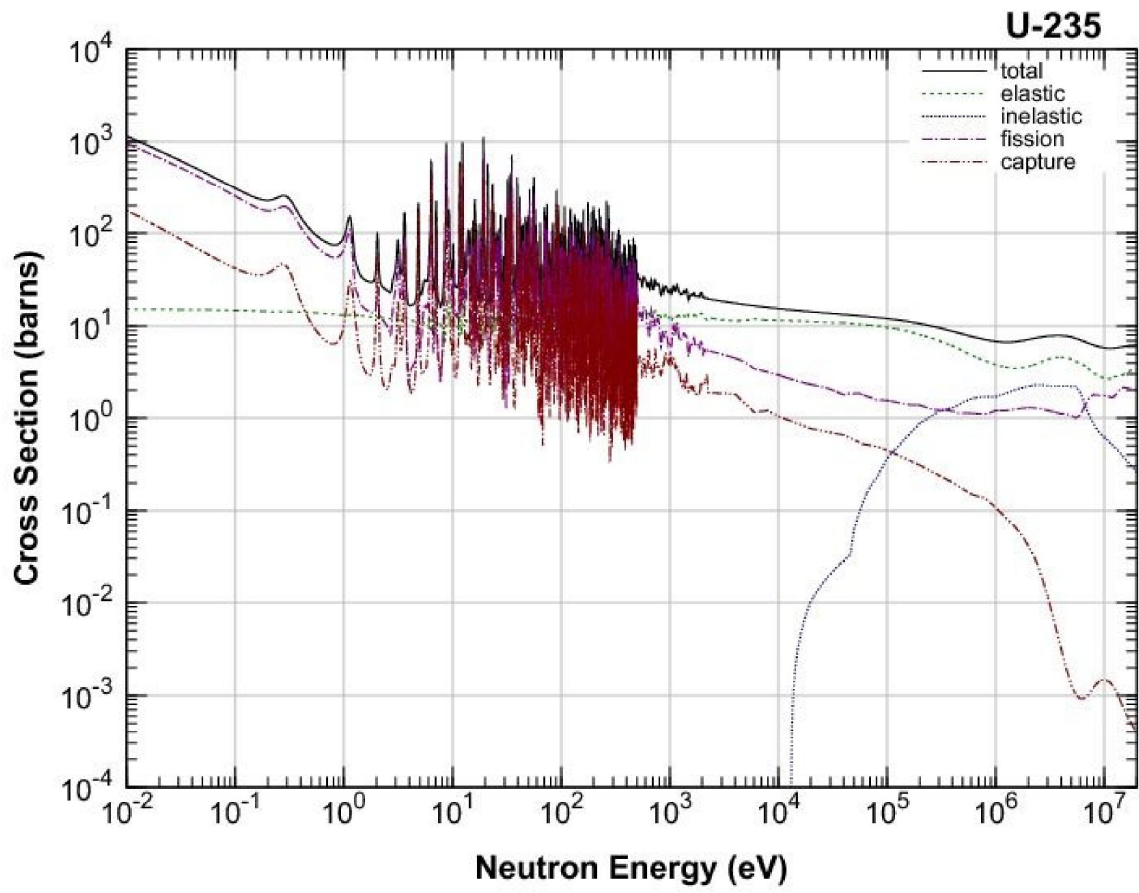
图3 ^{235}\text{U} 断面積
