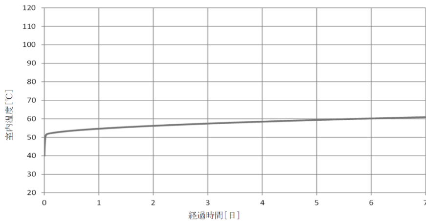
図 3-8 HPCS ポンプ室冷却機室の室温評価結果
