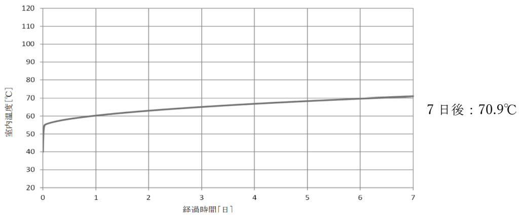
図 3-2 A-RHR ポンプ室の室温評価結果
