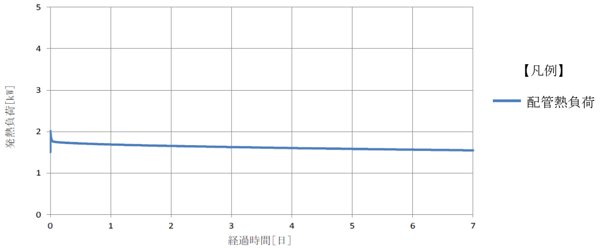
図 2-4 C-RHR ポンプ室内の熱負荷
