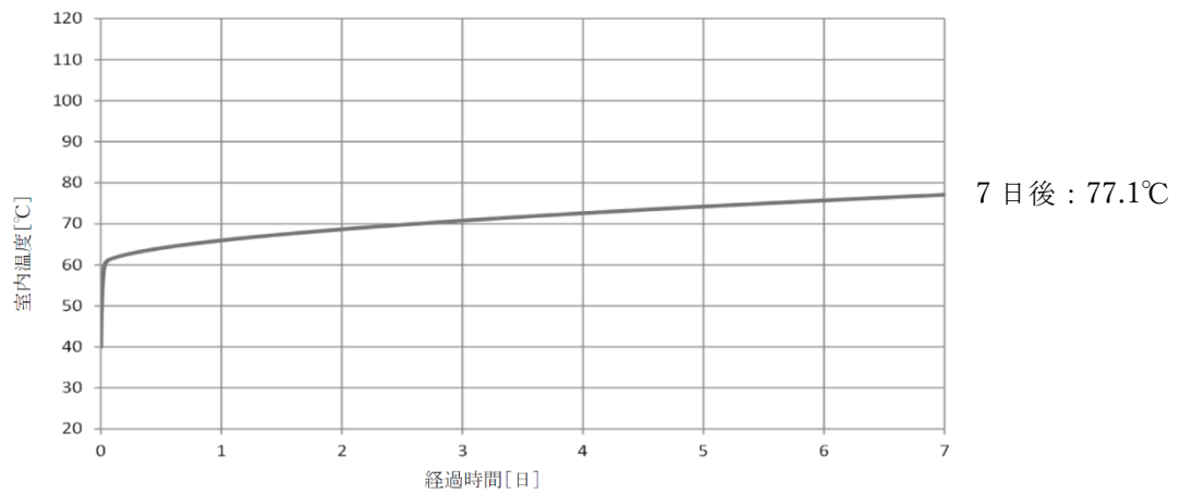
図 3-4 RCIC ポンプ室の室温評価結果
