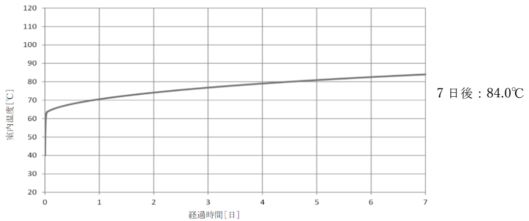
図 3-5 B-RHR ポンプ室の室温評価結果
