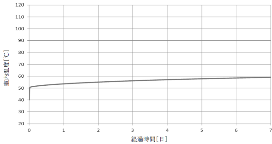
図 3-9 RHAR ポンプ室の室温評価結果
