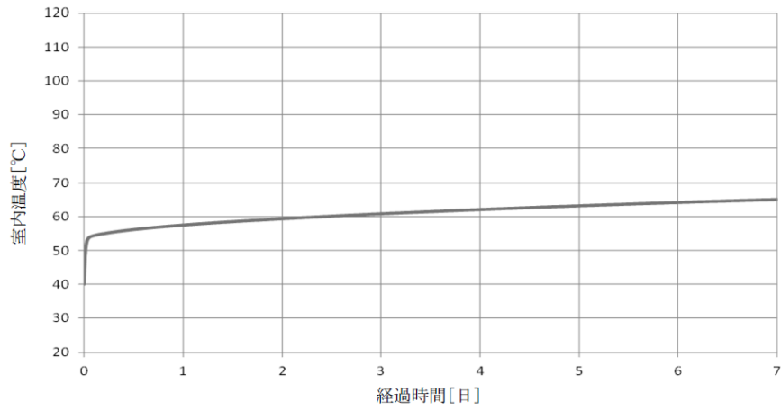
図 3-6 C-RHR ポンプ室の室温評価結果
