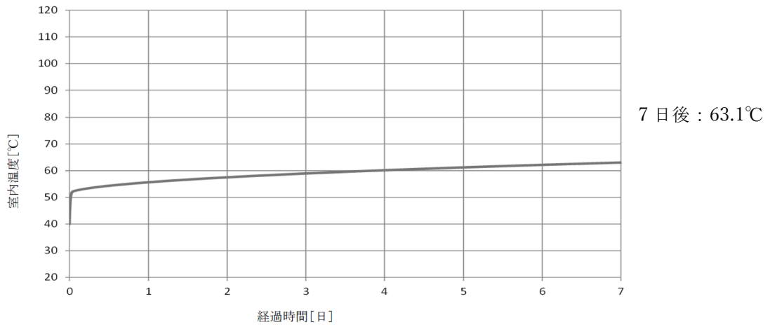
図 3-3 LPCS ポンプ室の室温評価結果
