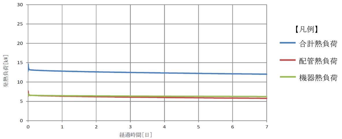
図 2-2 RCIC ポンプ室内の熱負荷
