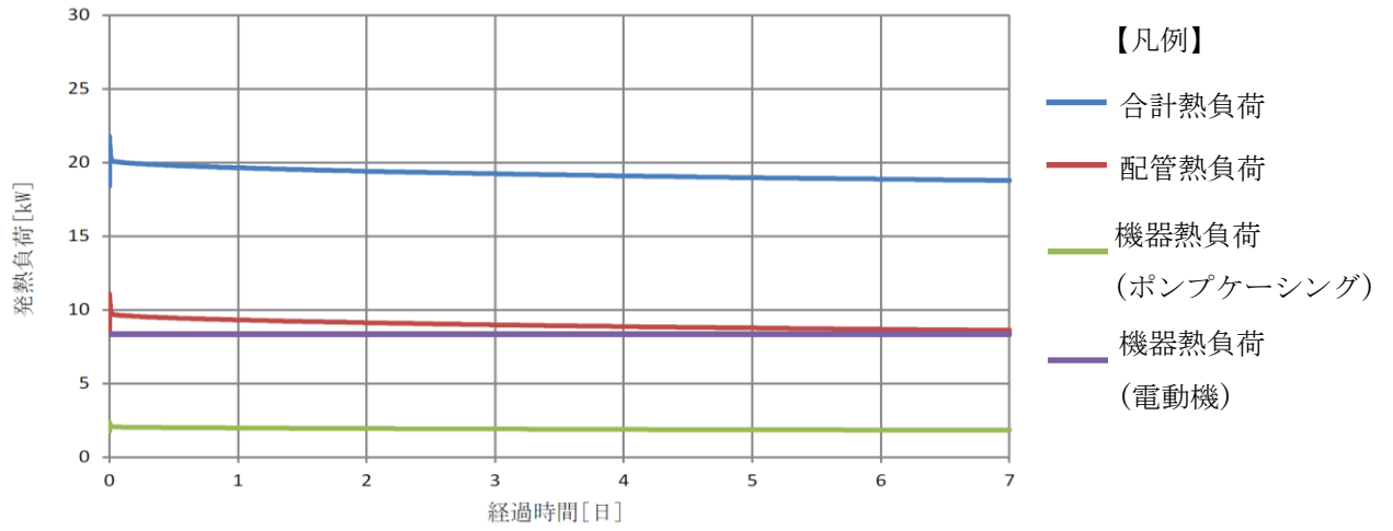
図 2-5 RHAR ポンプ室内の熱負荷
