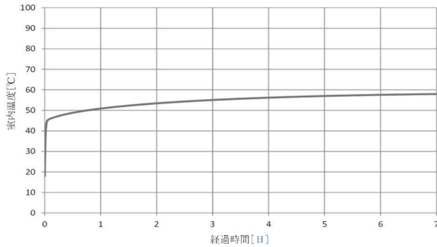
図 3-10 第 1 ベントフィルタ格納槽の室温評価結果
