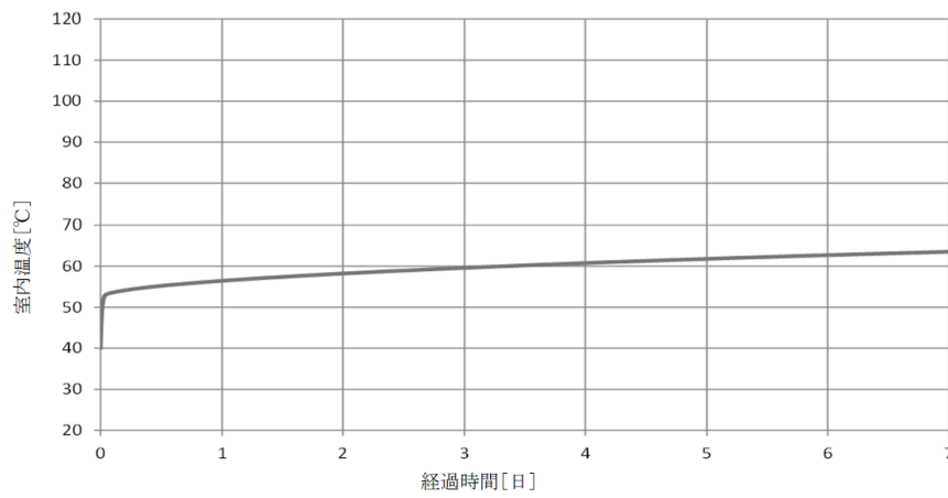
図 3-7 A-RHR ポンプ室冷却機室の室温評価結果
