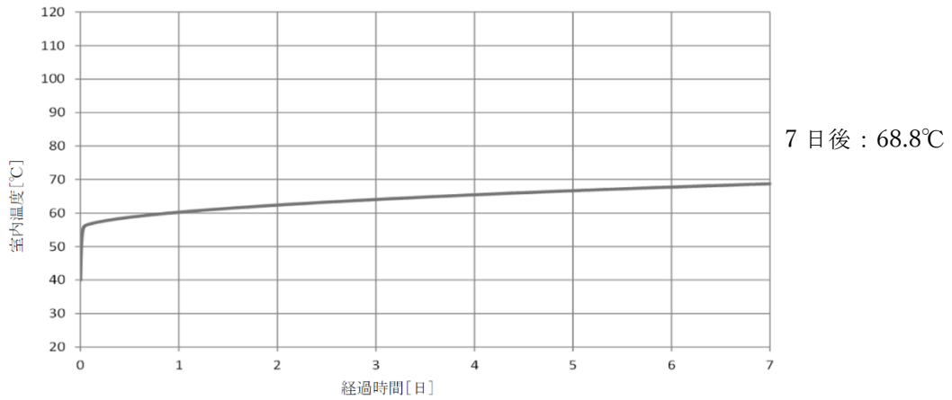
図 3-1 B-RHR ポンプ室冷却機室の室温評価結果
