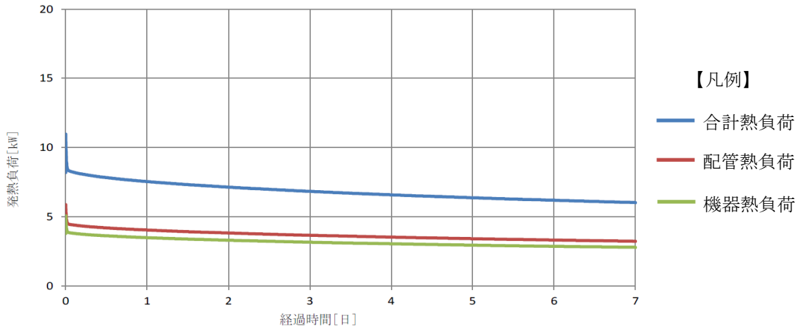
図 2-3 B-RHR ポンプ室内の熱負荷
