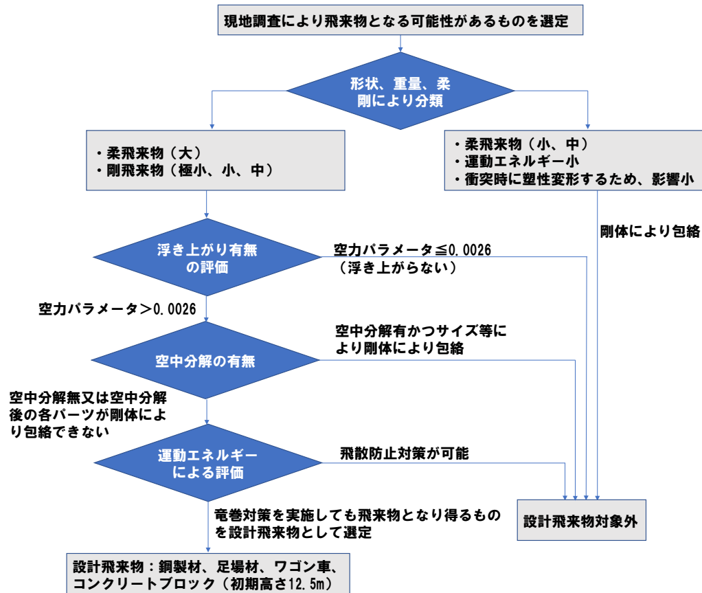
図 設計飛来物の選定フロー
