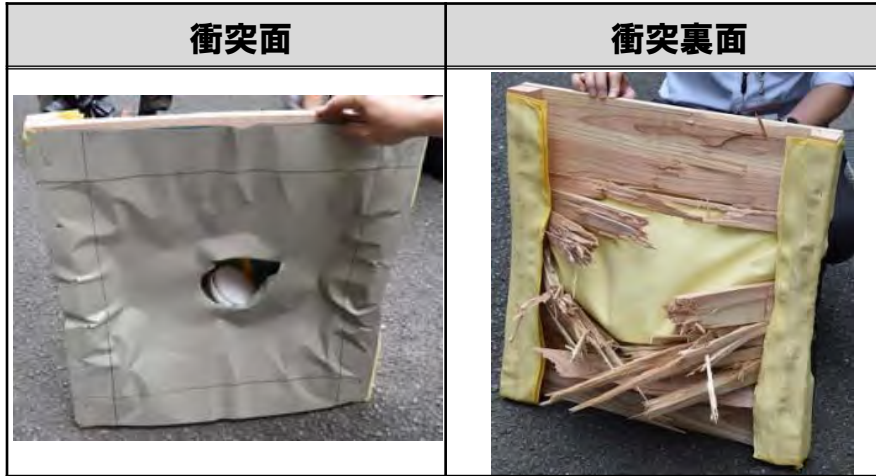
参考) 右記①～④と同構成の衝突側供試体での試験写真
