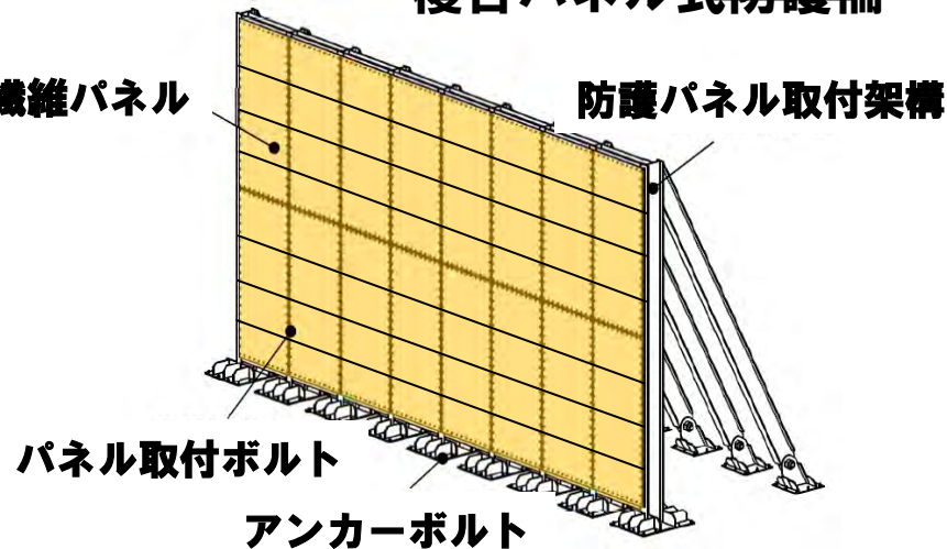
複合パネル式防護柵
