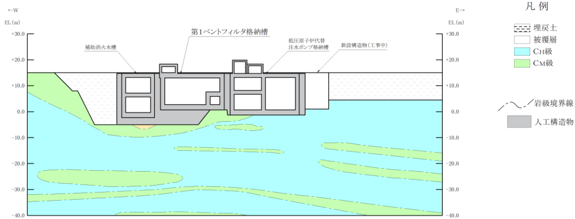
(岩級図)
