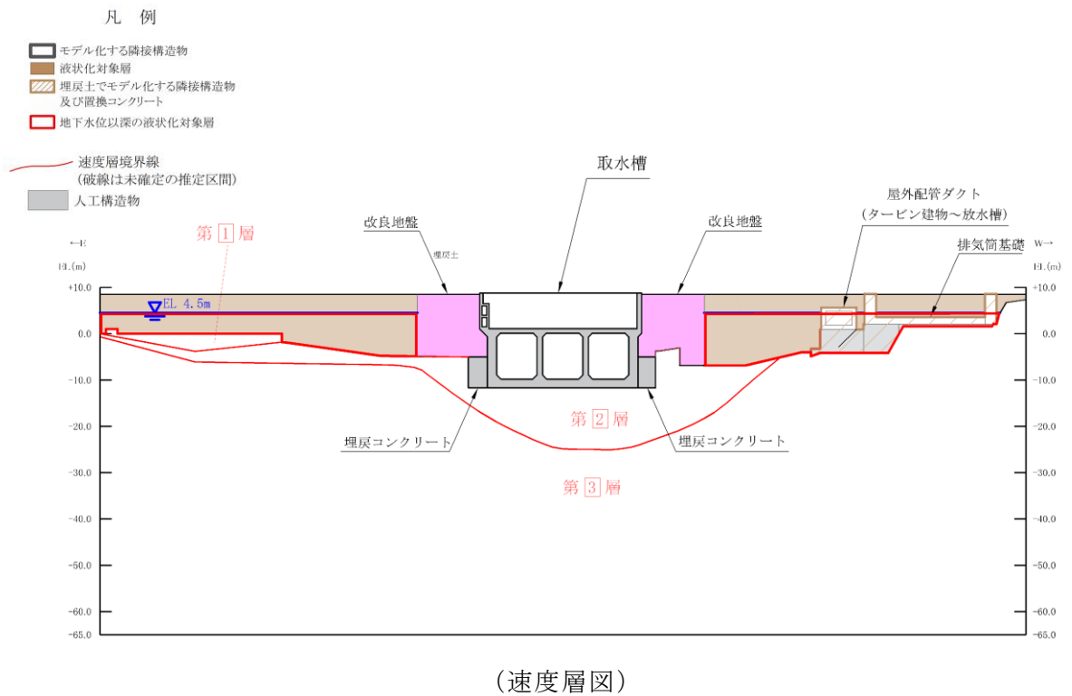
図 4.4-5 (2) 取水槽 地質断面図 (B-B 断面)
