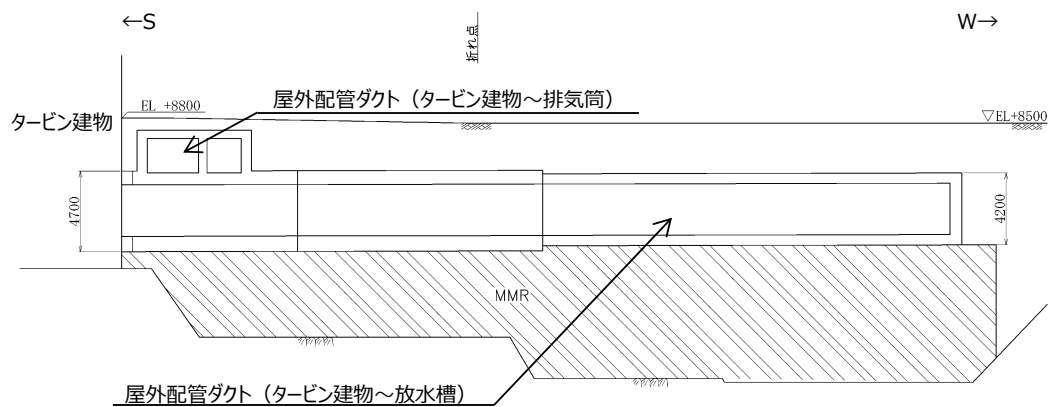
図 4.8-3 (3) 屋外配管ダクト (タービン建物～放水槽) 断面図 (D-D 断面)
