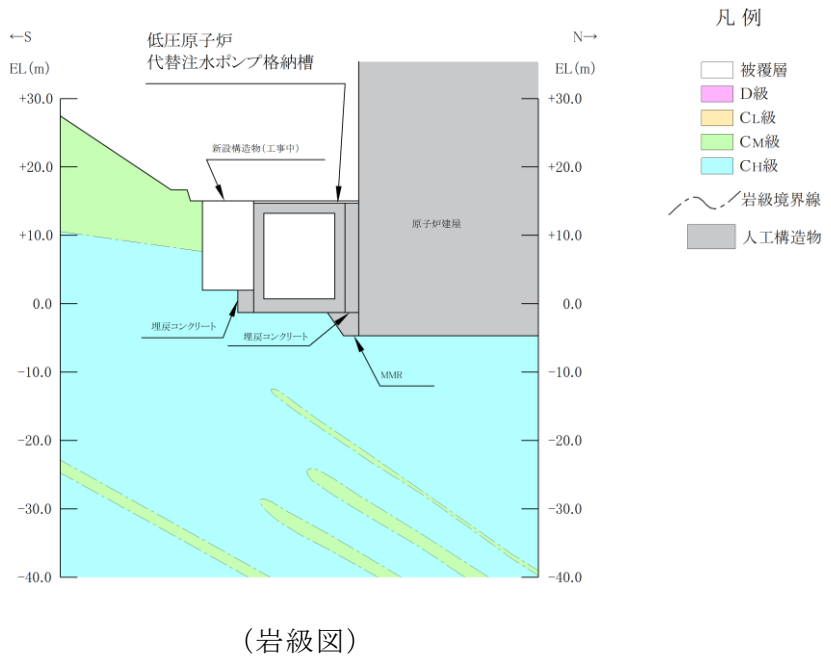
図 4.12-4 (1) 低圧原子炉代替注水ポンプ格納槽 地質断面図 (A-A断面)
