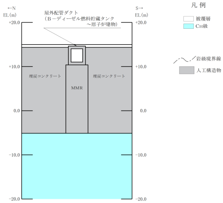
(岩級図)
