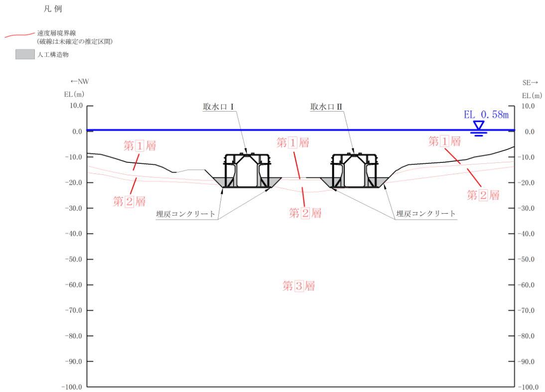
図 4.3-2(6) 取水口 地質断面図 (②全応力解析)
