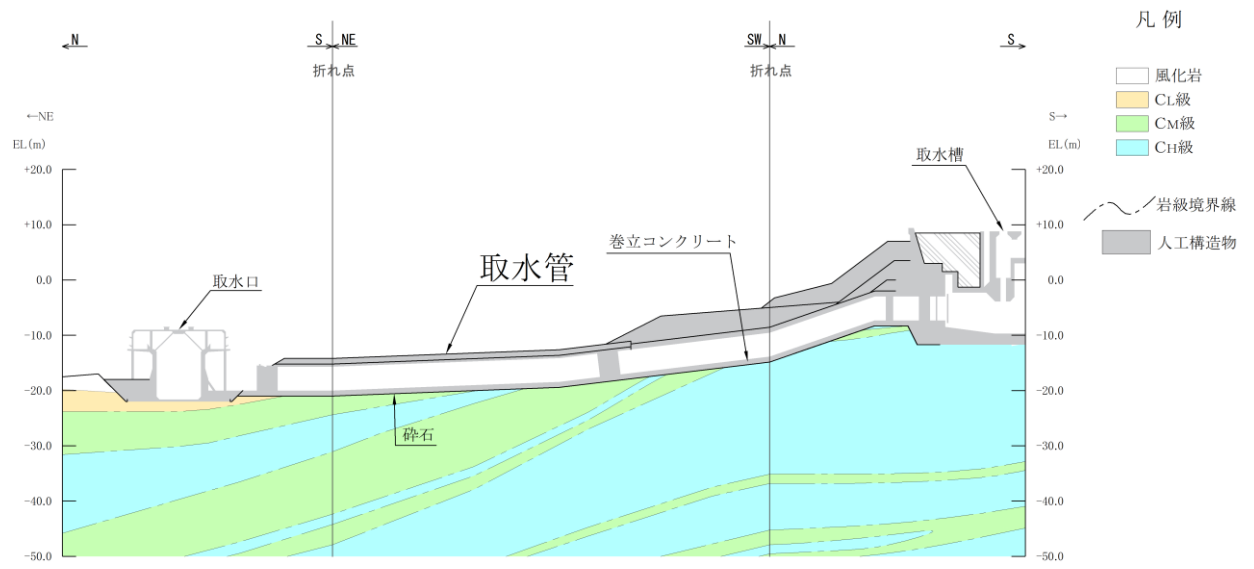
(岩級図)
