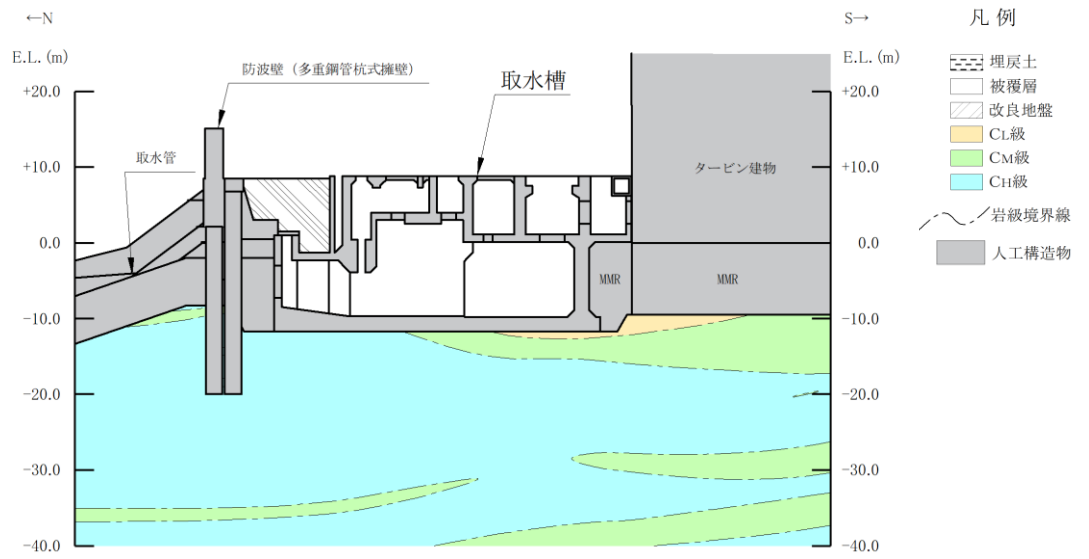
(岩級図)
