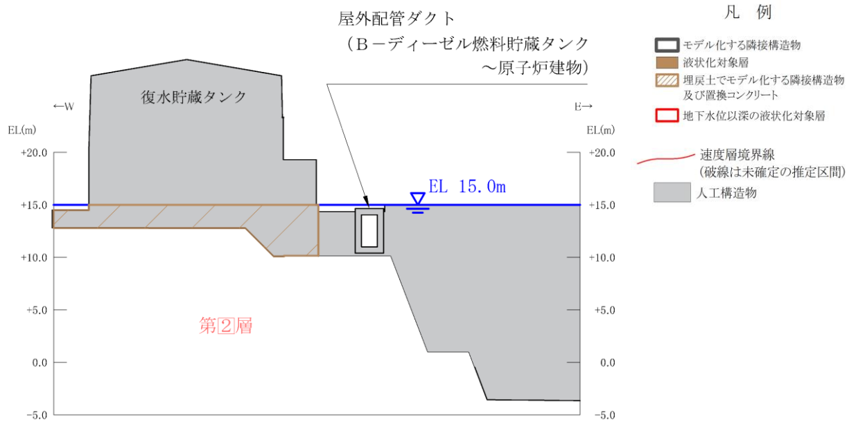
図 4.3-2(9) 屋外配管ダクト (B-ディーゼル燃料貯蔵タンク～原子炉建物) 地質断面図【A-A断面】 (②全応力解析)
