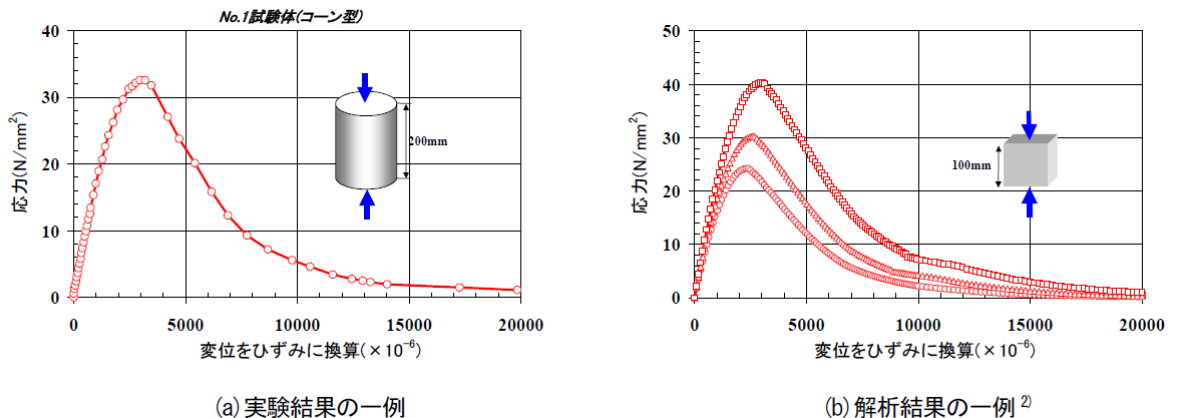
図6.3-3 コンクリートの圧縮ひずみが1.0% (10000 \mu ) 時点における残留応力 (土木学会マニュアル2005より引用)
