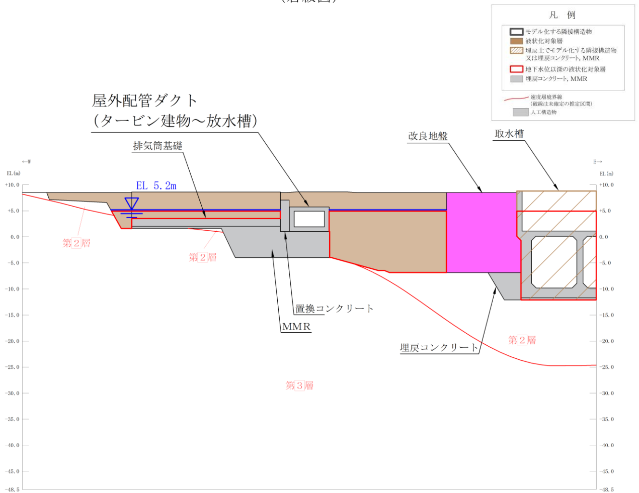
(速度層図)
