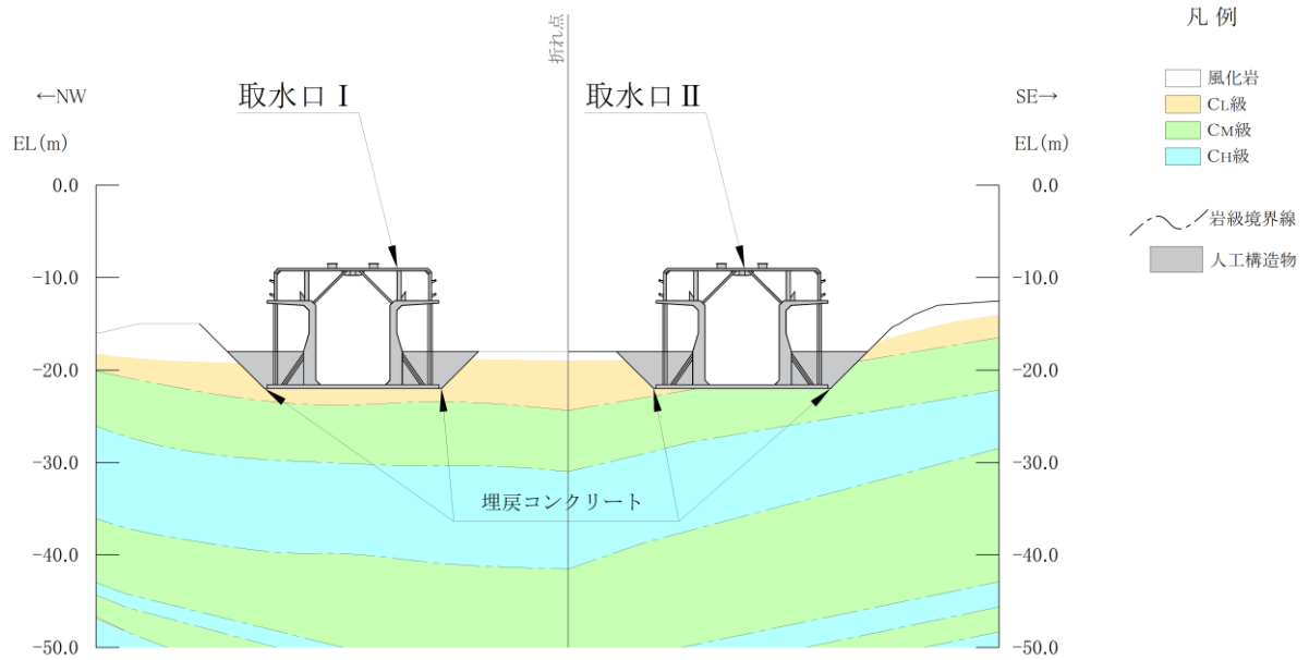
(岩級図)
