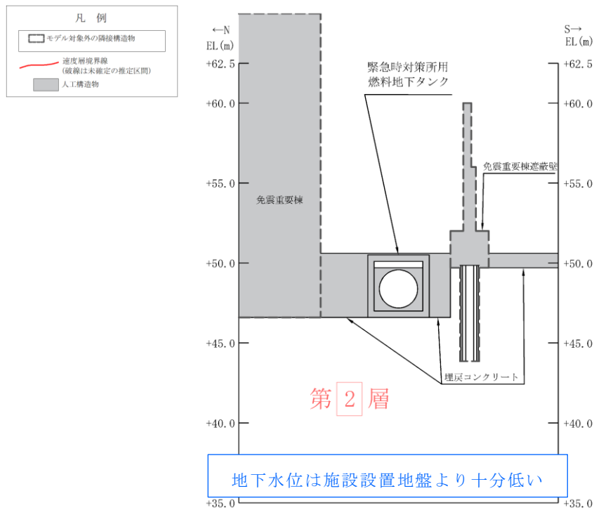
図 4.3-2(2) 緊急時対策所用燃料地下タンク 地質断面図
