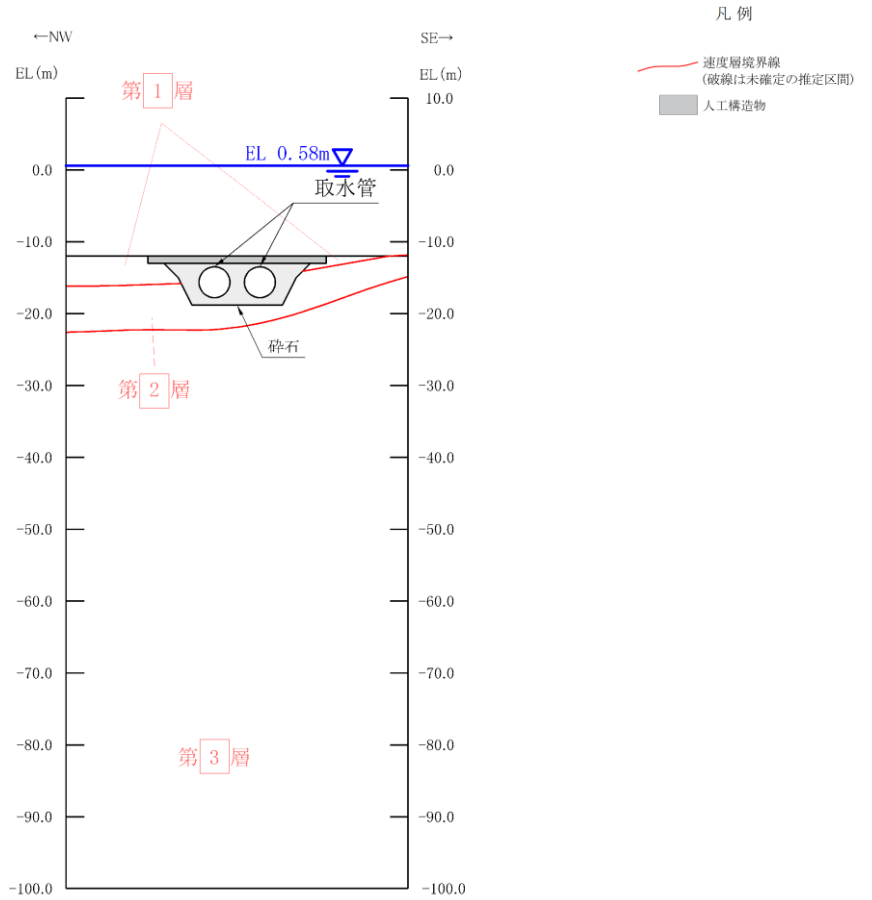
図 4.3-2(7) 取水管 地質断面図 (②全応力解析)
