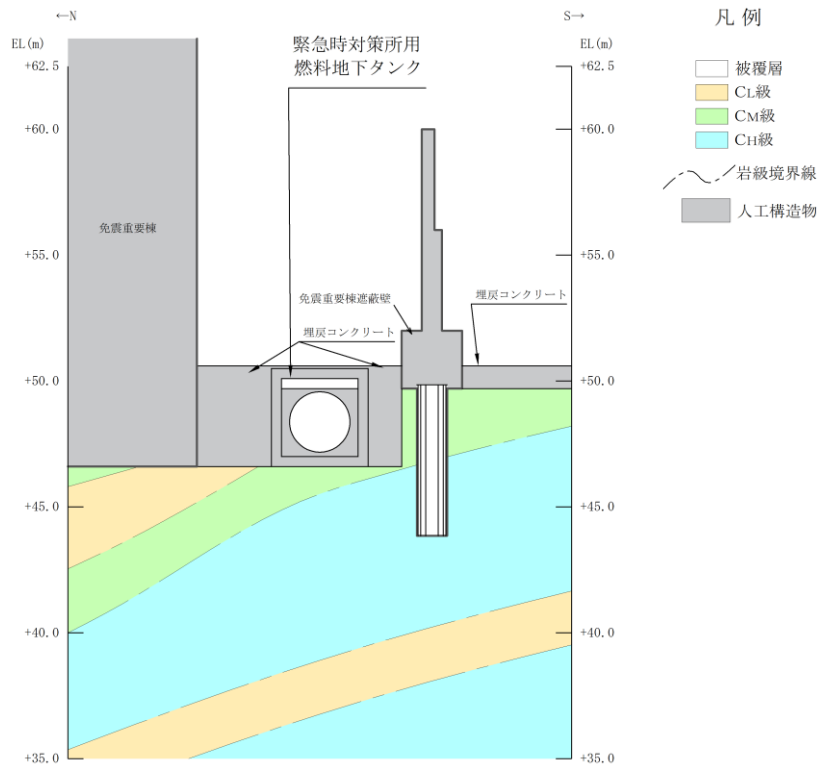
(岩級図)
