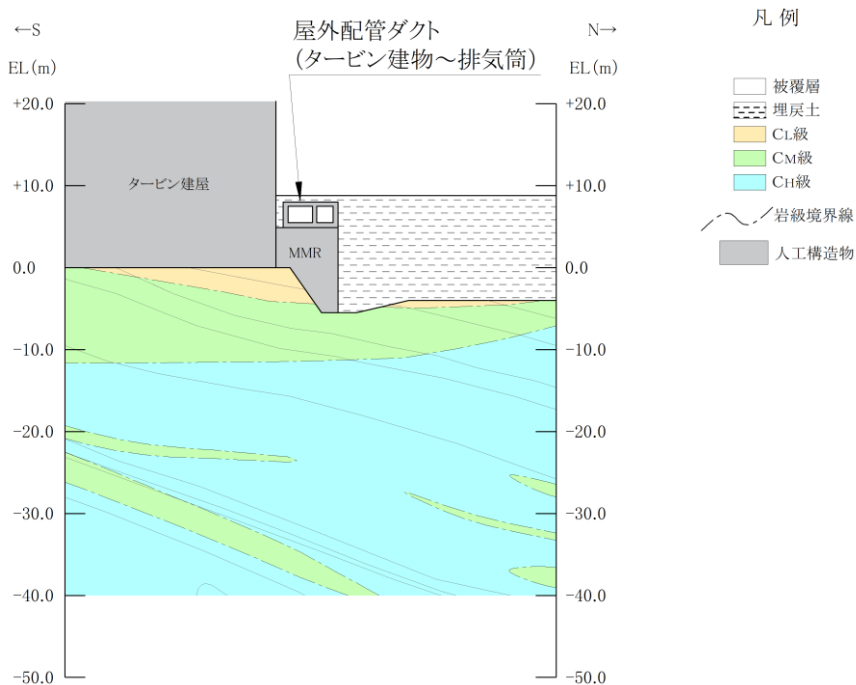
(岩級図)
