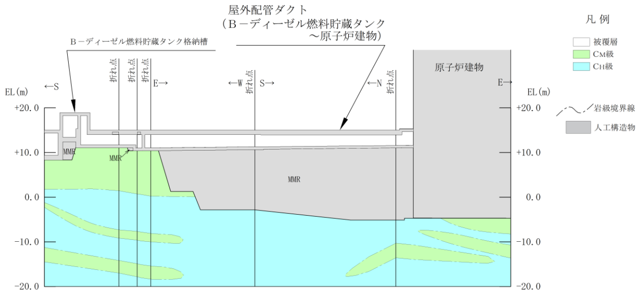
(岩級図)
