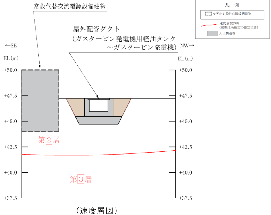
図 4.15-4 (1) 屋外配管ダクト
