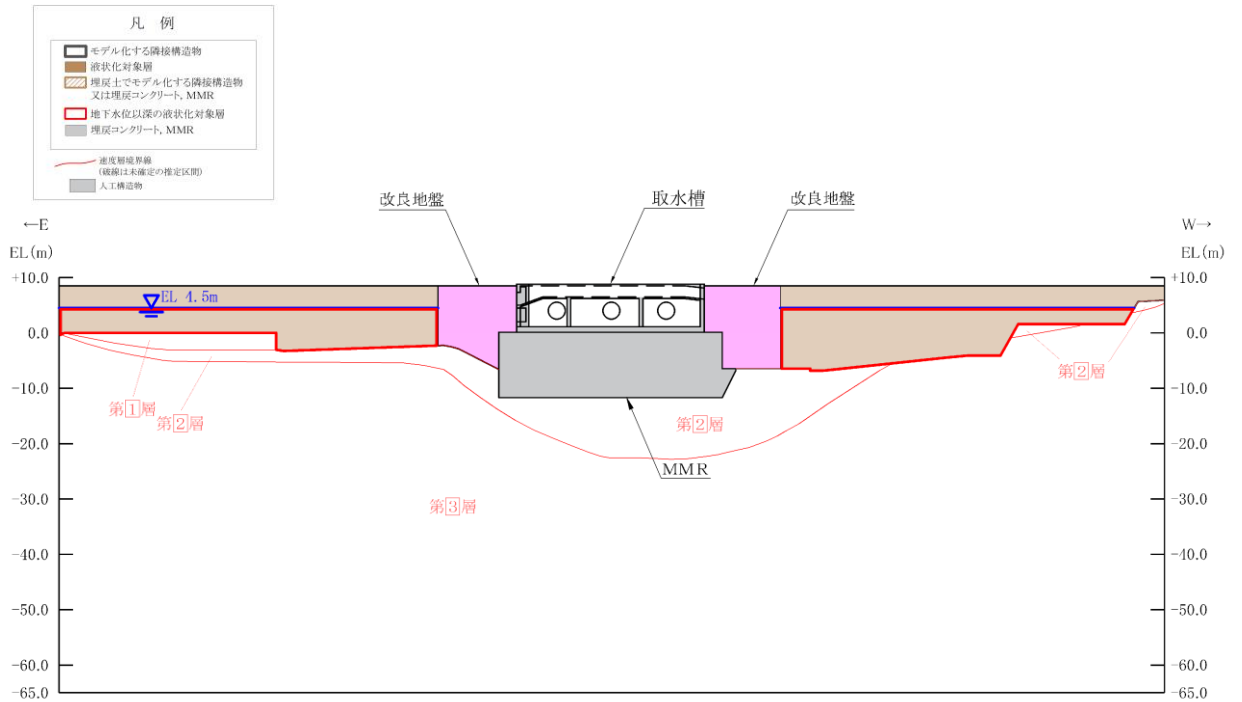
図 4.3-2(16) 取水槽【C-C断面】 地質断面図 (⑤有効応力解析)
