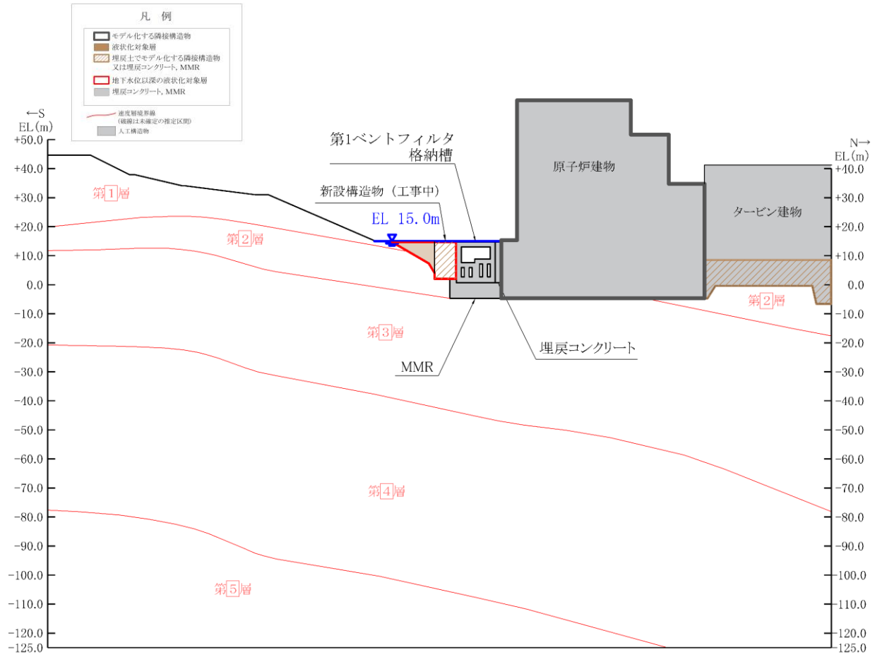
図 4.3-2(19) 第1ベントフィルタ格納槽 地質断面図
