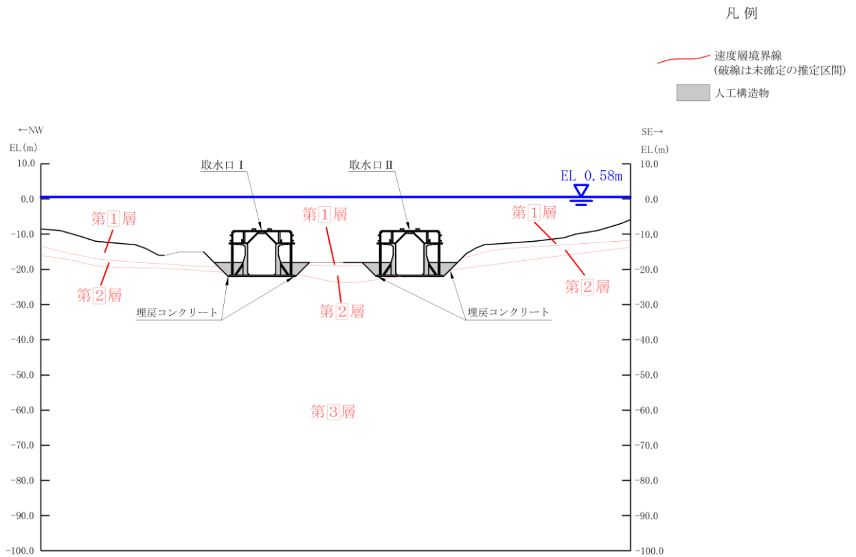
(速度層図)
