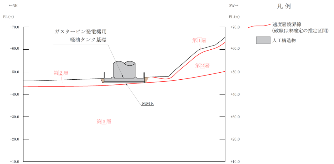
(速度層図)
