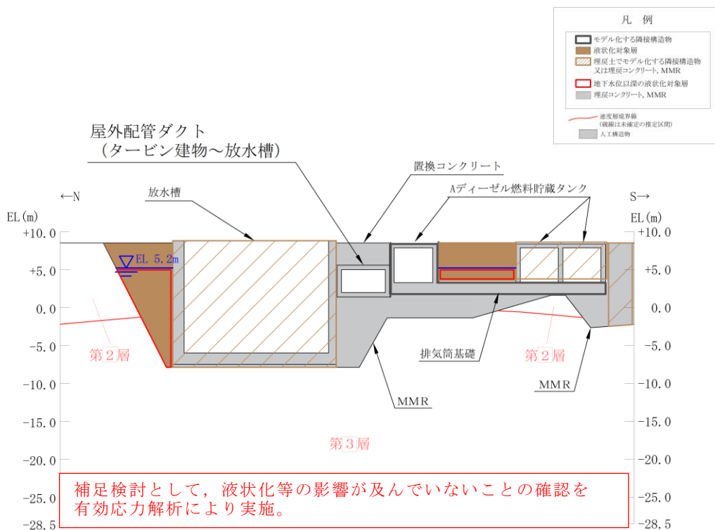
図 4.3-2(11) 屋外配管ダクト (タービン建物～放水槽)
