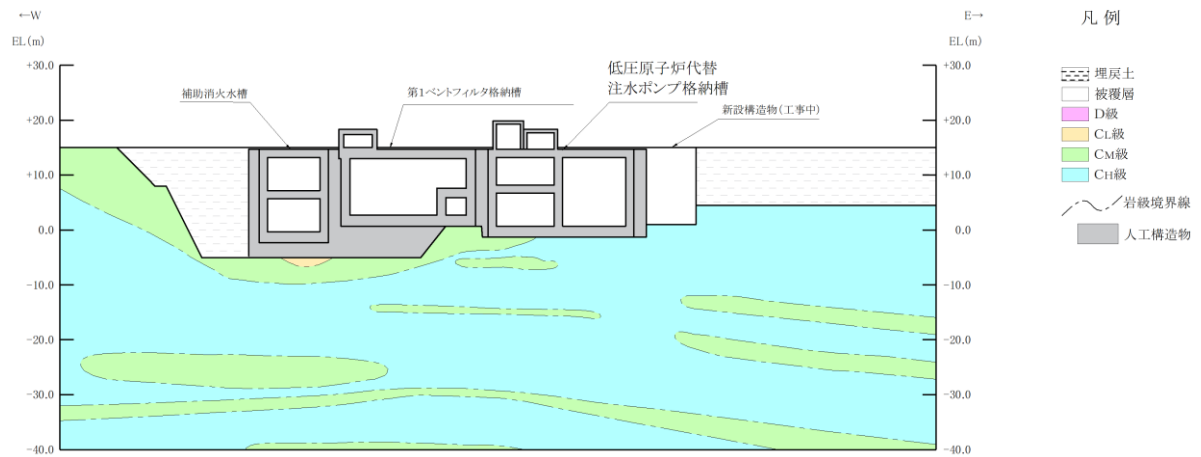
(岩級図)
