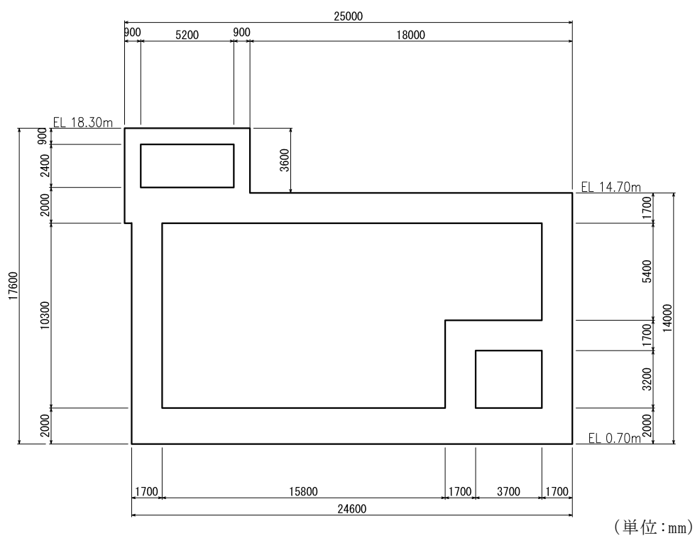
図 4.11-3 (3) 第1ベントフィルタ格納槽 断面図 (C-C断面)
