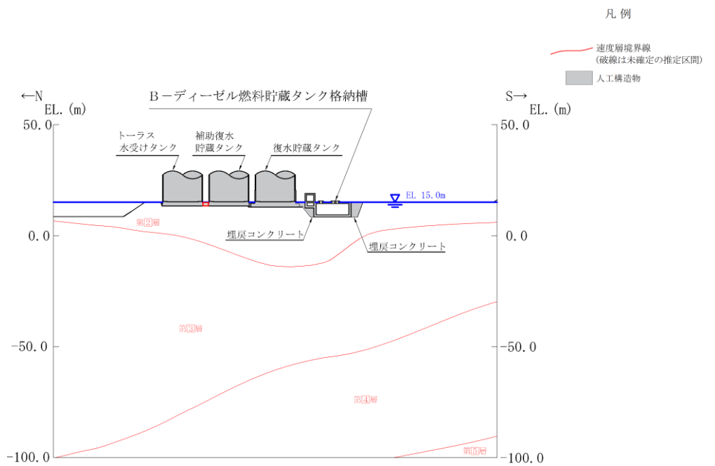
図 4.3-2(8) B-ディーゼル燃料貯蔵タンク格納槽 地質断面図【B-B断面】
