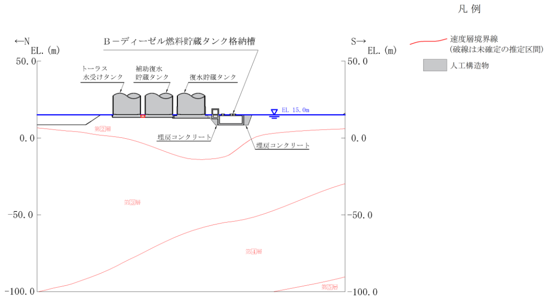
(速度層図)
