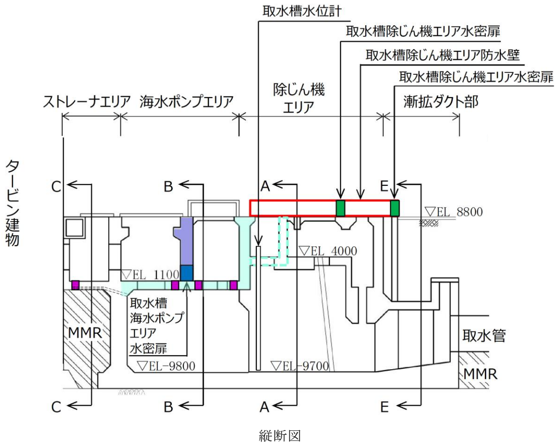
図 4.4-6 取水槽のうち止水機能が要求される範囲
