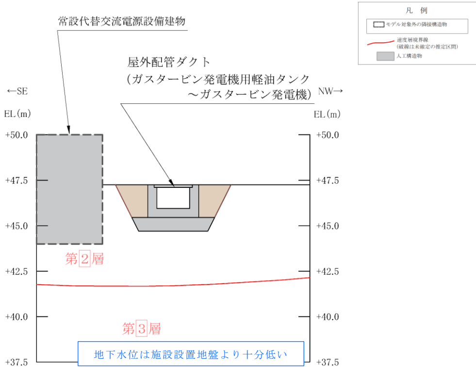
図 4.3-2(3) 屋外配管ダクト (ガスタービン発電機用軽油タンク~ガスタービン発電機) 地質断面図 (①全応力解析)
