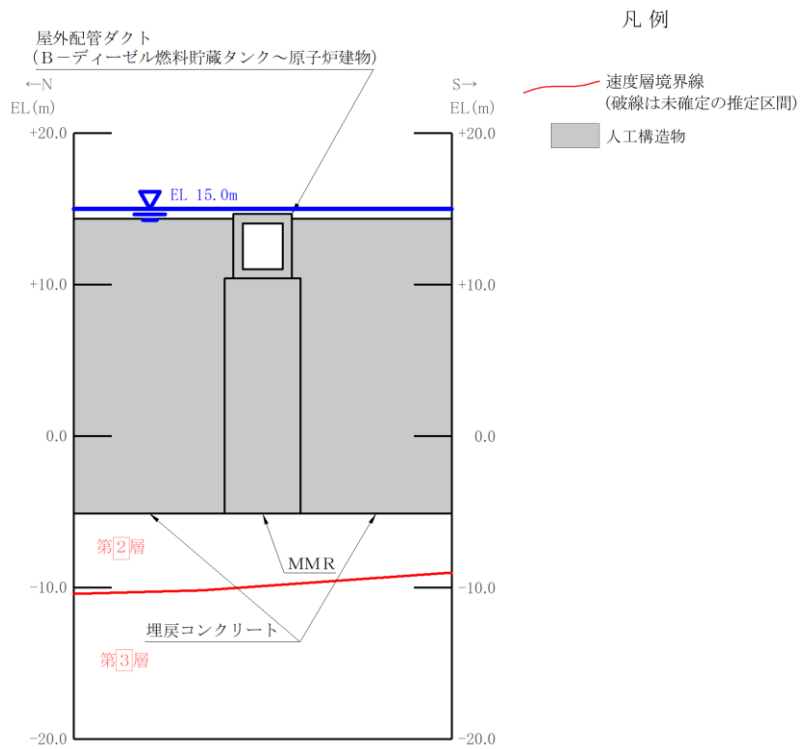
(速度層図)
