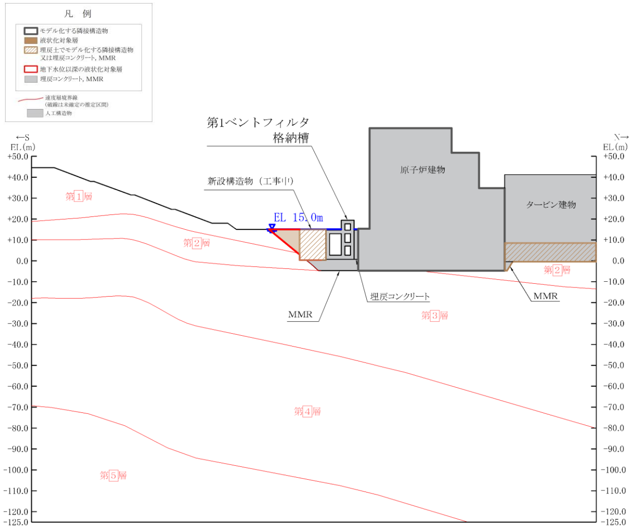
(速度層図)
