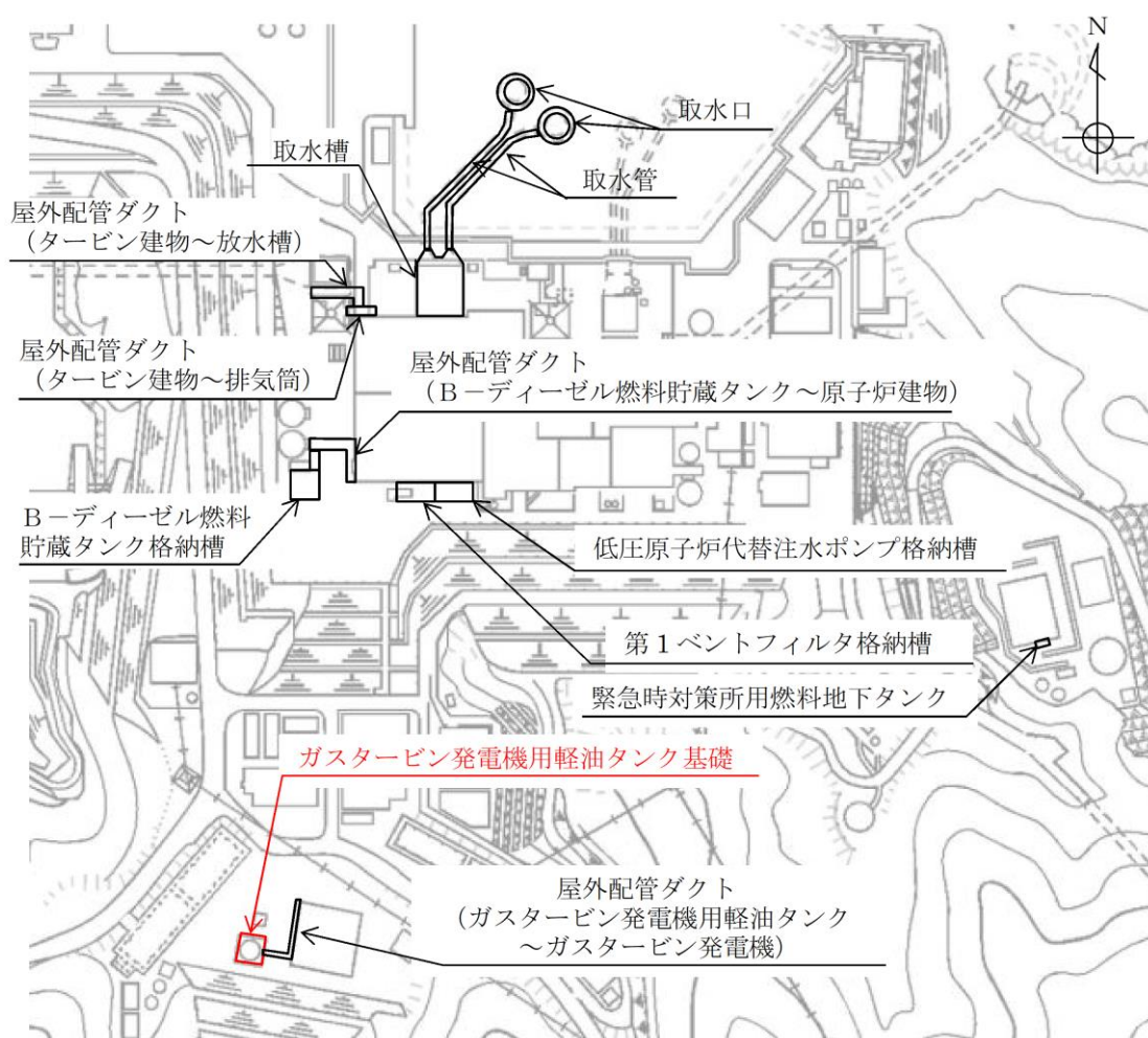
図 4.14-1 ガスタービン発電機用軽油タンク基礎 位置図
