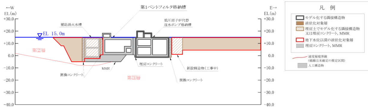
(速度層図)
