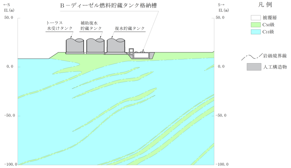
(岩級図)
