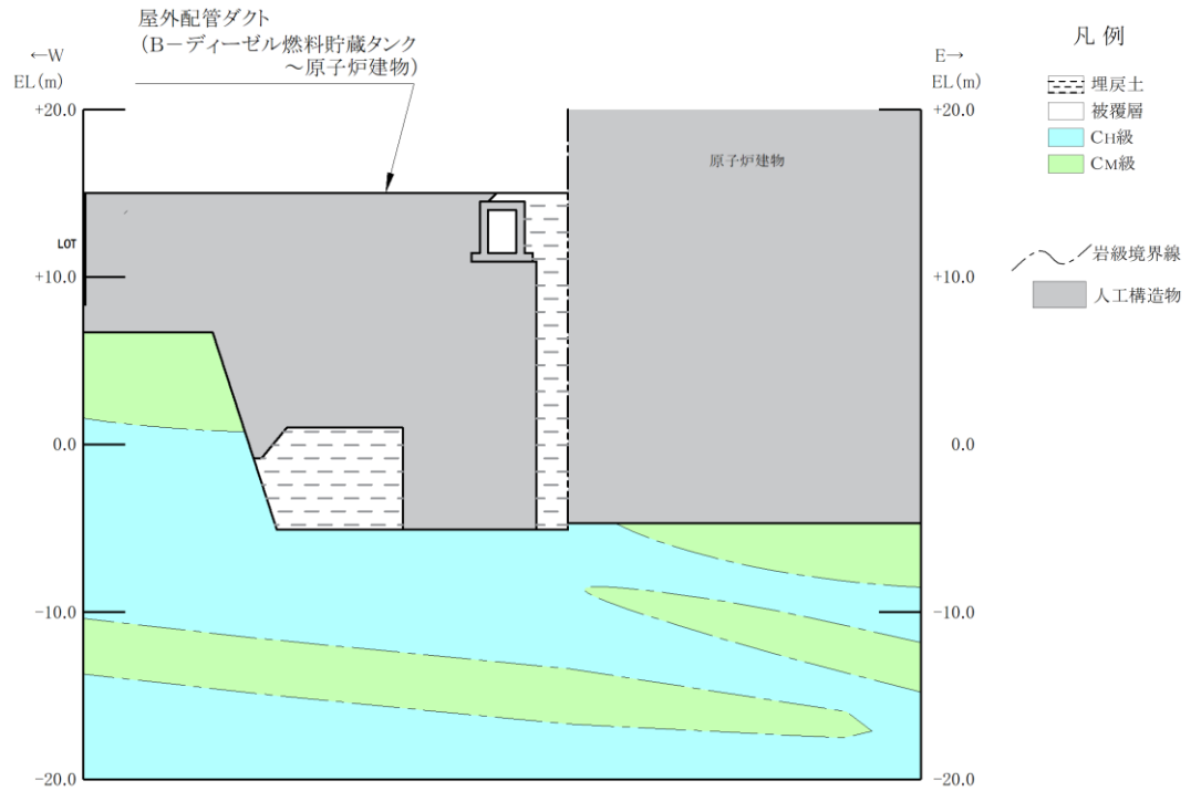
(岩級図)
