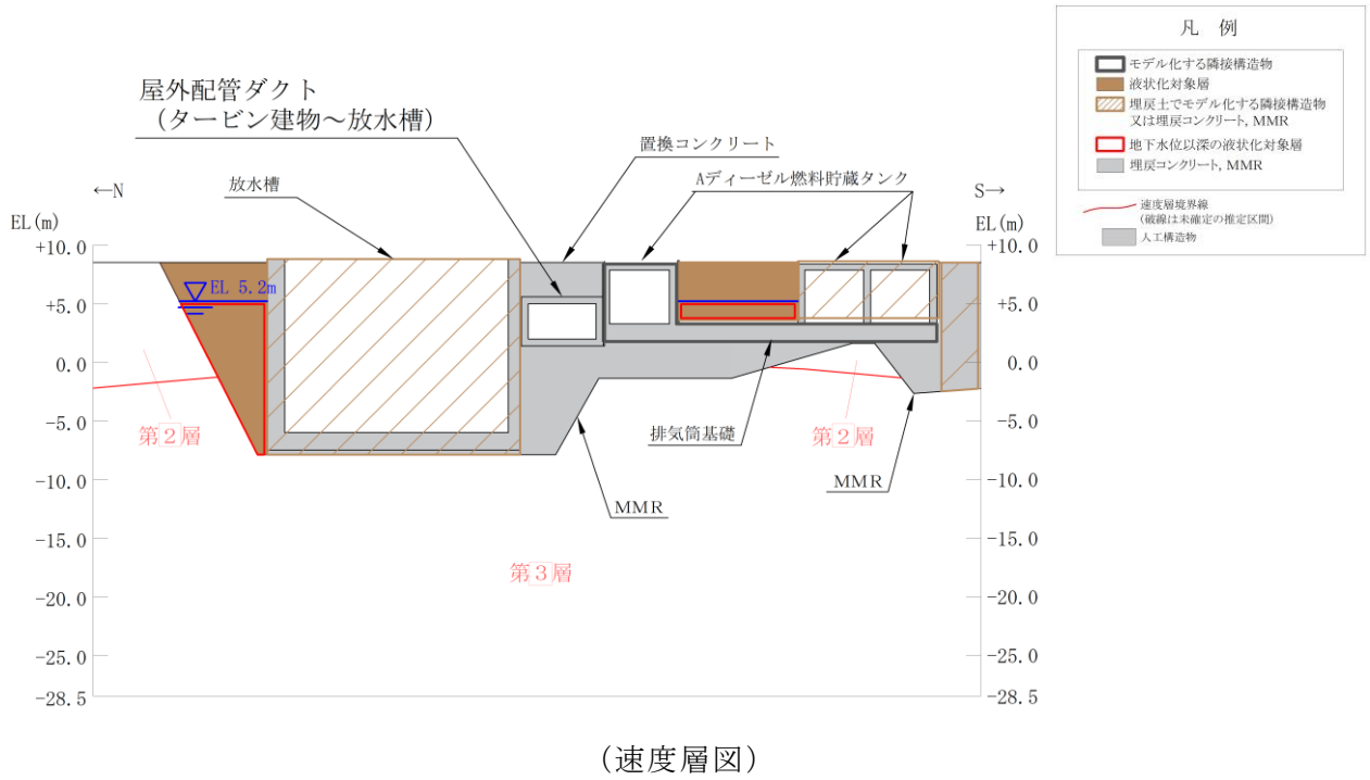
図 4.8—4 (1) 屋外配管ダクト (タービン建物～放水槽) 地質断面図 (A-A 断面)
