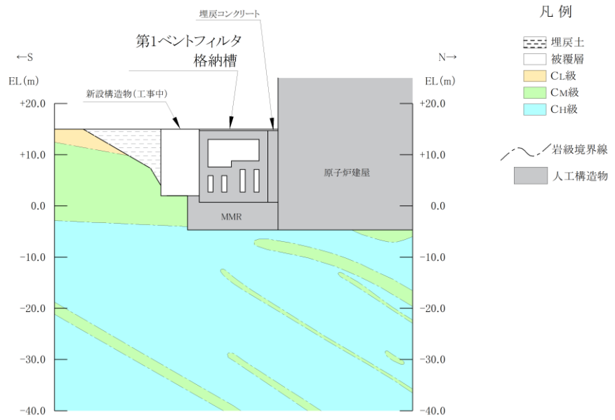
(岩級図)
