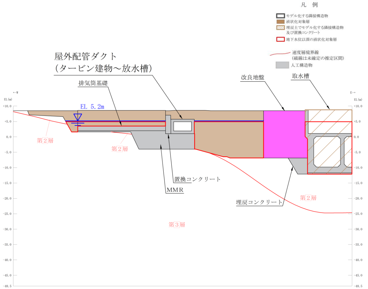
図 4.3-2(18) 屋外配管ダクト (タービン建物～放水槽) 地質断面図【C-C断面】 (⑤有効応力解析)
