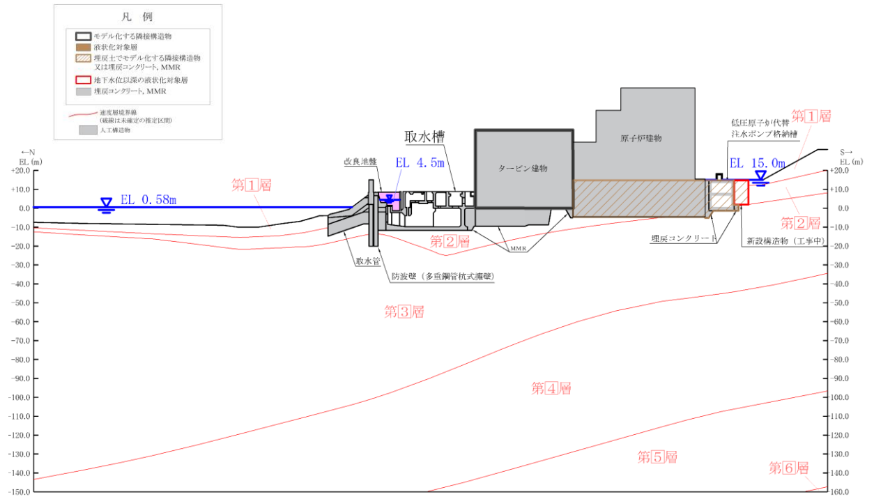
図 4.3-2(5) 取水槽【D-D断面】 地質断面図 (②全応力解析)
