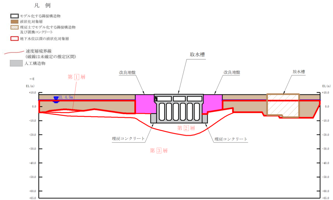
図 4.4-5 (1) 取水槽 地質断面図 (A-A断面)
