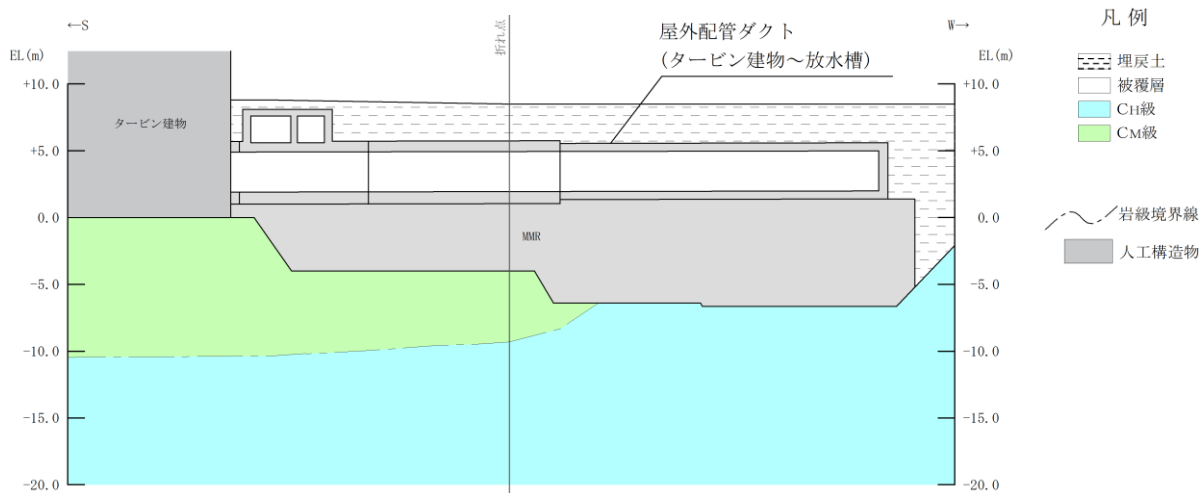
(岩級図)
