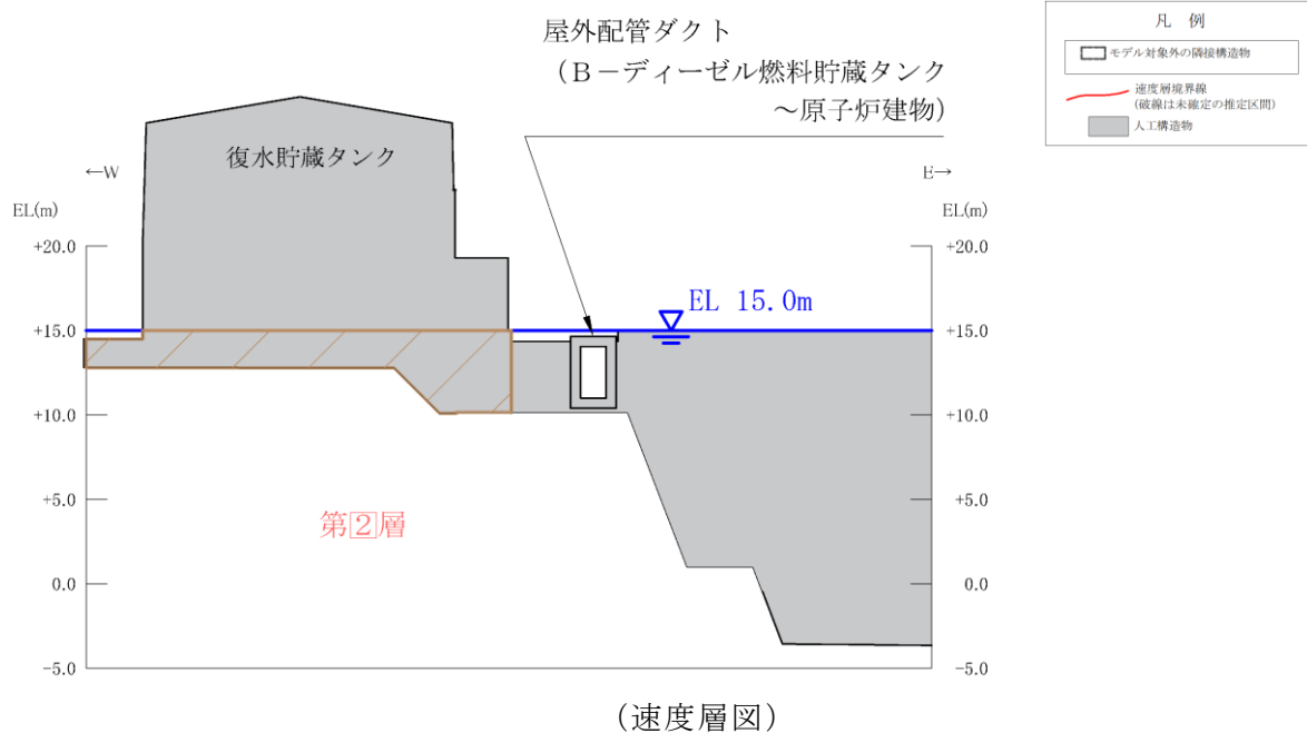
図 4.7-4 (1) 屋外配管ダクト (B-ディーゼル燃料貯蔵タンク～原子炉建物) 地質断面図 (A-A 断面)
