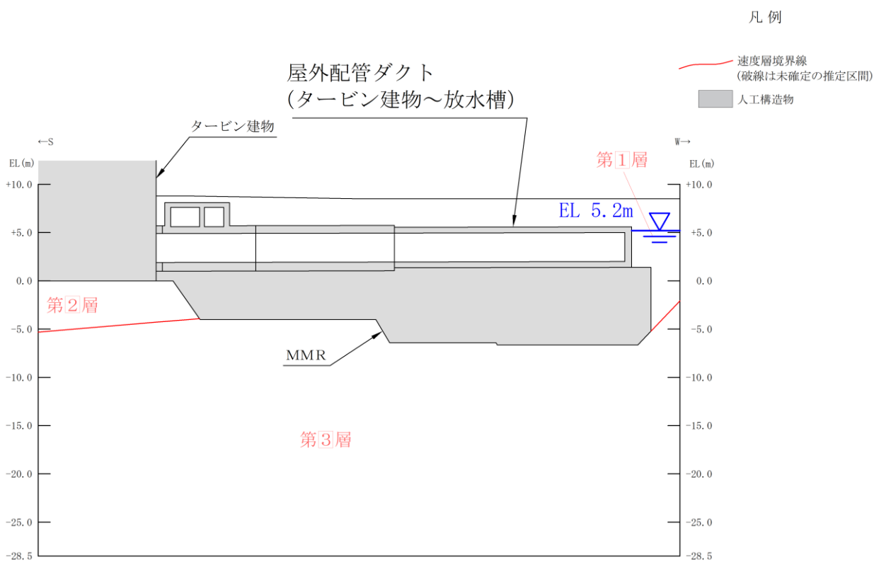
(速度層図)
