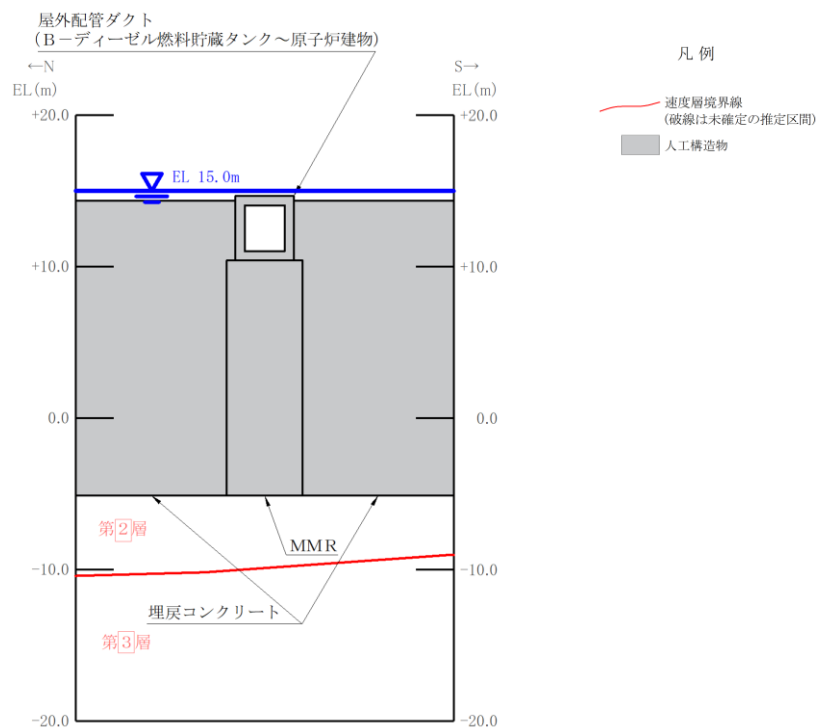
図 4.3-2(10) 屋外配管ダクト (B-ディーゼル燃料貯蔵タンク～原子炉建物) 地質断面図【B-B断面】 (②全応力解析)
