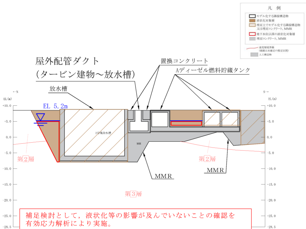
図 4.3-2(12) 屋外配管ダクト (タービン建物～放水槽)
