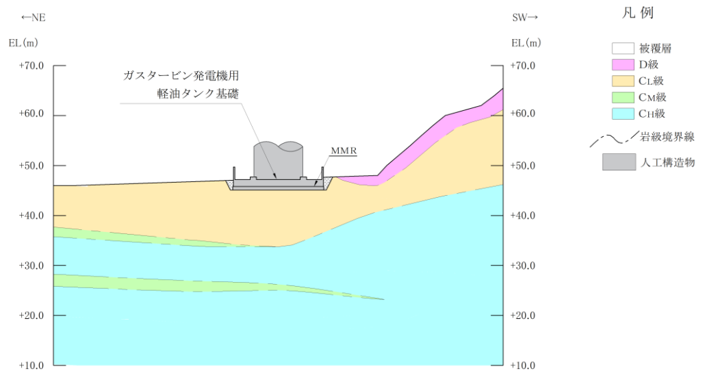
(岩級図)
