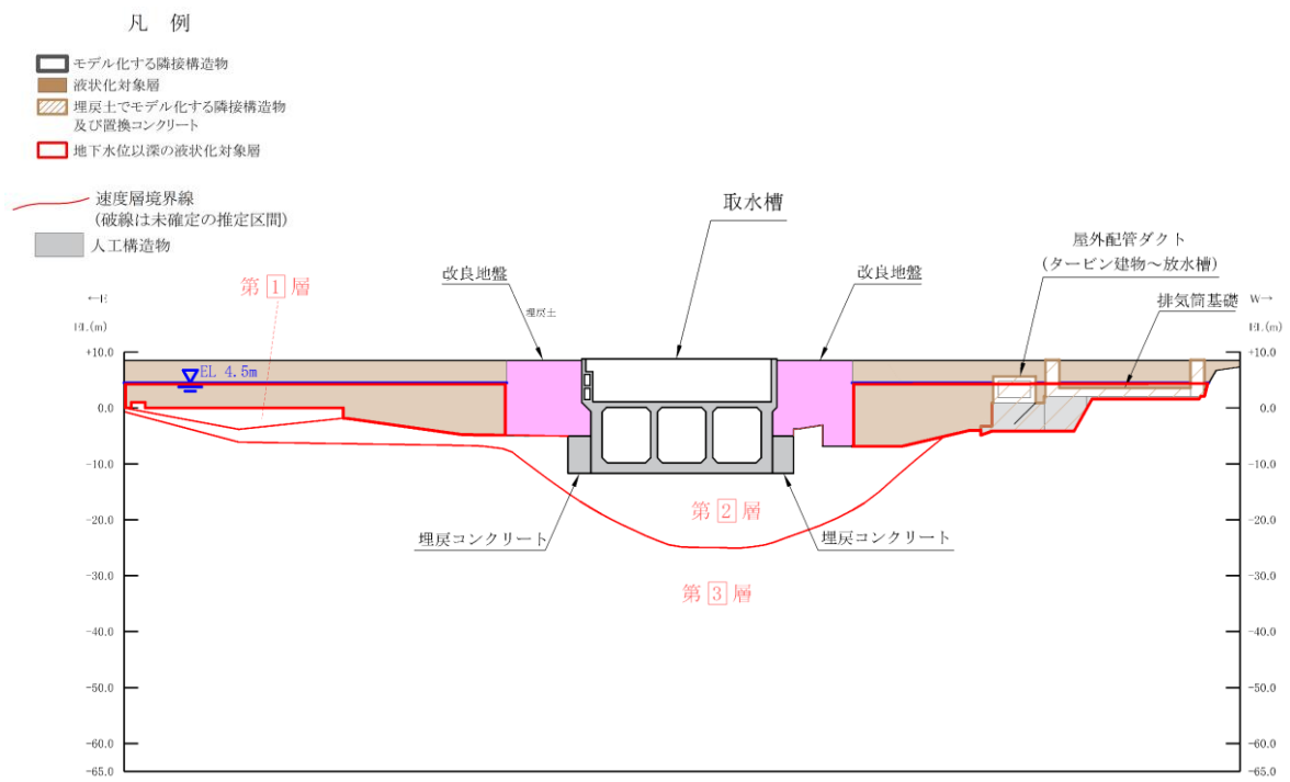
図 4.3-2(15) 取水槽【B-B断面】 地質断面図 (⑤有効応力解析)
