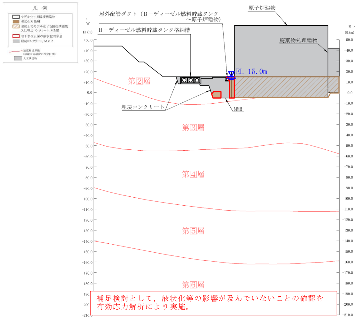
図 4.3-2(13) B-ディーゼル燃料貯蔵タンク格納槽 地質断面図【A-A断面】 (④全応力解析)
