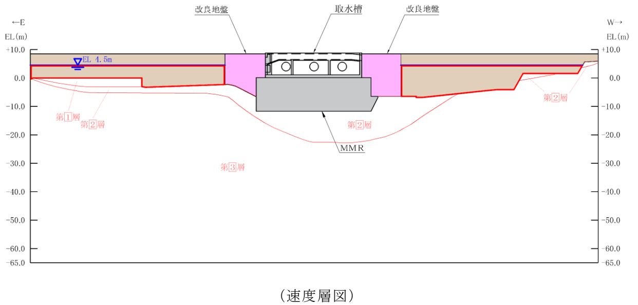
図 4.4-5 (3) 取水槽 地質断面図 (C-C断面)
