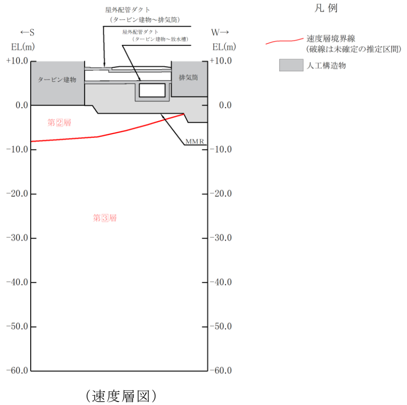
図 4.5-5 屋外配管ダクト (タービン建物～排気筒) 地質断面図 (C-C断面)
