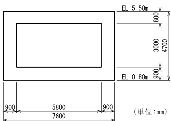
図 4.8-3 (2) 屋外配管ダクト (タービン建物～放水槽) 断面図 (C-C 断面)
