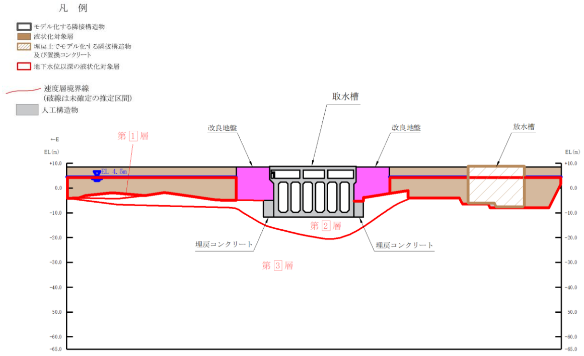
図 4.3-2(14) 取水槽【A-A断面】 地質断面図 (⑤有効応力解析)
