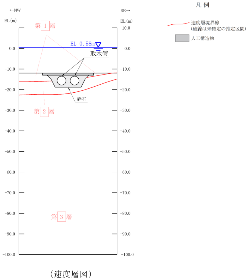
図 4.9-4 (2) 取水管 地質断面図 (C-C断面)
