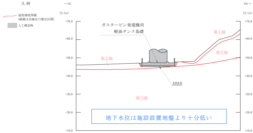
図 4.3-2(1) ガスタービン発電機用軽油タンク基礎 地質断面図
