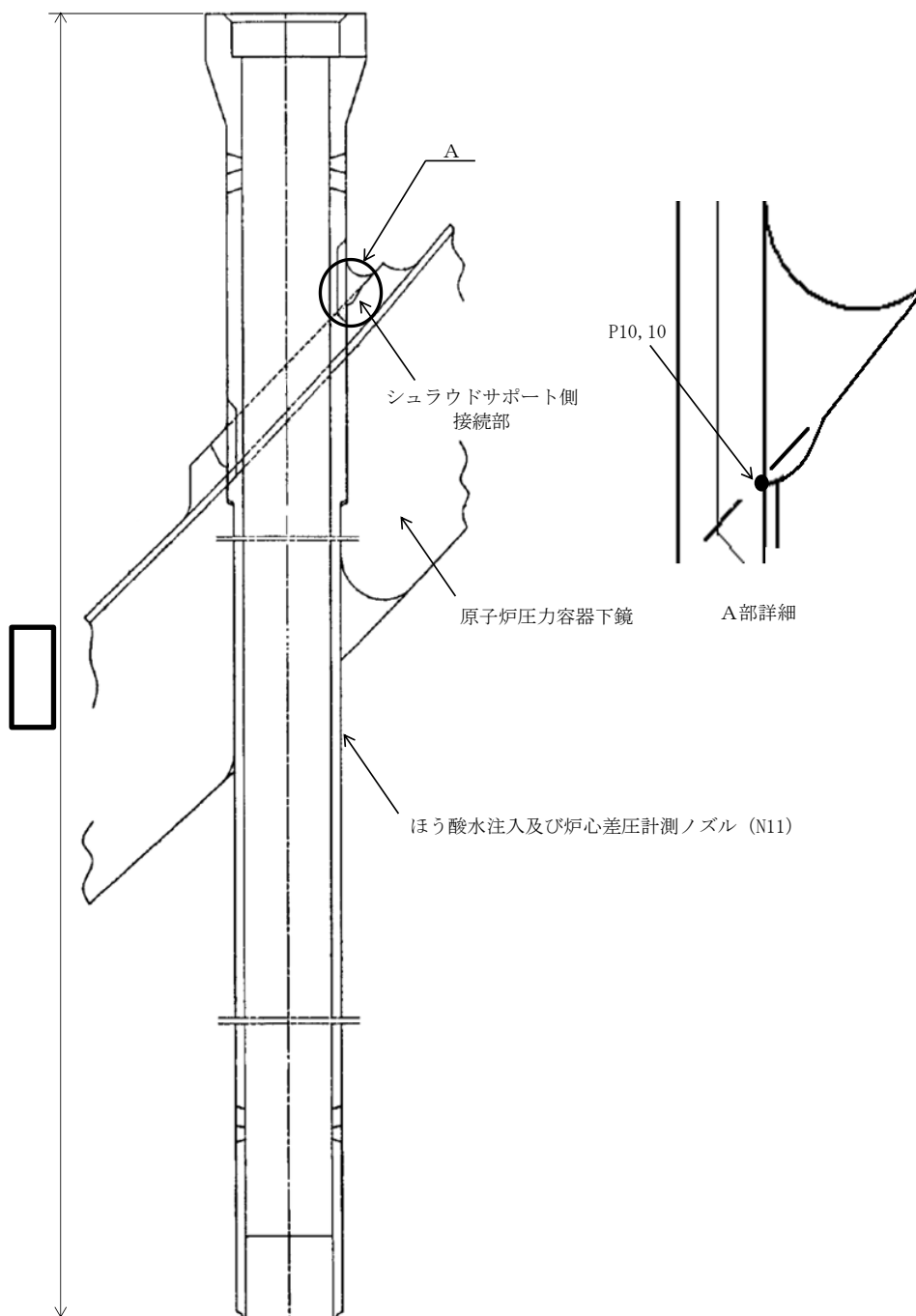
図1 ほう酸水注入及び炉心差圧計測ノズル (N11) の応力計算書構造図
