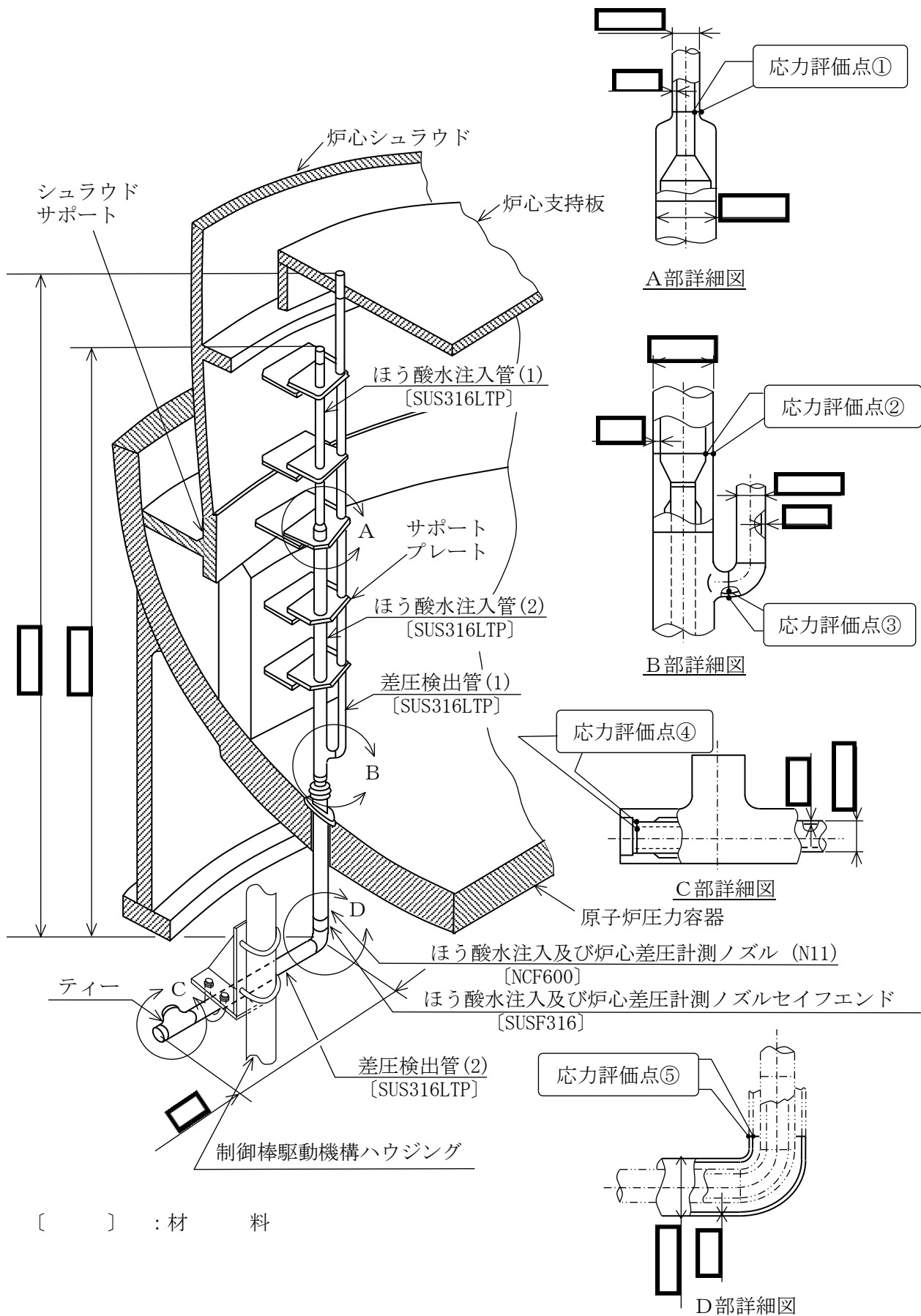
図2 本設備の応力評価点
