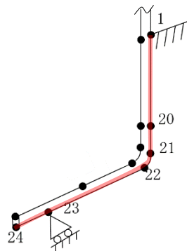
本設備の解析モデル
