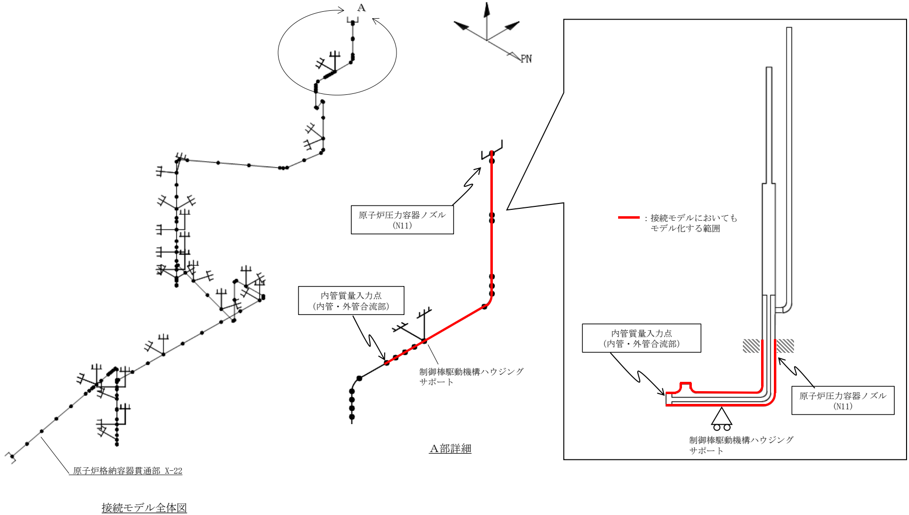
図3 接続配管の解析モデル
