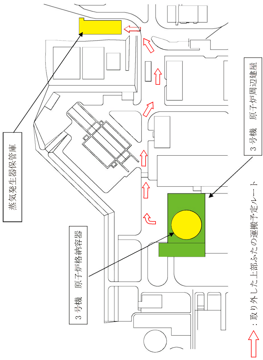
図2 原子炉容器上部ふたの運搬方法及び運搬予定ルート
