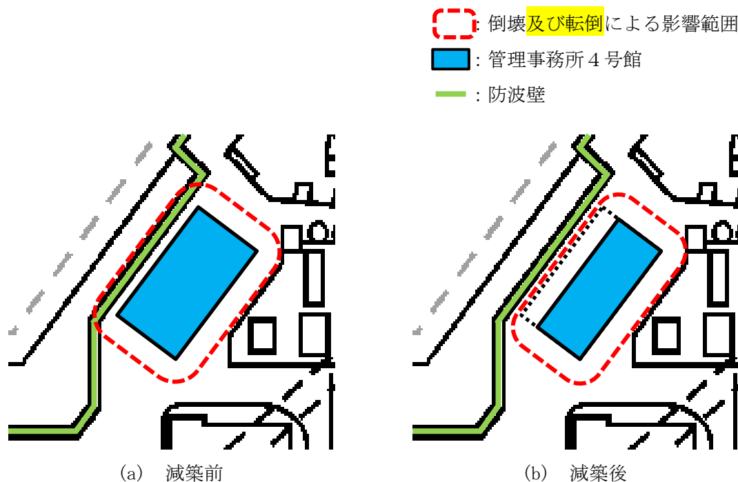
図6-3 管理事務所4号館の減築前後の倒壊及び転倒による影響範囲
