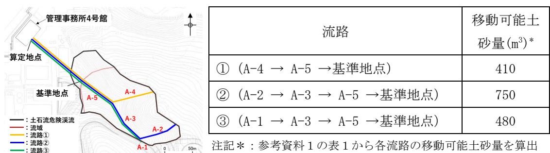
図6-8 土石流危険溪流⑦の各流路の移動可能土砂量
