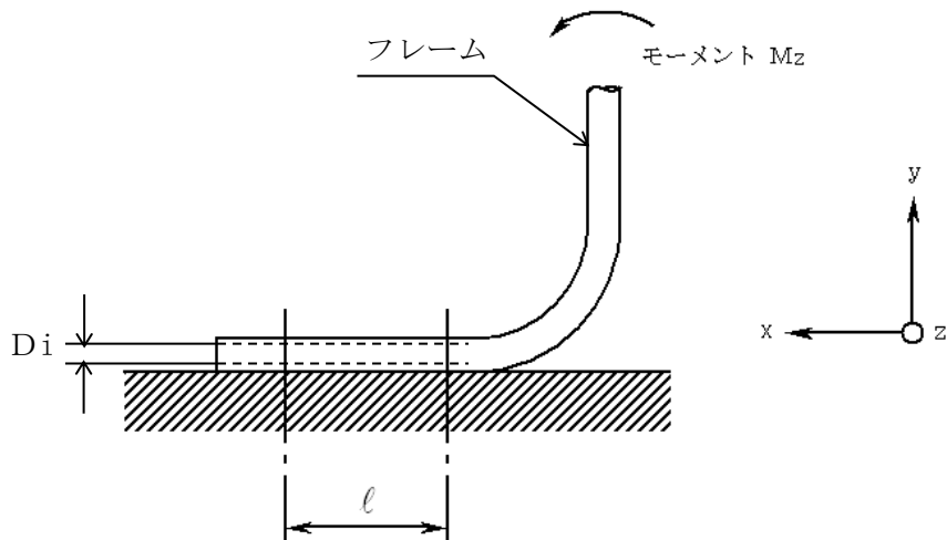
図 4-3 取付ボルト部の概要
