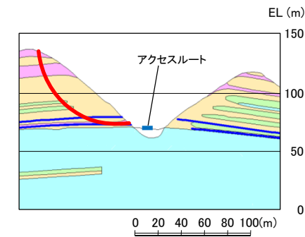
⑭-⑭' 断面
