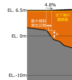
③-③断面
