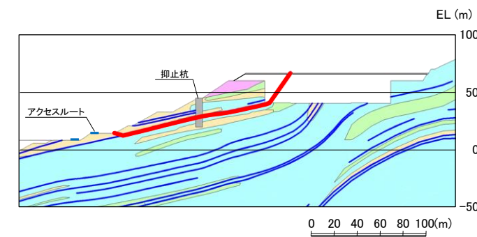
①-①' 断面
