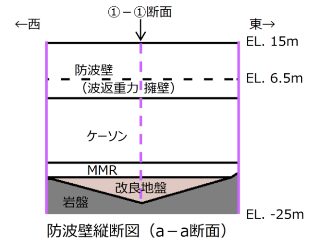
図 3-15 3 号機北西側における防波壁 (波返重力擁壁) (縦断図)
