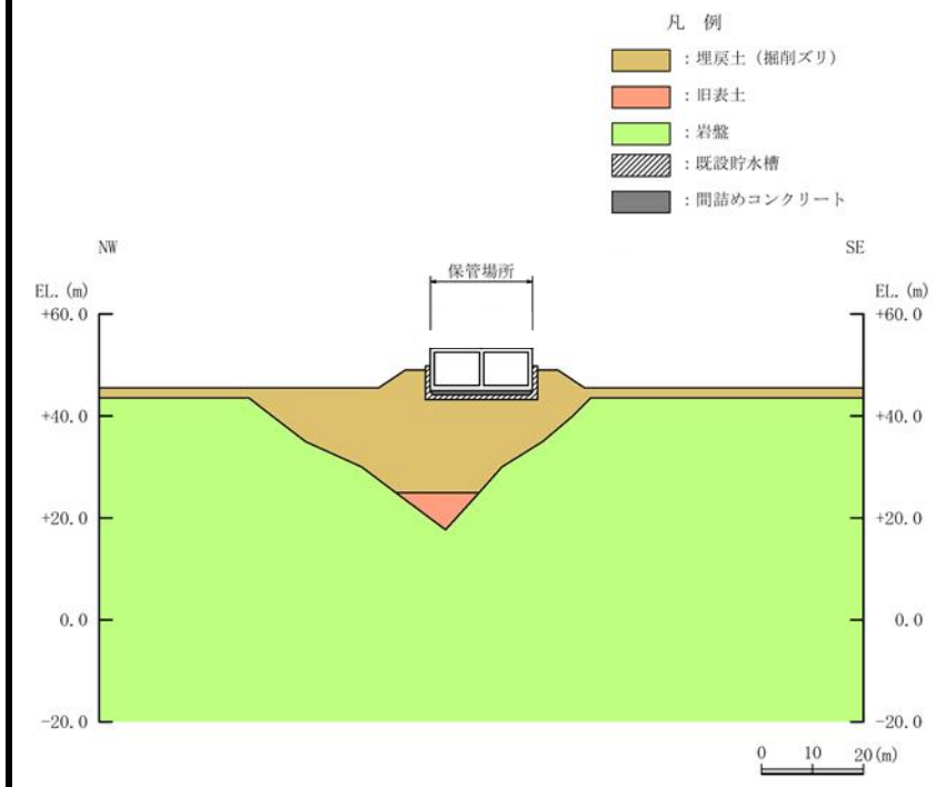
図 2-9 保管場所 (第 2 保管エリア) の地中埋没構造物 (輪谷貯水槽(西 1/西 2))
