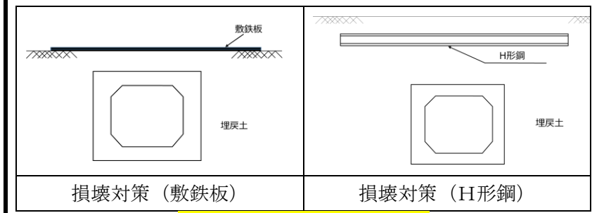
図 3-19 損壊対策の概念図
