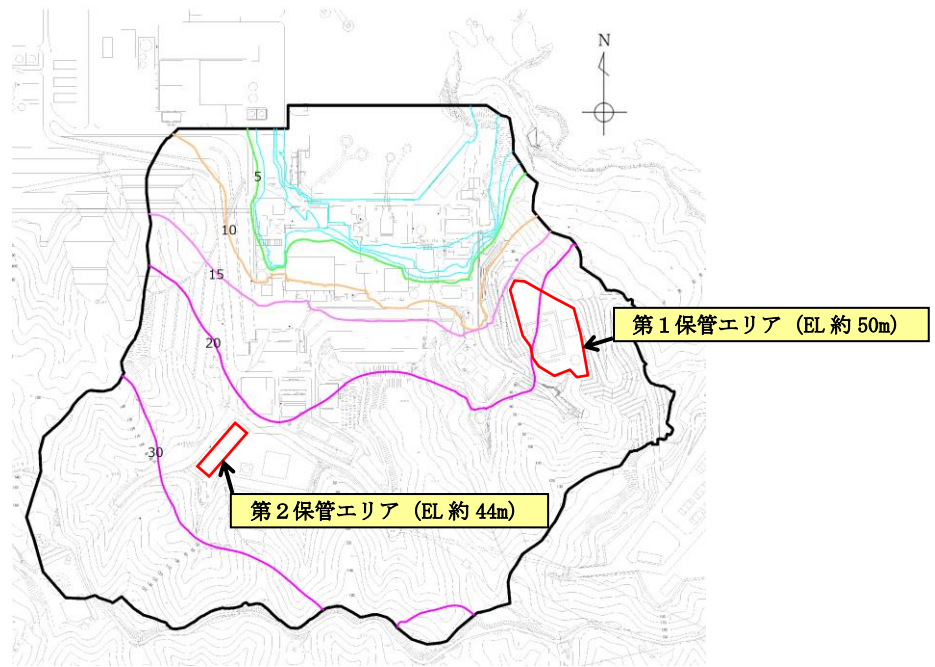
1, 2号機エリア
