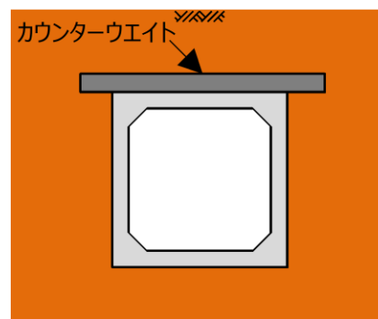
図 3-12 浮き上がり対策
