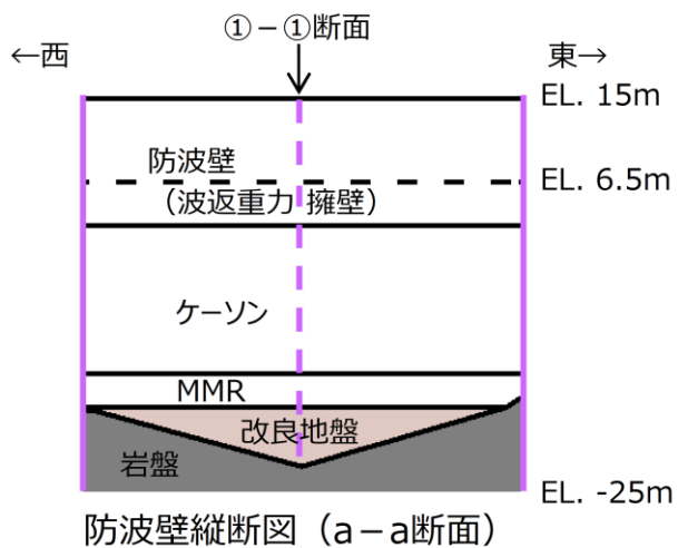
図 3-15 3号機北西側における防波壁（波返重力擁壁）（縦断図）
