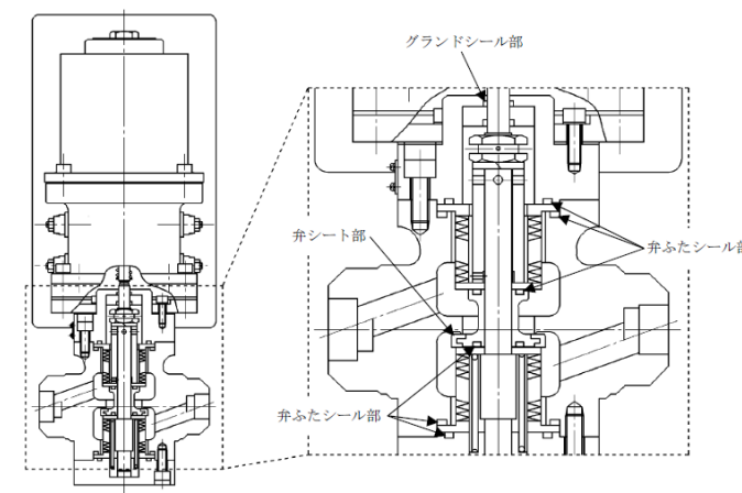
図 10-4 T I P プラグ弁評価対象
