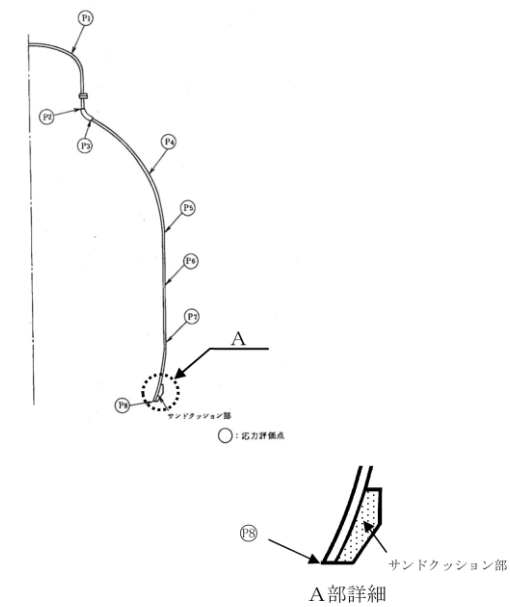
図 4-1 応力評価点
