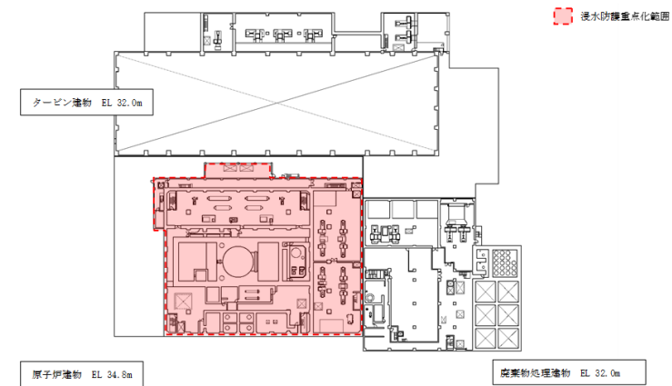
図 3-29(3) 浸水防護重点化範囲 (平面図) (3/4)
