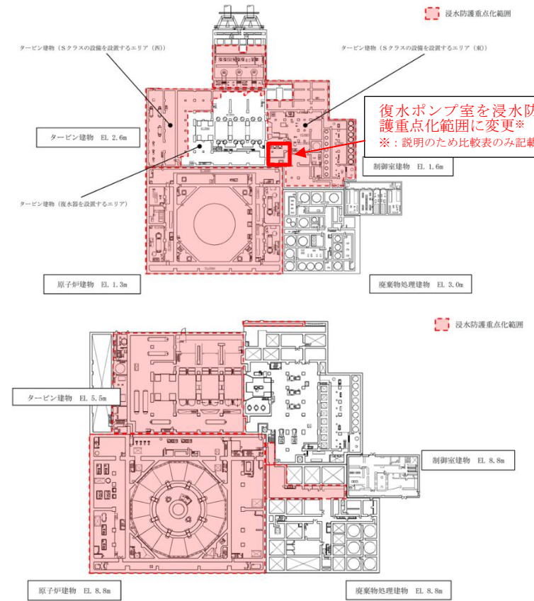
図 3-29(1) 浸水防護重点化範囲 (平面図) (1/4)
