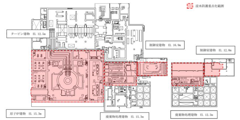
図 3-29(2) 浸水防護重点化範囲 (平面図) (2/4)
