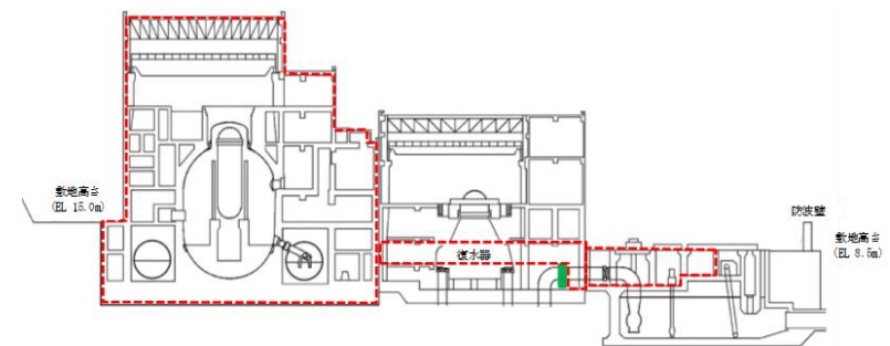
図 3-29(5) 浸水防護重点化範囲 (断面図)
