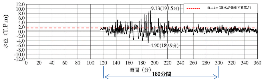
図 3-24 漏水による浸水量評価
