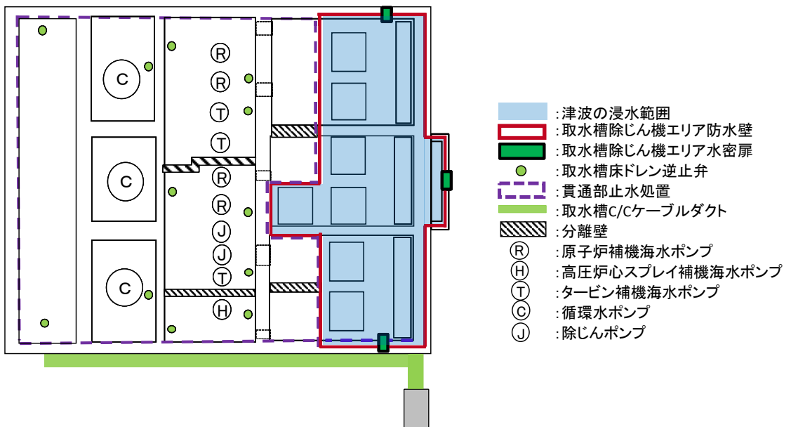
図 3-8 取水槽の浸水対策の概要 (平面図)
