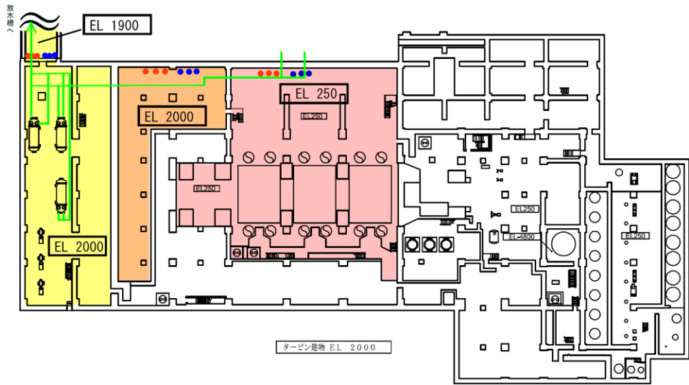
タービン建物
