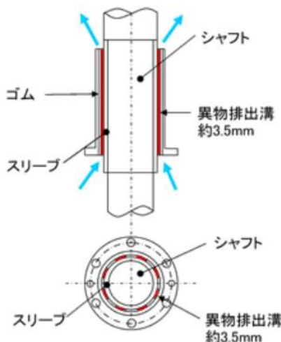
図 3-38 海水ポンプ軸受構造図
