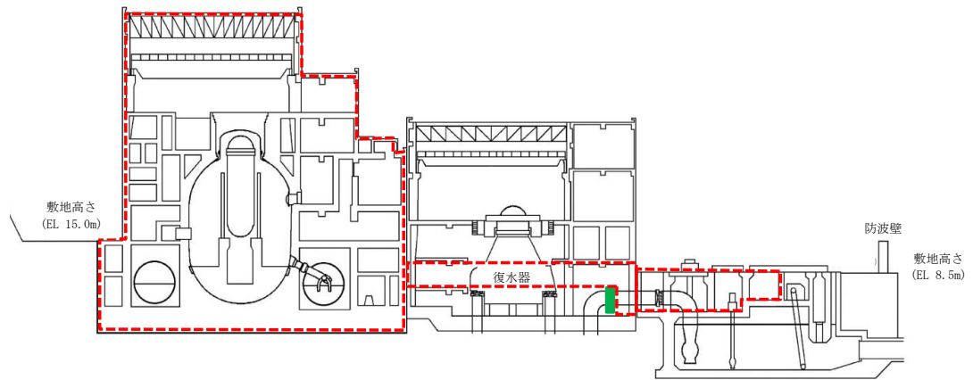
図 3-29(5) 浸水防護重点化範囲 (断面図)
