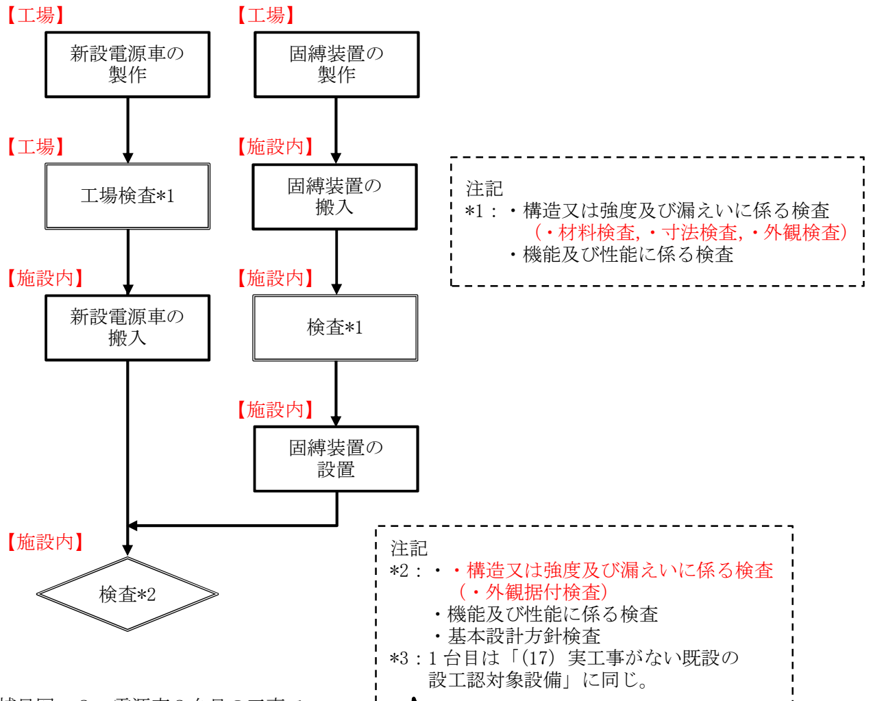
補足図-2 電源車2台目の工事フロー
