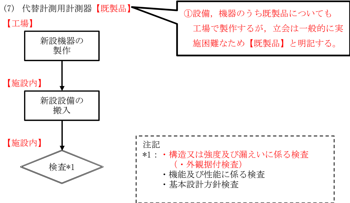
補足図－4 代替計測用計測器の工事フロー
