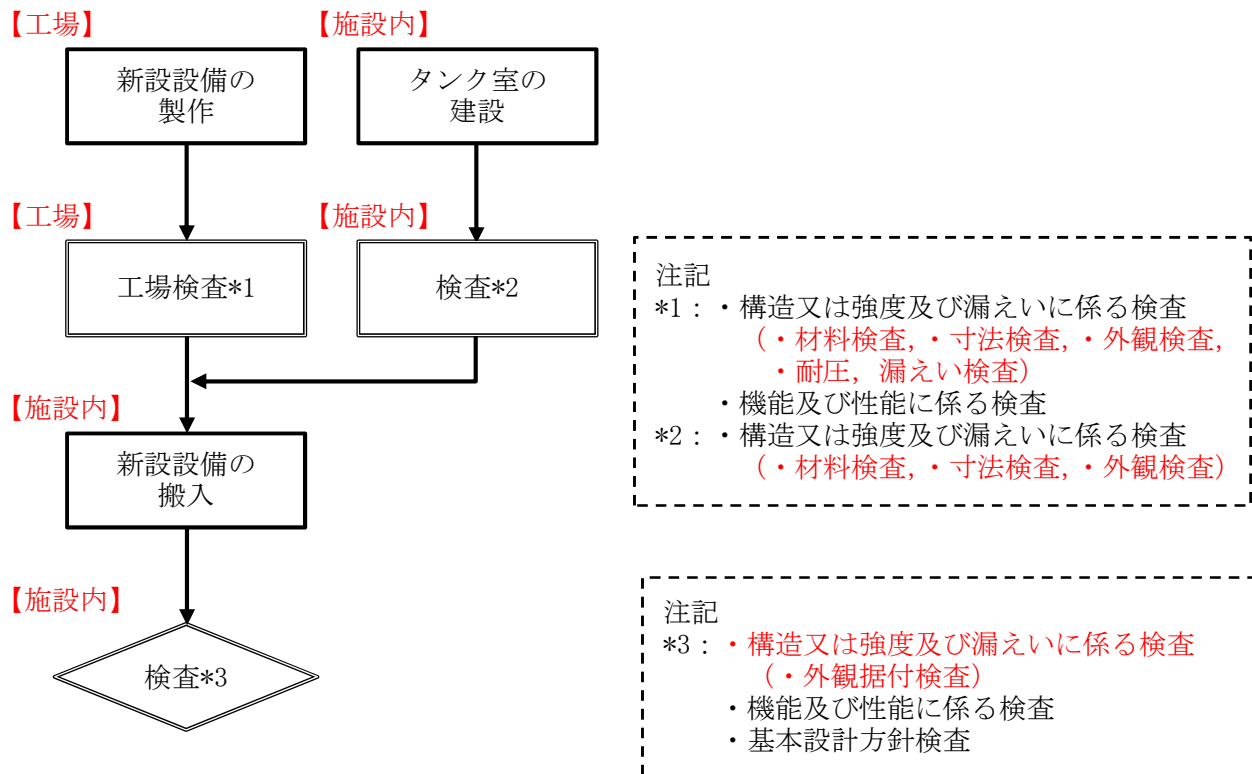
補足図－5 軽油貯蔵タンク（地下式）の工事フロー
