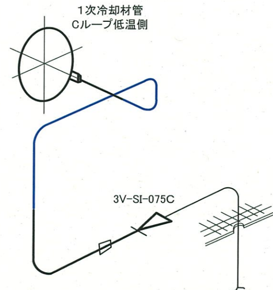
○工事後の配管ルート
