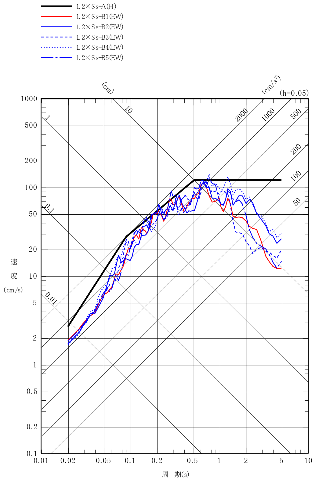
第 6-1 図(2) 1.2 \times S_s - A と 1.2 \times S_s - B の応答スペクトル (EW 方向)
