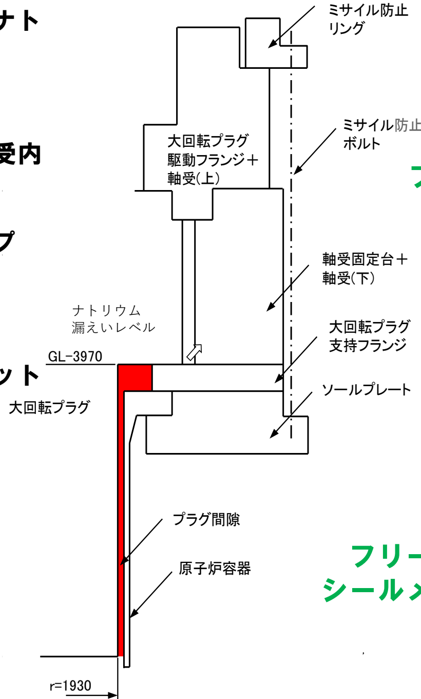
大回転プラグの構造概要
