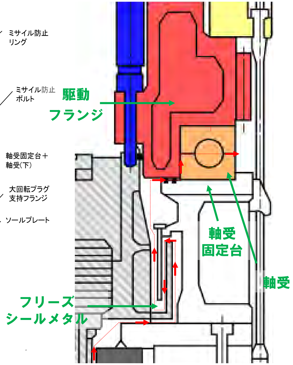
大回転プラグの構造概要
