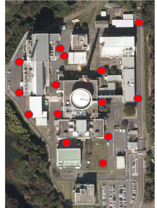
● : 屋外消火栓
