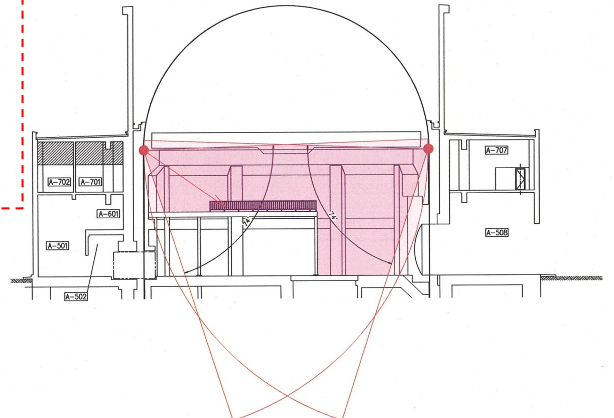
B-B断面
