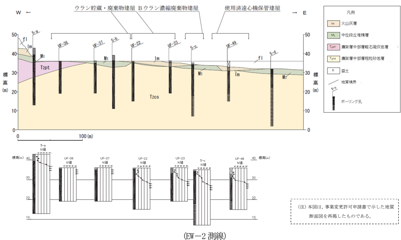
図3 地質断面図 (1/2)
