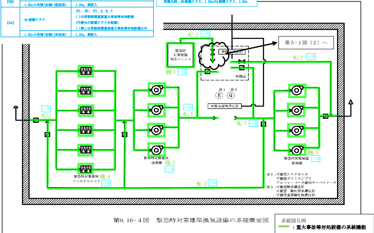
第5-1図(1) 緊急時対策建屋換気設備の耐震クラス範囲の概要図 (事業許可変更申請書 添付書類六 第9.16-4図抜粋)
