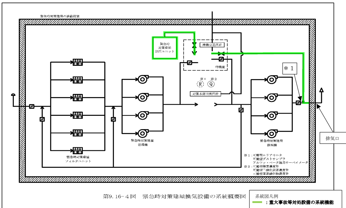
第2-3図 緊急時対策建屋換気設備 系統概要図（緊急時対策建屋加圧ユニットによる加圧） （事業許可変更申請書 添付書類六 第9.16-4図抜粋）
