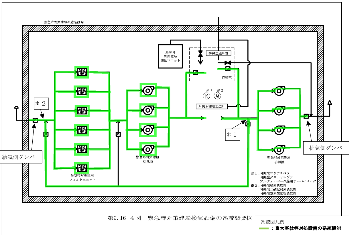
第2-2図 緊急時対策建屋換気設備 系統概要図（再循環モード） （事業許可変更申請書 添付書類六 第9.16-4図抜粋）
