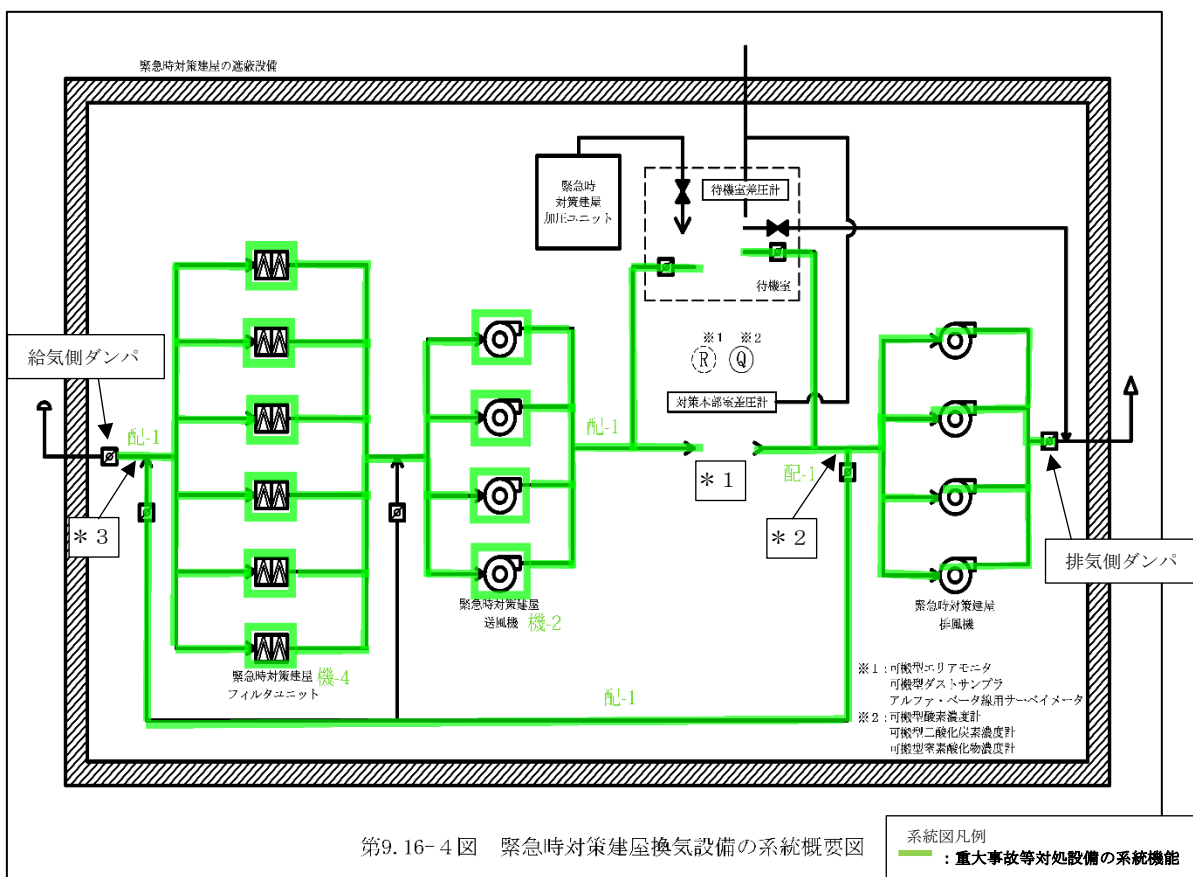
第3-2図 緊急時対策建屋換気設備 系統概要図 (再循環モード)
