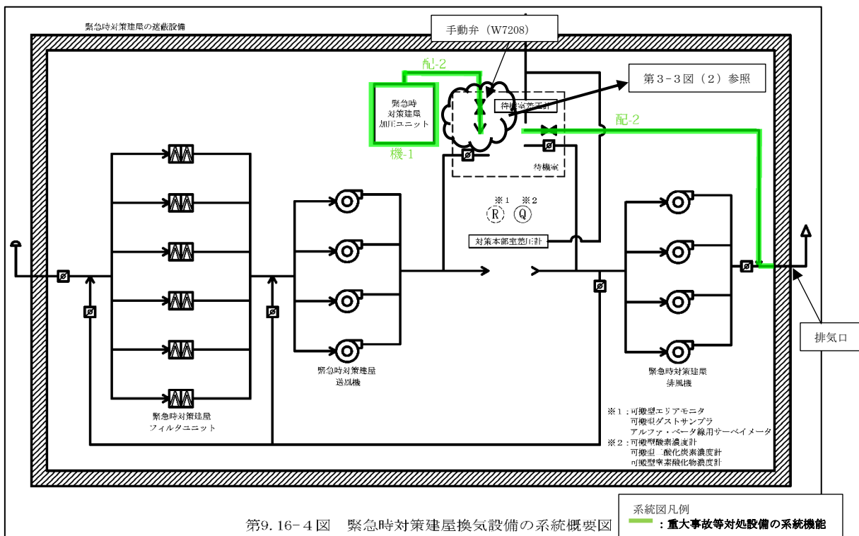
第3-3図(1) 緊急時対策建屋換気設備 系統概要図 (緊急時対策建屋加圧ユニットによる加圧) (事業許可変更申請書 添付書類六 第9.16-4図抜粋)
