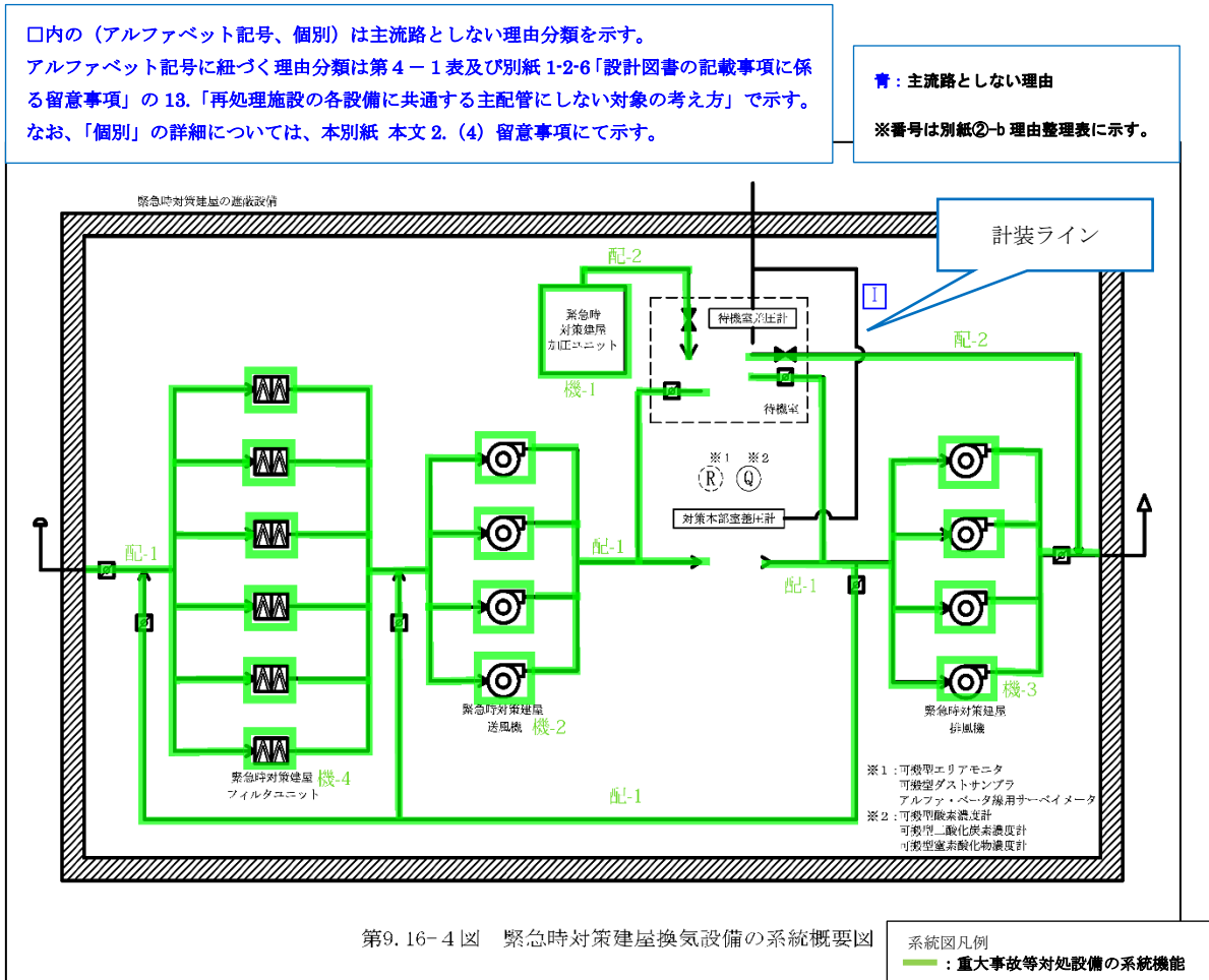
第4-3図 緊急時対策建屋換気設備に係る主流路の範囲及び主流路としていない範囲の概要図
