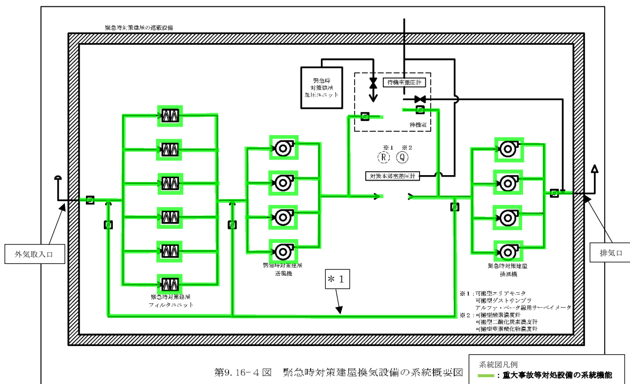
第2-1図 緊急時対策建屋換気設備 系統概要図（外気取入加圧モード）
