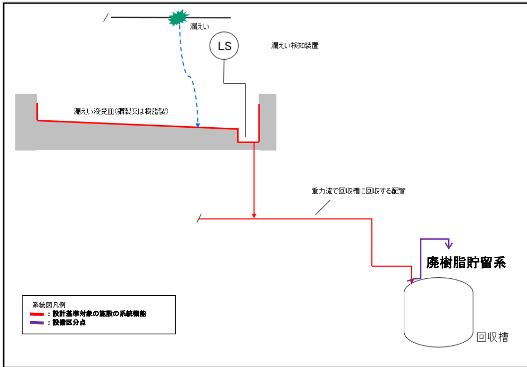
第2-2図 低レベル廃液等の漏えい液の保持 (漏えいした溶液の保持、重力流による回収)
