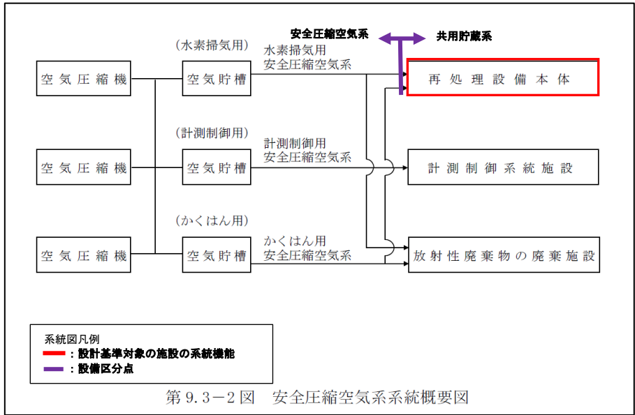
第 2 - 5 図 安全圧縮空気系 系統概要図 (事業変更許可申請書 添付書類六 第9.3-2 図抜粋)
