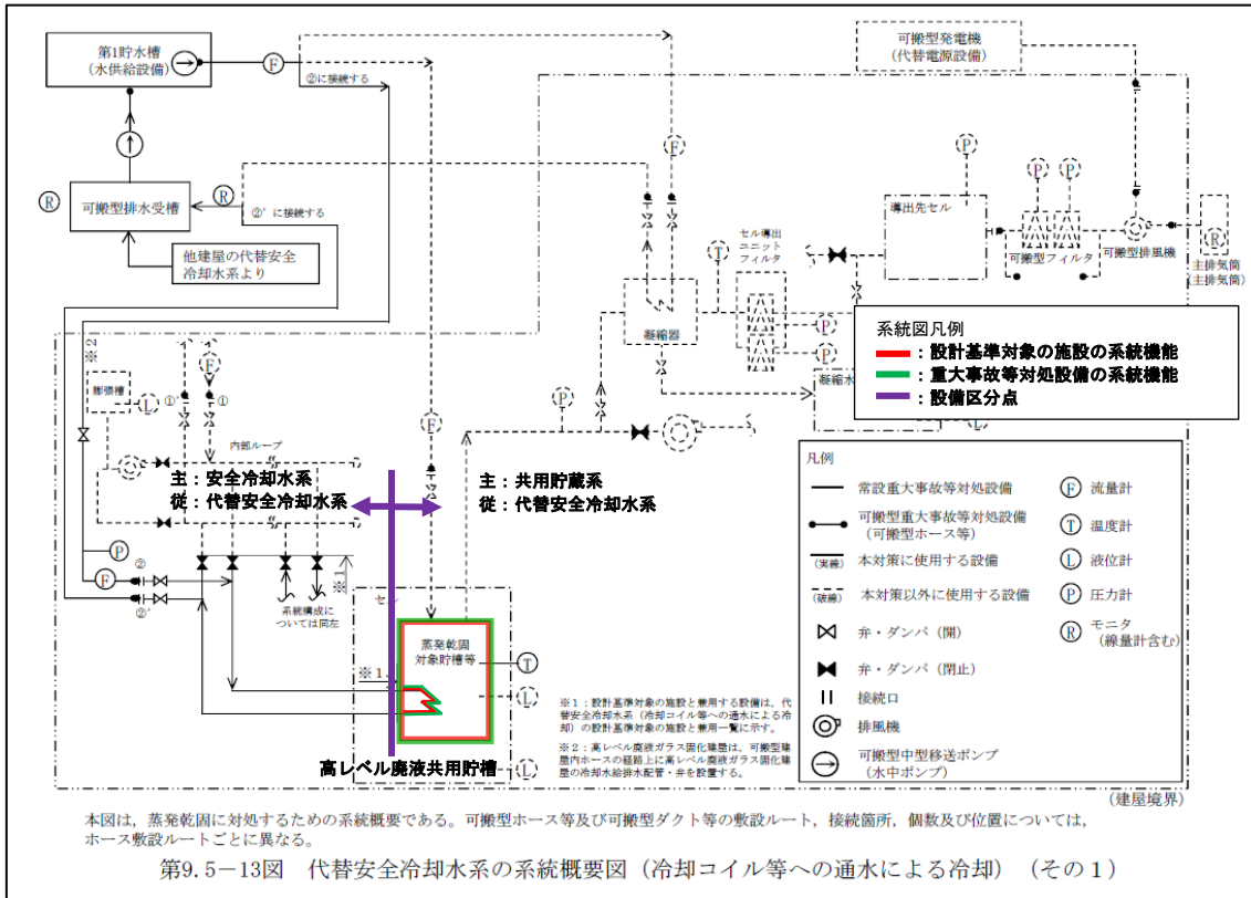
第2-8図 代替安全冷却水の系統概要図 (冷却コイル等への通水による冷却) (事業変更許可申請書 添付書類六 第9.5-13図抜粋)
