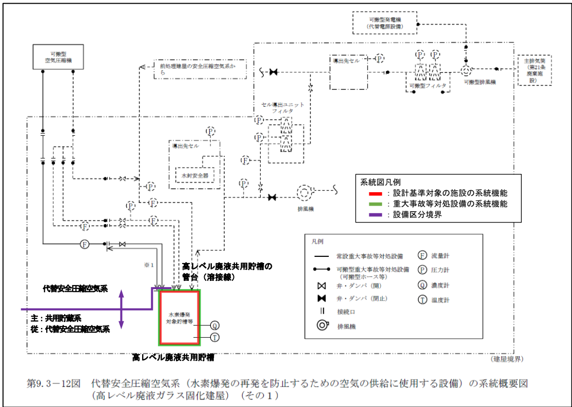
第3-10図 代替安全圧縮空気系（水素爆発の再発を防止するための空気供給に使用する設備） 系統概要図 （事業変更許可申請書 添付書類六 第9.3-12図抜粋）
