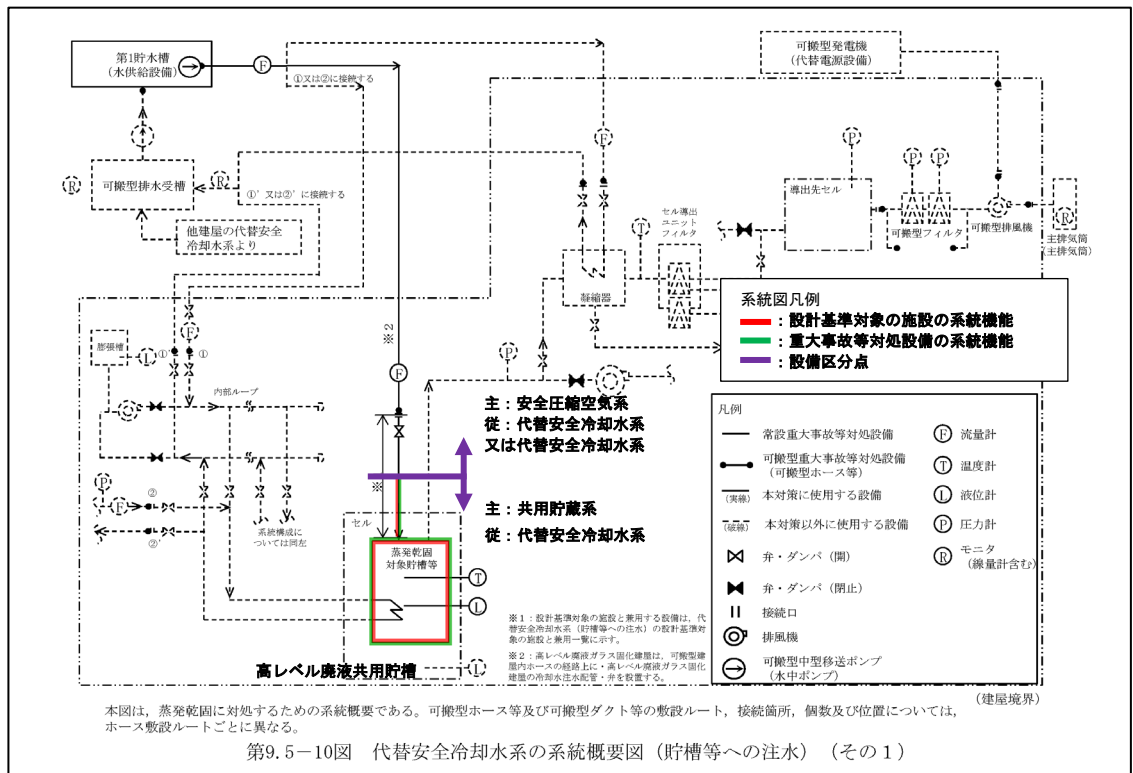
第2-7図 代替安全冷却水系の系統概要図 (貯槽等への注水) (事業変更許可申請書 添付書類六 第9.5-10図抜粋)
