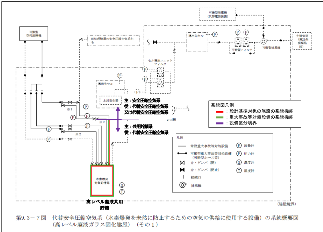
第2-10図 代替安全圧縮空気系（水素爆発を未然に防止するための空気供給に使用する設備）の系統概要図 （事業変更許可申付書類六 第9.3-7図抜粋）
