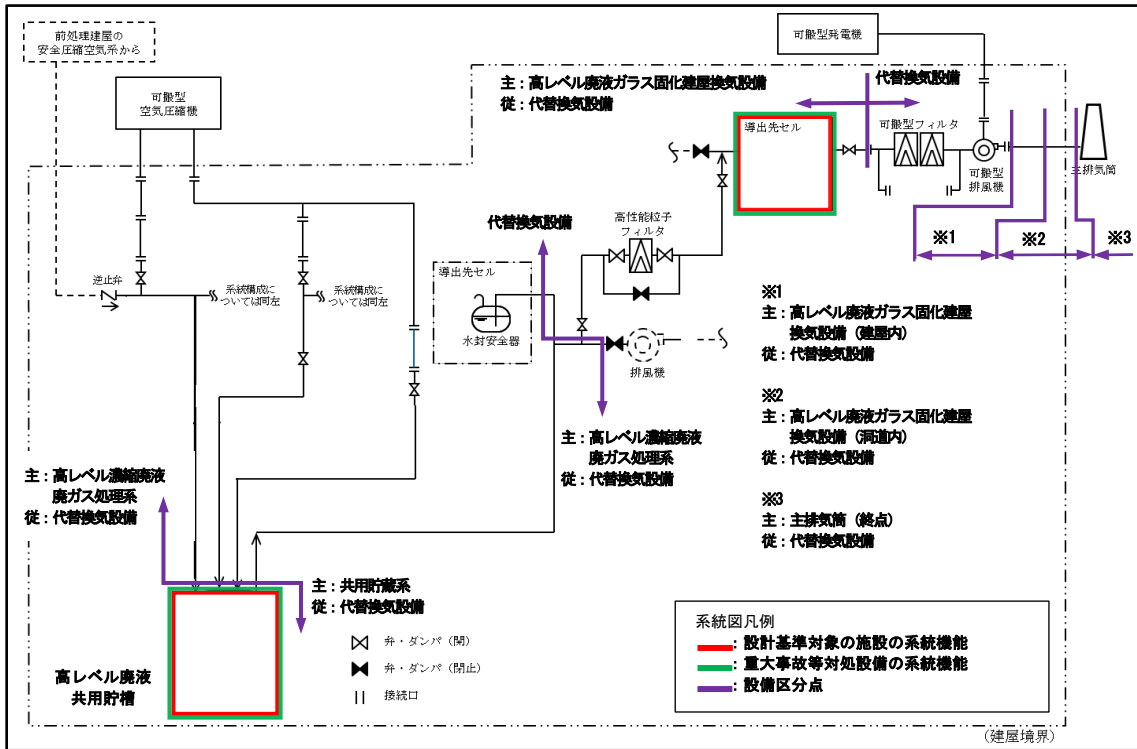
第 3 - 11 図 代替換気設備 系統概要図
