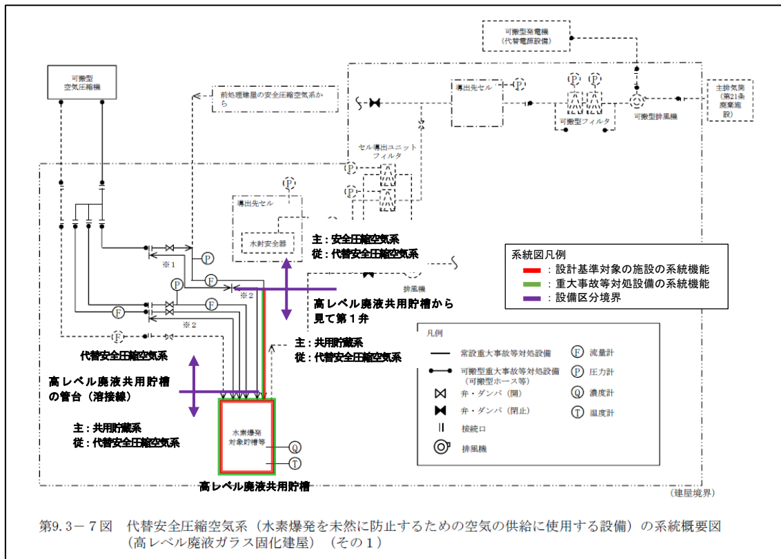
第3-9図 代替安全圧縮空気系（水素爆発を未然に防止するための空気供給に使用する設備） 系統概要図 （事業変更許可申付書類六 第9.3-7図抜粋）
