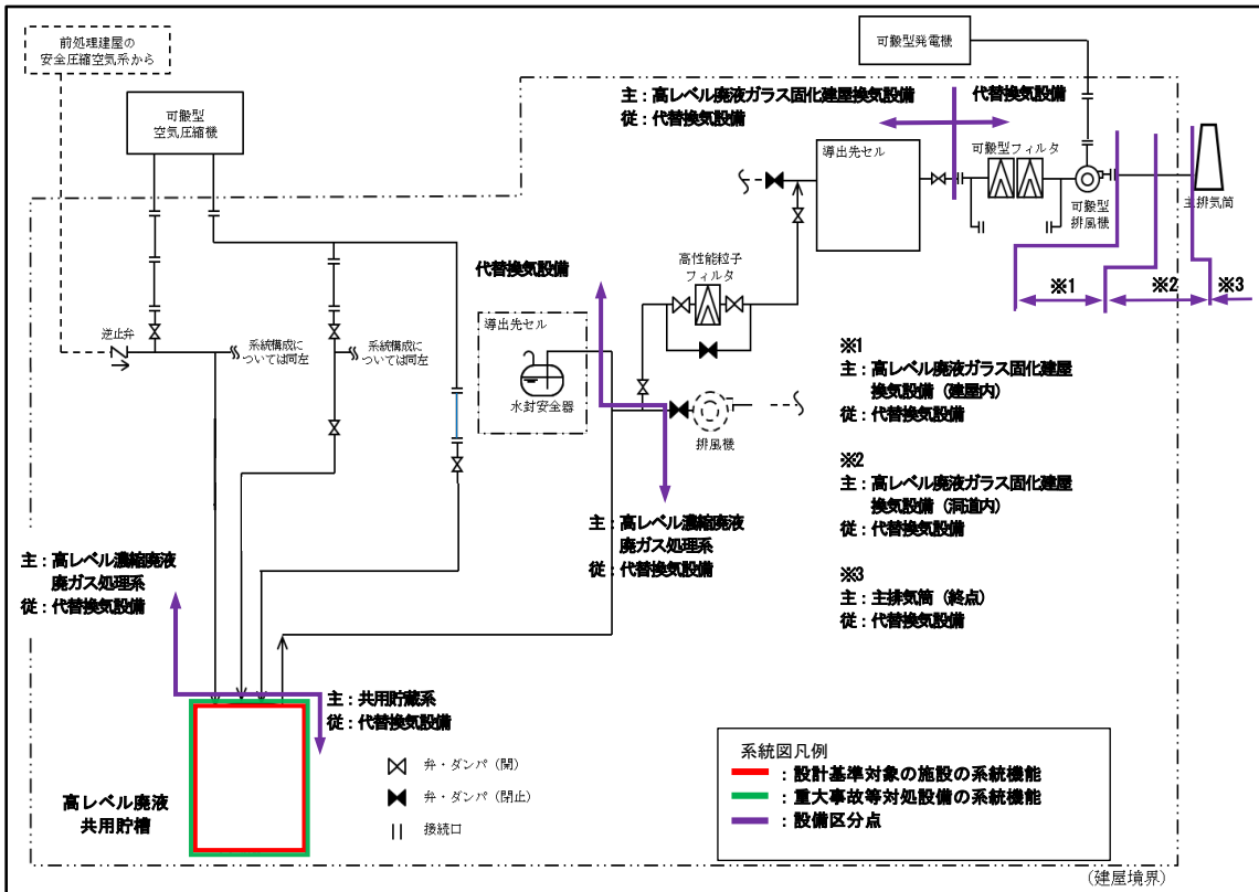
第2-12図 代替換気設備 系統概要図 (事業変更許可申請書 添付書類六 第7.2-38図(1)抜粋)
