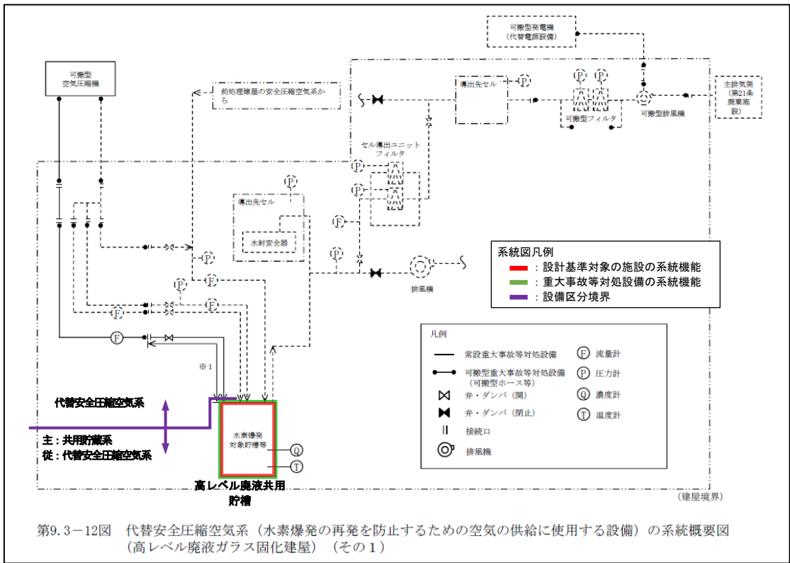
第2-11図 代替安全圧縮空気系（水素爆発の再発を防止するための空気供給に使用する設備）の系統概要図 （事業変更許可申請書 添付書類六 第9.3-12図抜粋）
