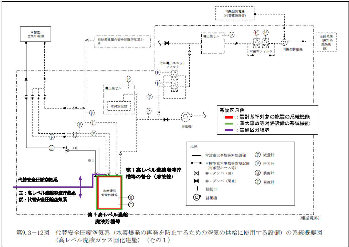
第3-12図 代替安全圧縮空気系（水素爆発の再発を防止するための空気の供給に使用する設備） 系統概要図 （事業変更許可申請書 添付書類六 第9.3-12図抜粋）
