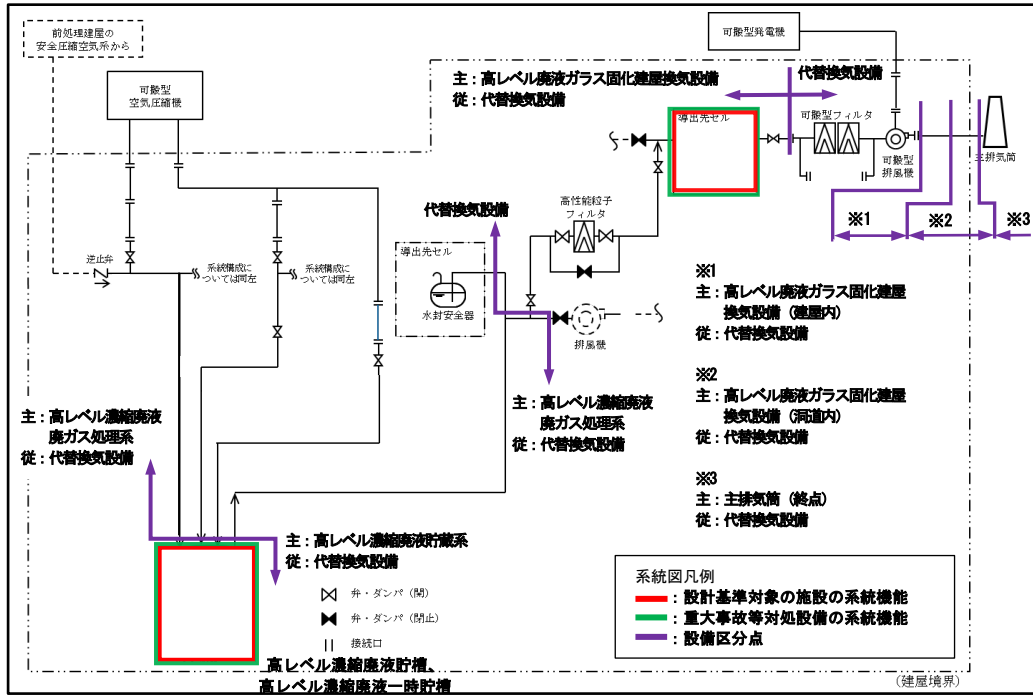
第2-15図 代替換気設備 系統概要図
