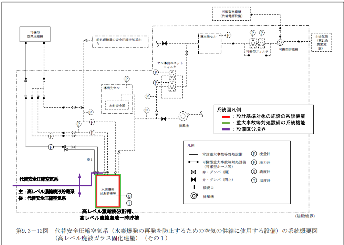
第2-14図 代替安全圧縮空気系（水素爆発の再発を防止するための空気の供給に使用する設備）の系統概要図 （事業変更許可申請書 添付書類六 第9.3-12図抜粋）
