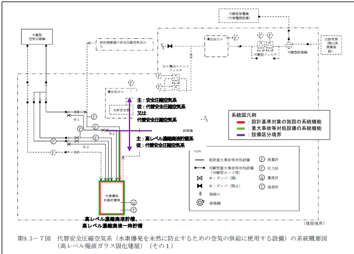
第2-13図 代替安全圧縮空気系（水素爆発を未然に防止するための空気の供給に使用する設備）の系統概要図（事業変更許可申付書類六 第9.3-7図抜粋）
