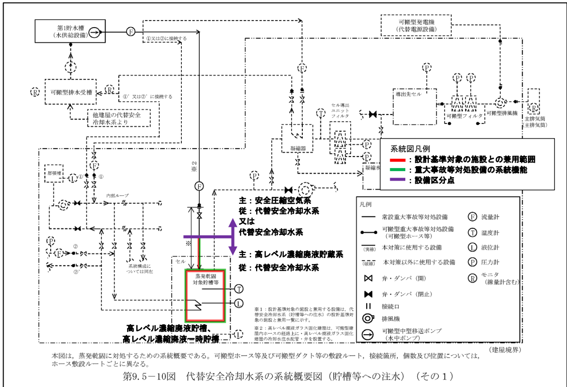
第2-10図 代替安全冷却水系の系統概要図 (貯槽等への注水) (事業変更許可申請書 添付書類六 第9.5-10図抜粋)
