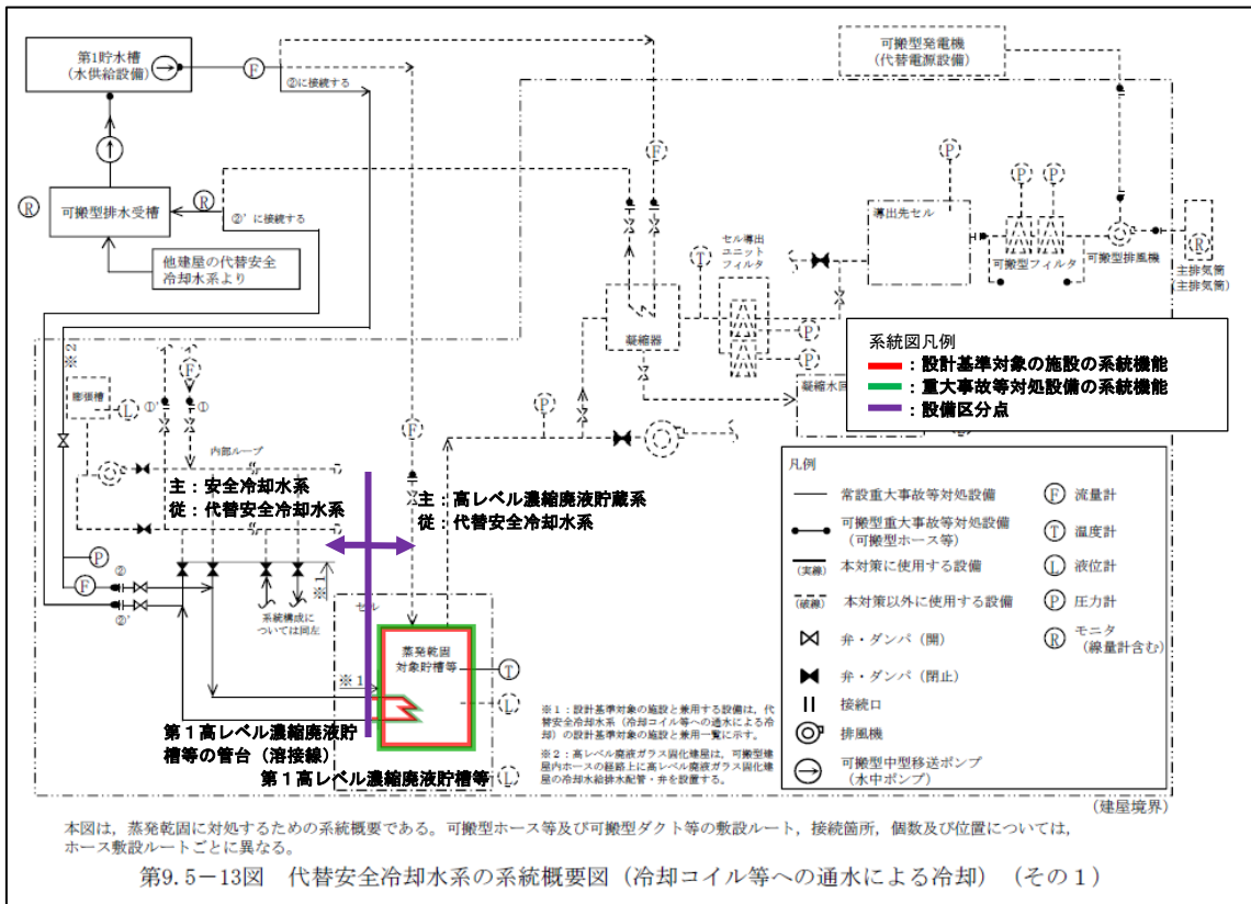
第3-9図 代替安全冷却水 系統概要図 (冷却コイル等への通水による冷却) (事業変更許可申請書 添付書類六 第9.5-13図抜粋)
