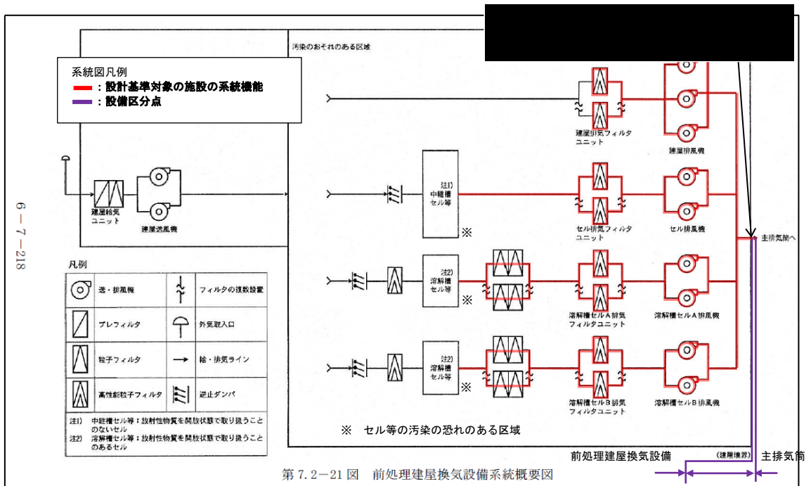
第 2 - 1 図 前処理建屋換気設備 系統概要図 (事業変更許可申請書 添付書類六 第7.2-21図抜粋)
