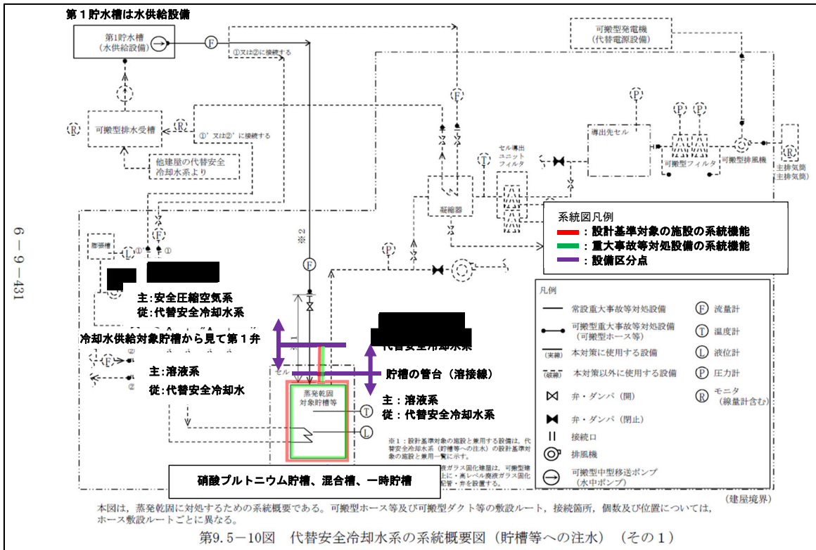
第3-9図(1) 代替安全冷却水系 系統概要図 (計装用空気ライン以外からの貯槽等への注水) (事業変更許可申請書 添付書類六 第9.5-10図抜粋)
