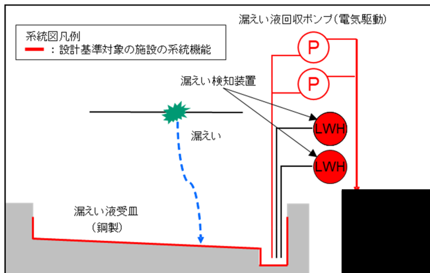
第 2 - 4 図 沸騰のおそれのある溶液の回収（ポンプによる回収）
