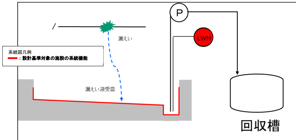
第 2 - 5 図 低レベル廃液の漏えい液の保持 (漏えいした溶液の保持)
