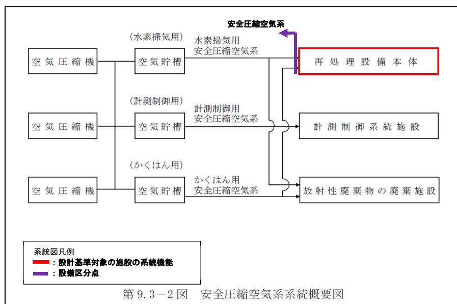
第2-7図 安全圧縮空気系 系統概要図
