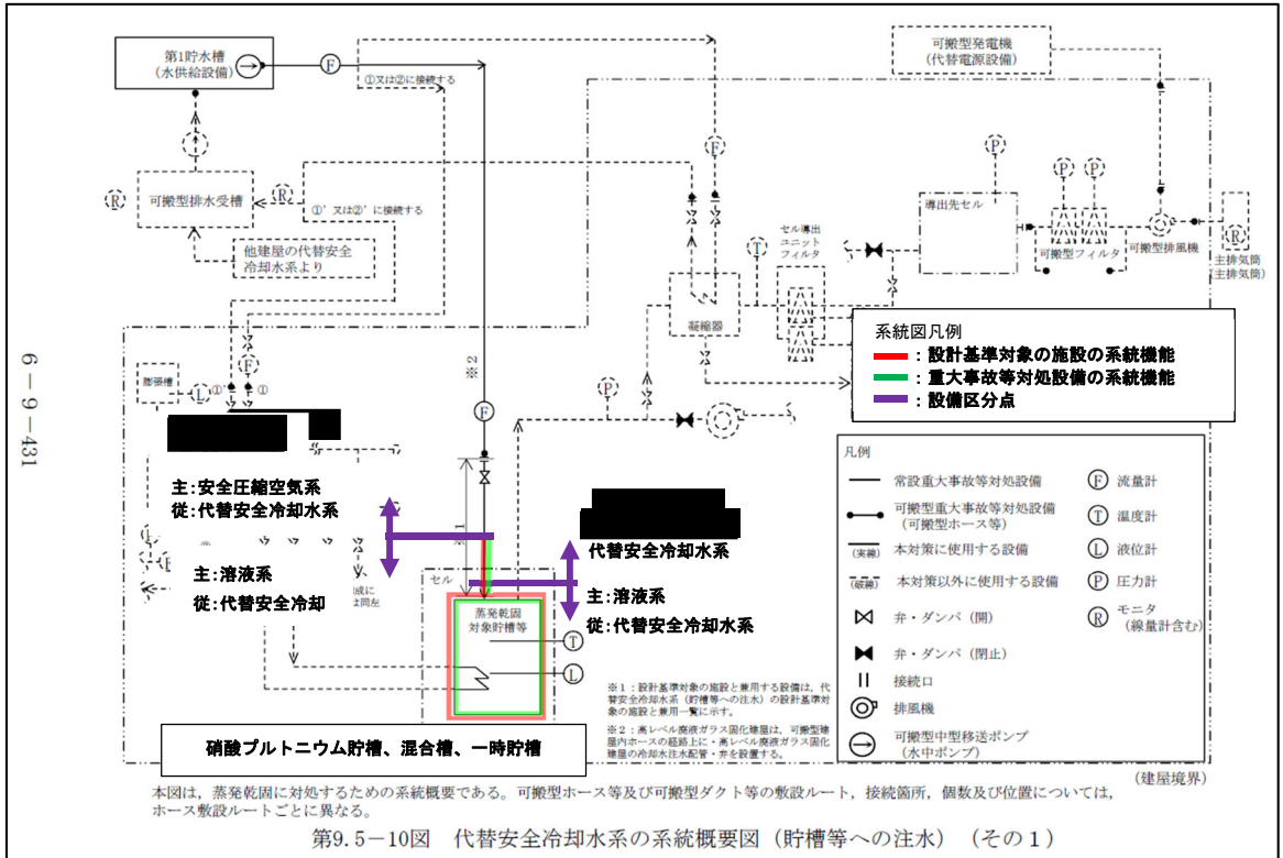
第2-9図 代替安全冷却水系 系統概要図 (事業変更許可申請書 添付書類六 第9.5-10図抜粋)
