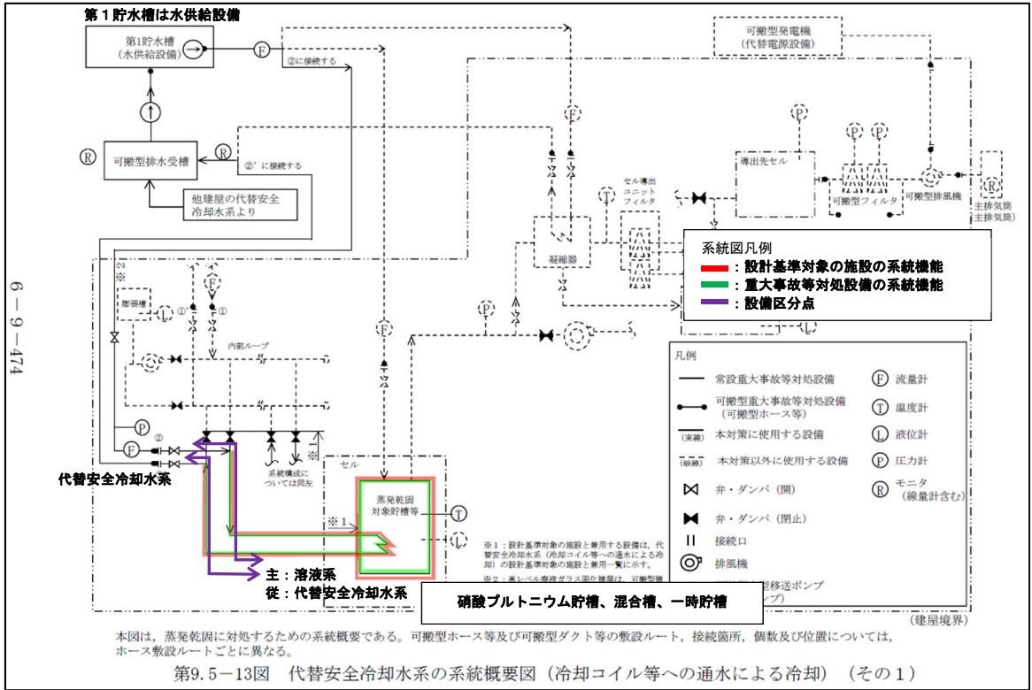
第2-10図 代替安全冷却水 系統概要図 (冷却コイル等への通水による冷却) (事業変更許可申請書 添付書類六 第9.5-13図抜粋)
