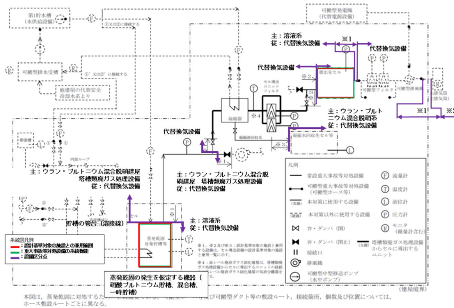
第3-11図 代替換気設備（セル導出設備） 系統概要図 （事業変更許可申請書 添付書類六 第7.2-37図(1)抜粋）
