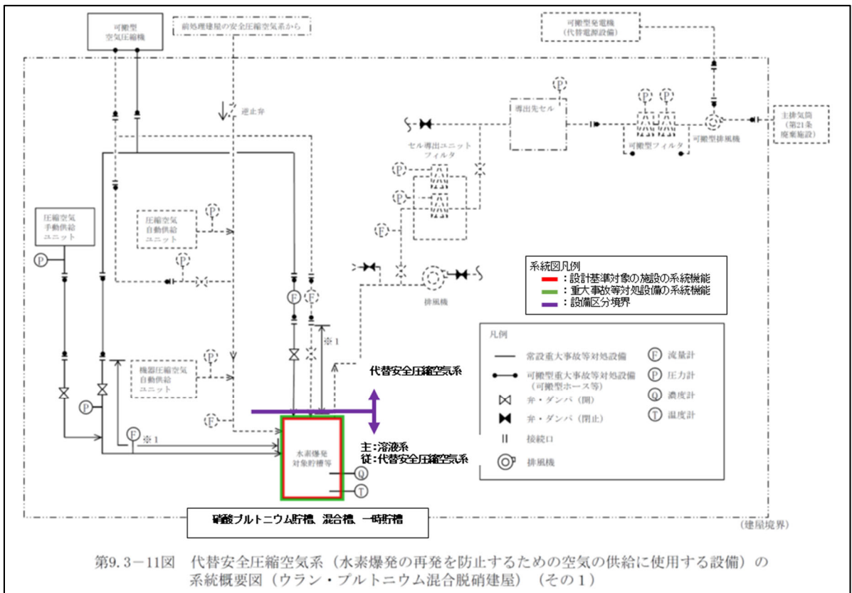
第2-13図 代替安全圧縮空気系（水素爆発の再発を防止するための空気の供給に使用する設備）の系統概要図 （事業変更許可申請書 添付書類六 第9.3-11図抜粋）
