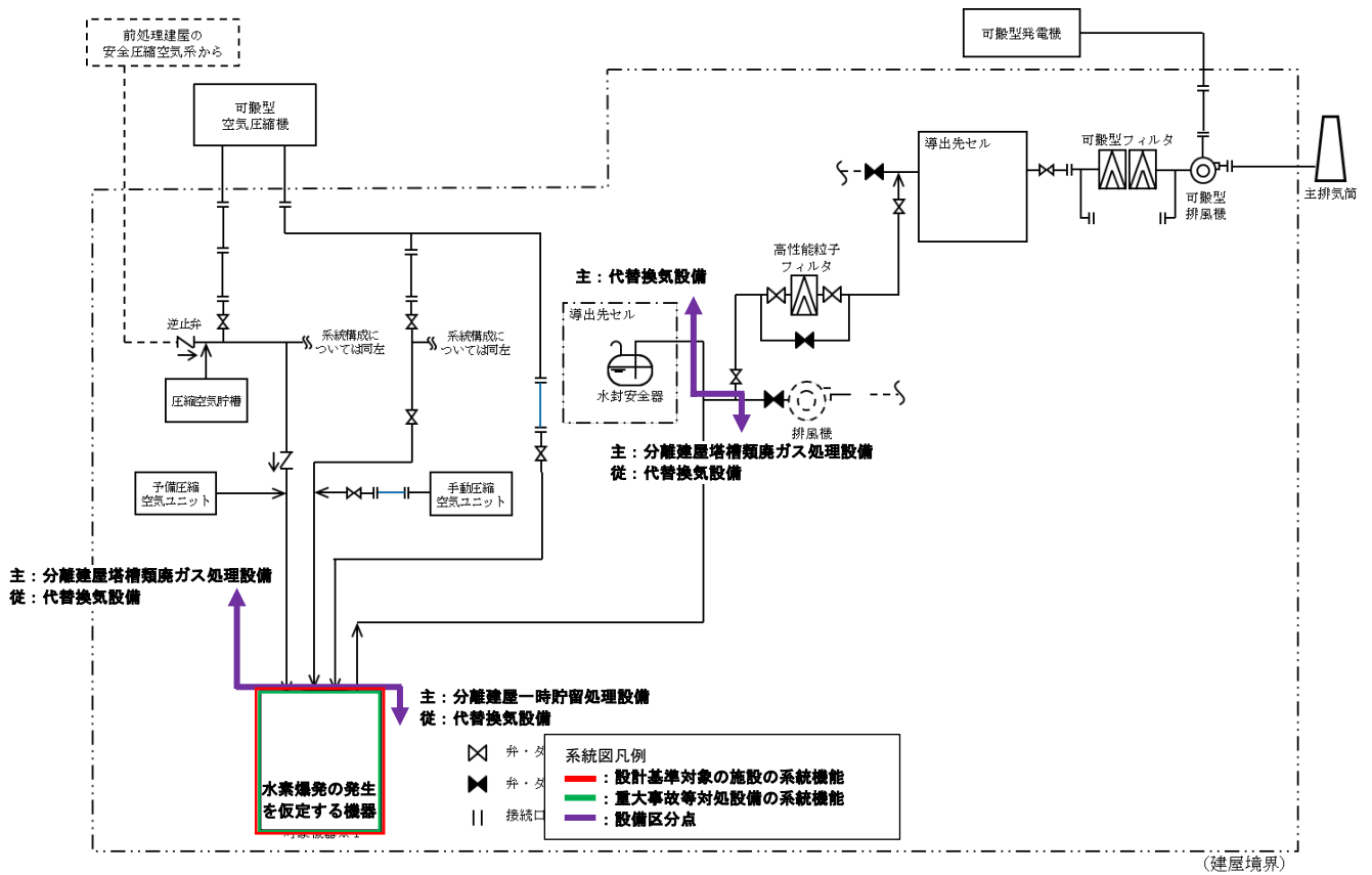
第3-14図 代替換気設備 系統概要図
