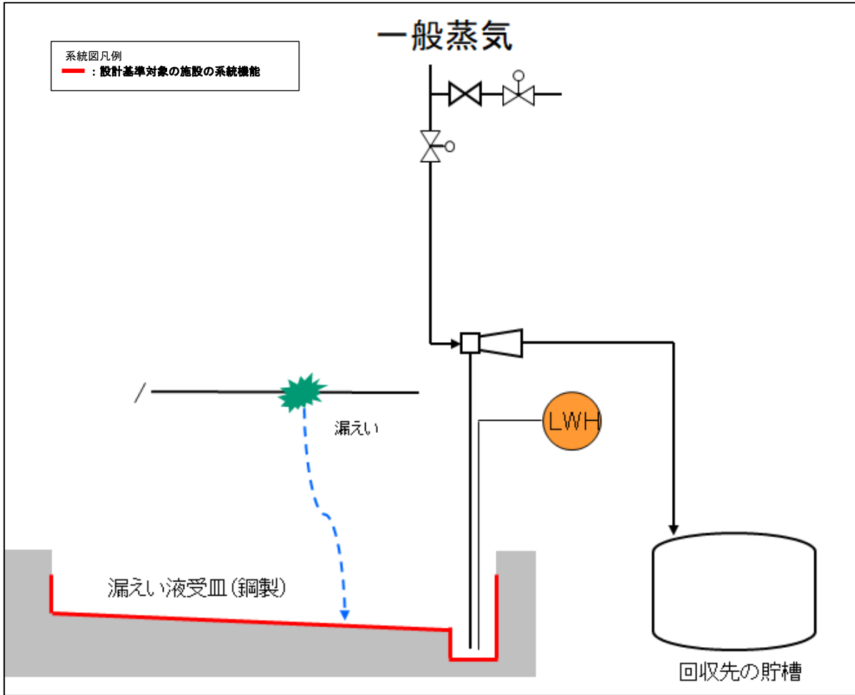
第2-5図 低レベル廃液等の漏えい液の保持（漏えいした溶液の保持）
