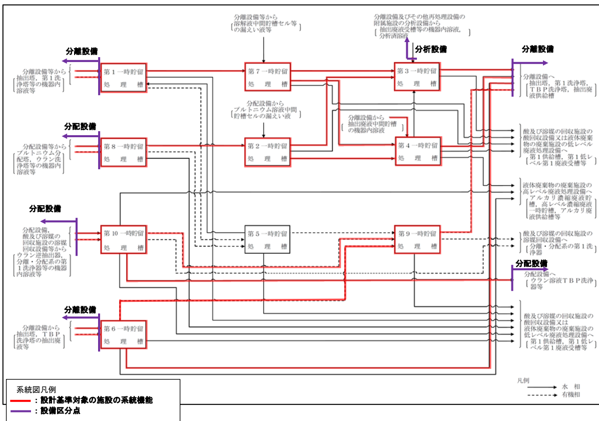
第2-1図 分離建屋一時貯留処理設備 系統概要図 (事業許可申請書 添付書類六 第4.4-2図抜粋)
