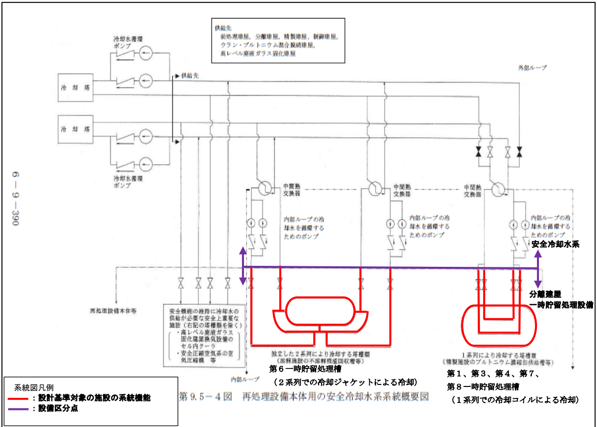
第2-2図 安全冷却水系 系統概要図 (事業変更許可申請書 添付書類六 第9.5-4図抜粋)
