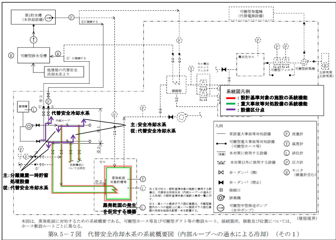
第2-7図 代替安全冷却水系 系統概要図 (内部ループへの通水による冷却) (事業変更許可申請書 添付書類六 第9.5-7図抜粋)
