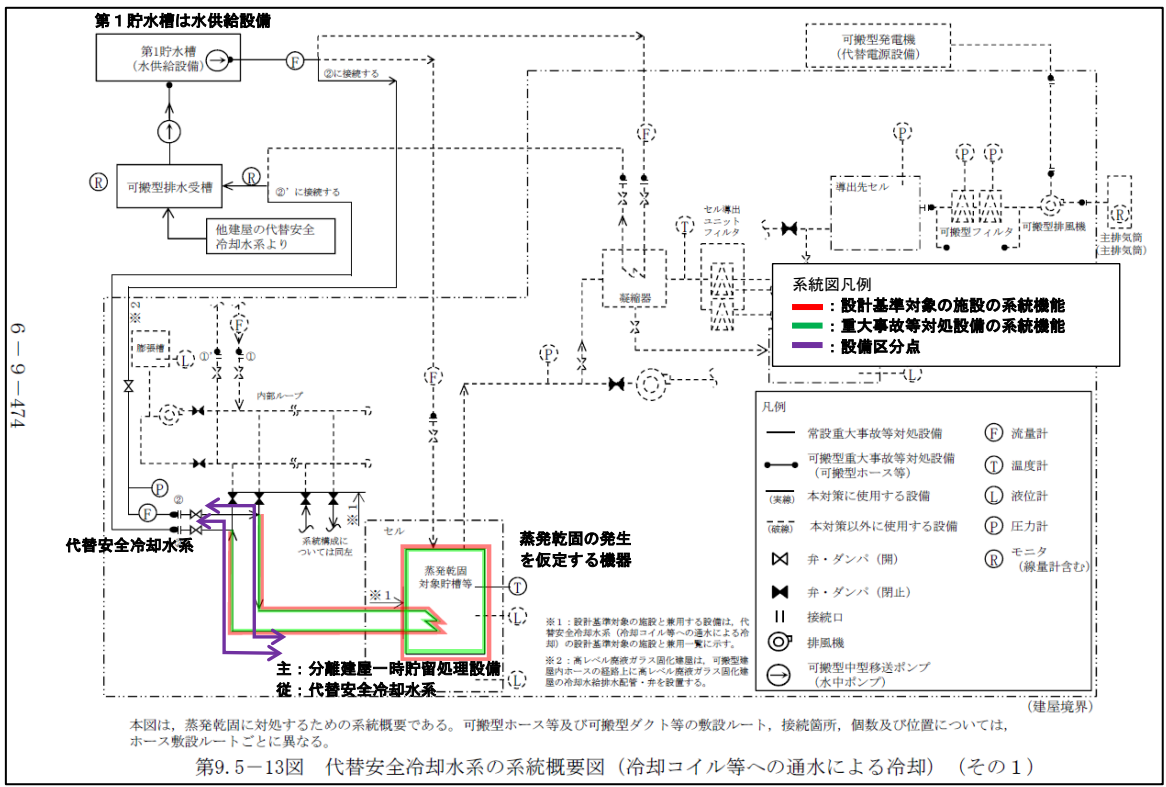
第2-9図 代替安全冷却水 系統概要図（冷却コイル等への通水による冷却） （事業変更許可申請書 添付書類六 第9.5-13図抜粋）
