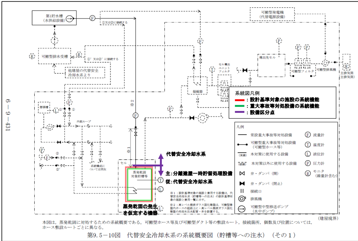
第2-8図 代替安全冷却水系 系統概要図 (貯槽等への注水) (事業変更許可申請書 添付書類六 第9.5-10図抜粋)
