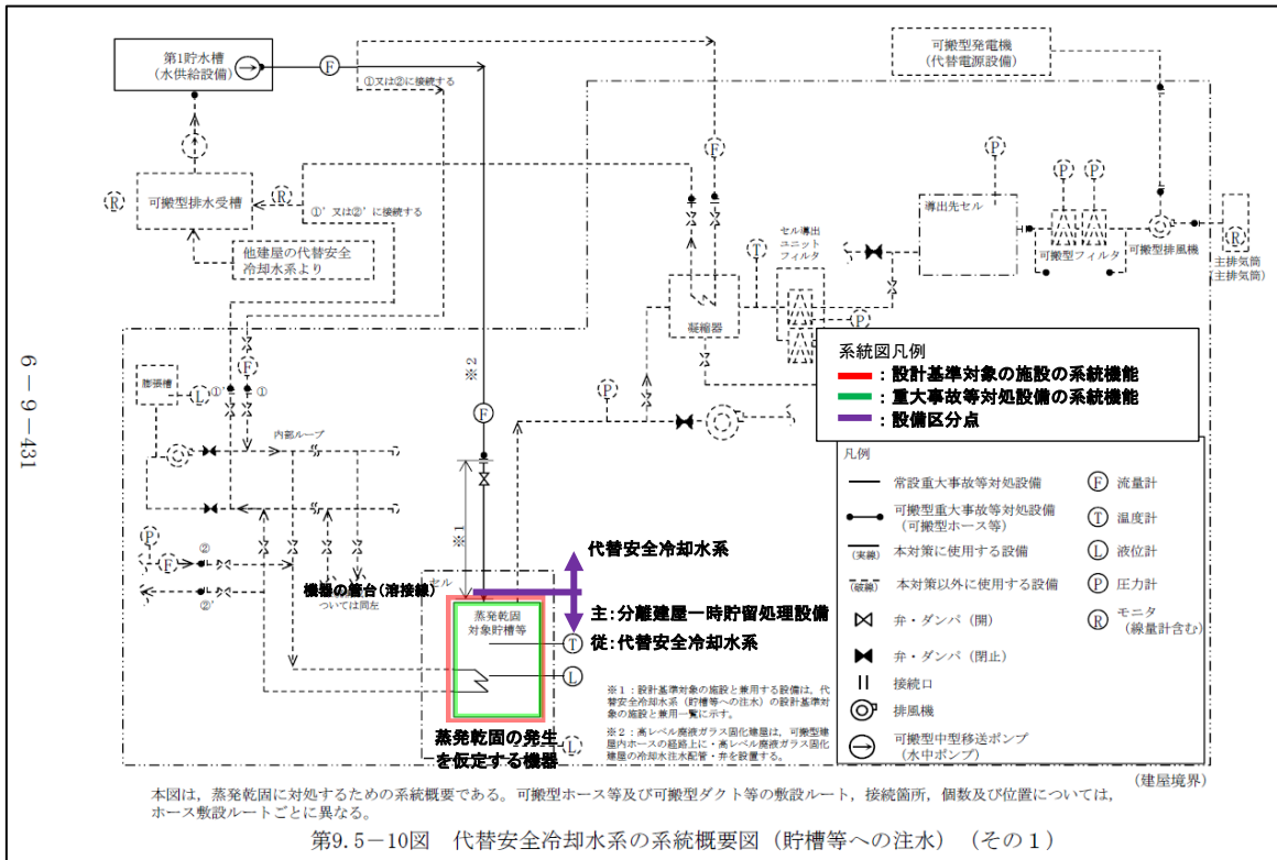
第3-7図 代替安全冷却水系 系統概要図 (貯槽等への注水) (事業変更許可申請書 添付書類六 第9.5-10図抜粋)
