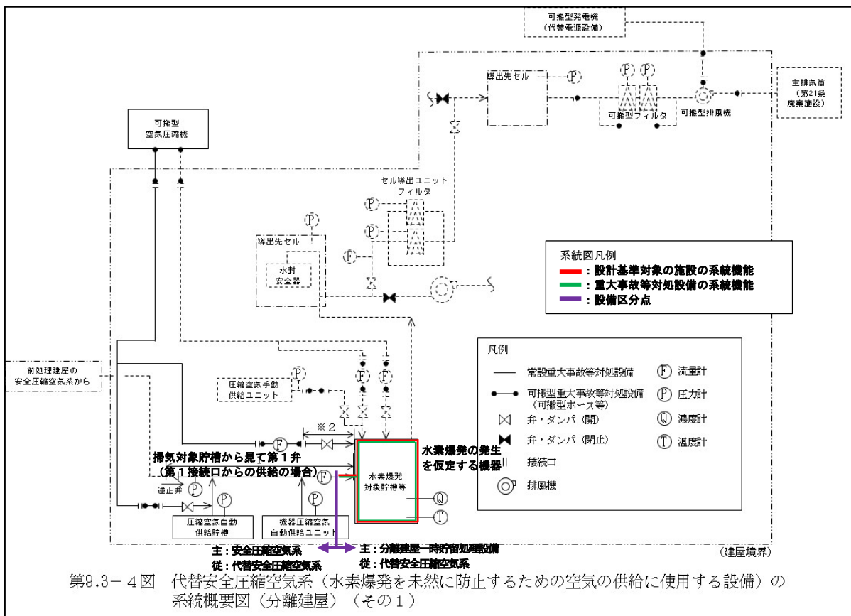
※1：水素掃気配管・弁、※2：機器圧縮空気供給配管・弁 第3-11図 代替安全圧縮空気系（水素爆発を未然に防止するための空気供給に使用する設備）の系統概要図 （事業変更許可申付書類六 第9.3-7図抜粋）
