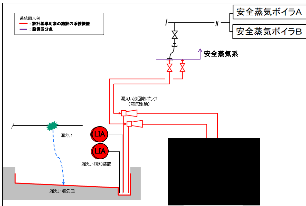
第 2 - 4 図 沸騰のおそれのある高レベル廃液等の回収
