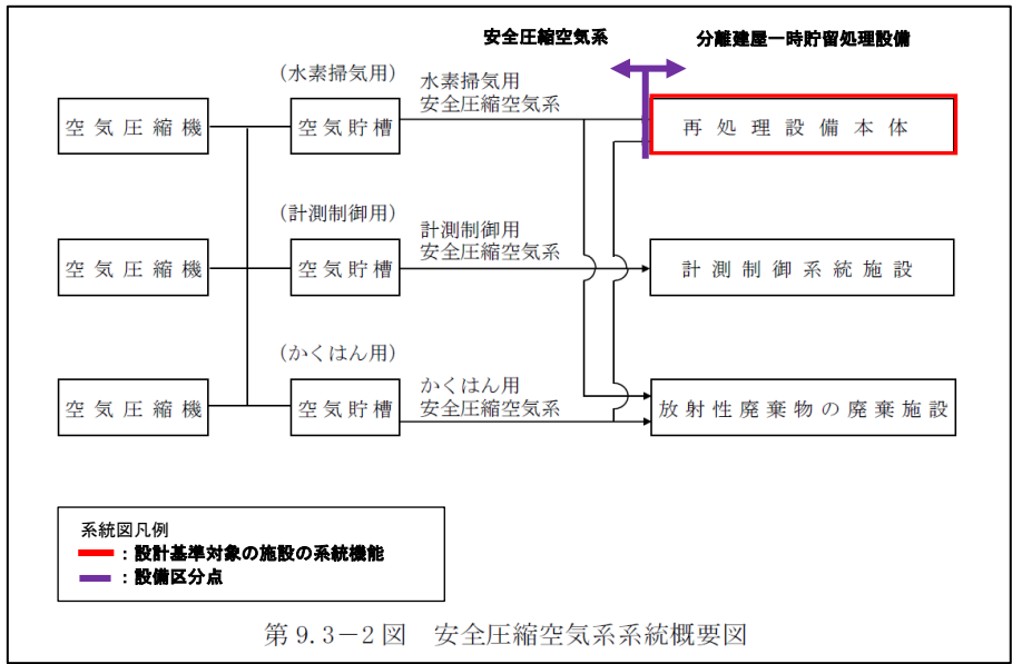
第 2 - 6 図 安全圧縮空気系 系統概要図 (事業変更許可申請書 添付書類六 第9.3-2 図抜粋)
