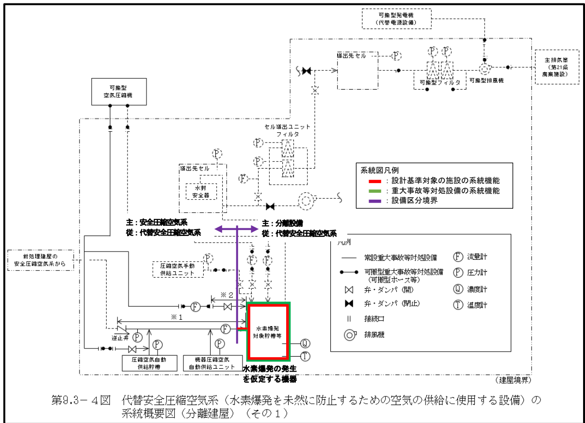
第2-16図 代替安全圧縮空気系（水素爆発を未然に防止するための空気供給に使用する設備）の系統概要図
