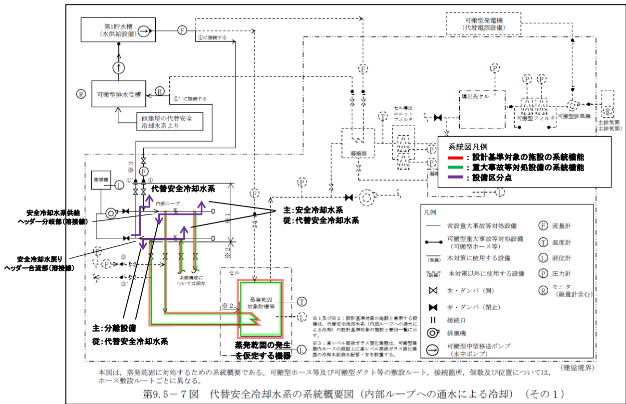
第3-9図 代替安全冷却水系 系統概要図 (内部ループ通水) (事業変更許可申請書 添付書類六 第9.5-7図抜粋)
