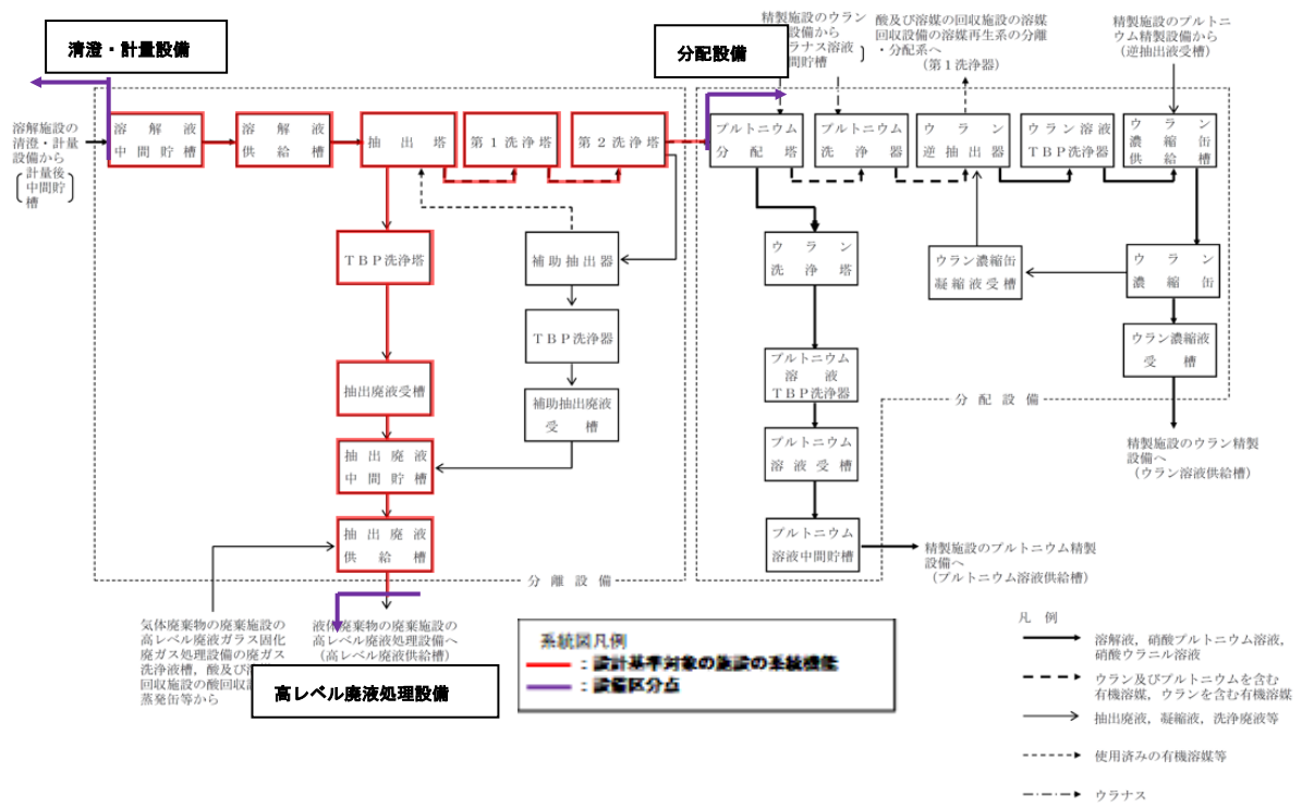
第2-1図 分離設備 系統概要図 (事業変更許可申請書 添付書類六 第4.4-1図抜粋)
