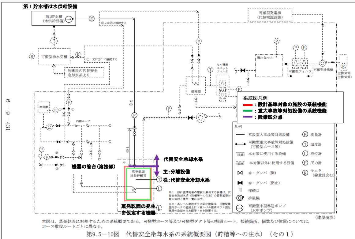
第3-10図 (1) 代替安全冷却水系 系統概要図 (事業変更許可申請書 添付書類六 第9.5-10図抜粋)
