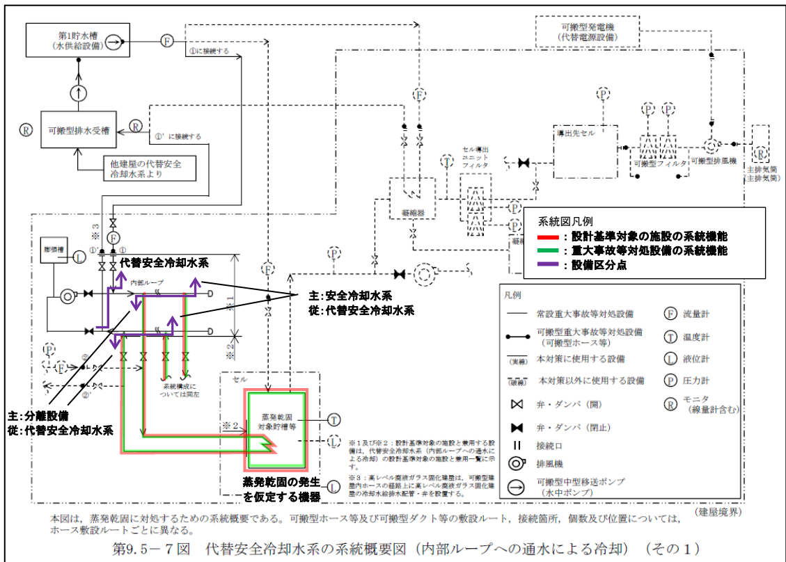
第2-12図 代替安全冷却水系 系統概要図 (内部ループへの通水による冷却) (事業変更許可申請書 添付書類六 第9.5-7図抜粋)
