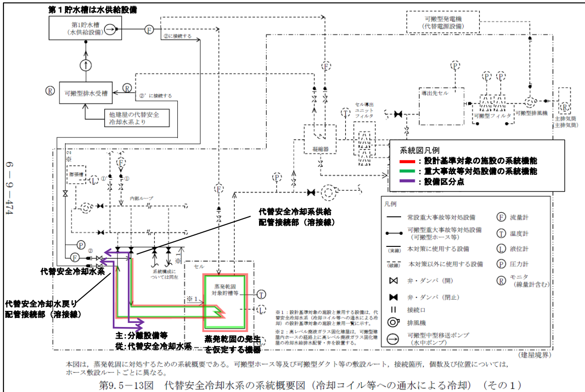
第3-12図 代替安全冷却水 系統概要図(冷却コイル等への通水による冷却) (事業変更許可申請書 添付書類六 第9.5-13図抜粋)
