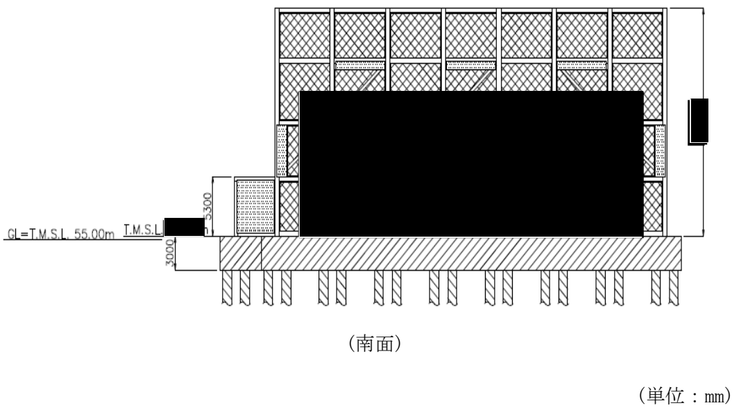
第 2.2-3 図 飛来物防護ネット架構の概略側面図 (1/2)
