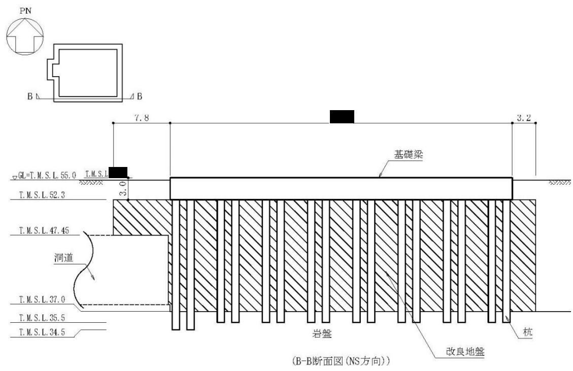
第1-4図 基礎梁及び杭の断面図(1/2)(単位：m)
