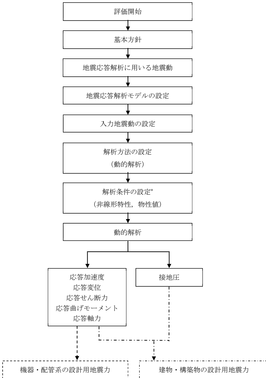
第 2.3-1 図 安全冷却水 B 冷却塔基礎の地震応答解析フロー
