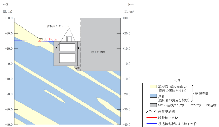
図 3.3-30 低圧代替注水ポンプ格納槽の地下水位分布 (南北：ポンプ室)
