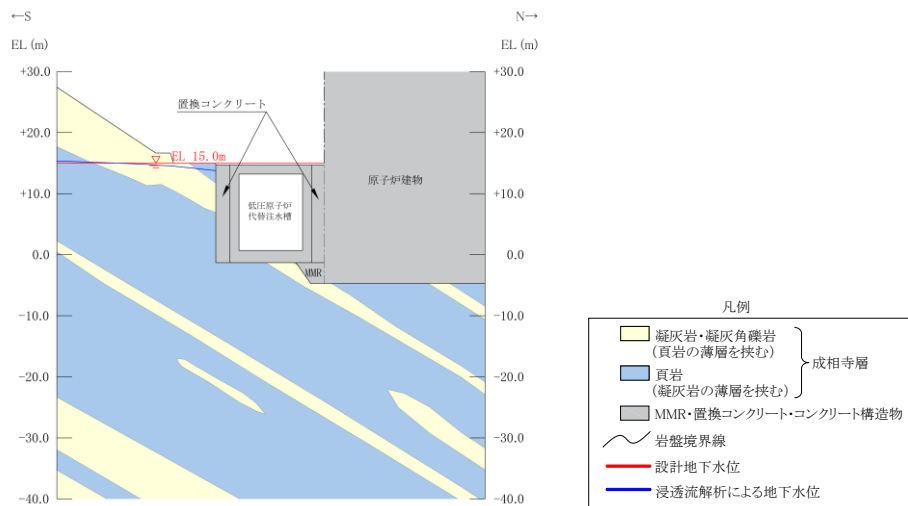
図 3.3-29 低圧代替注水ポンプ格納槽の地下水位分布 (南北：水室)
