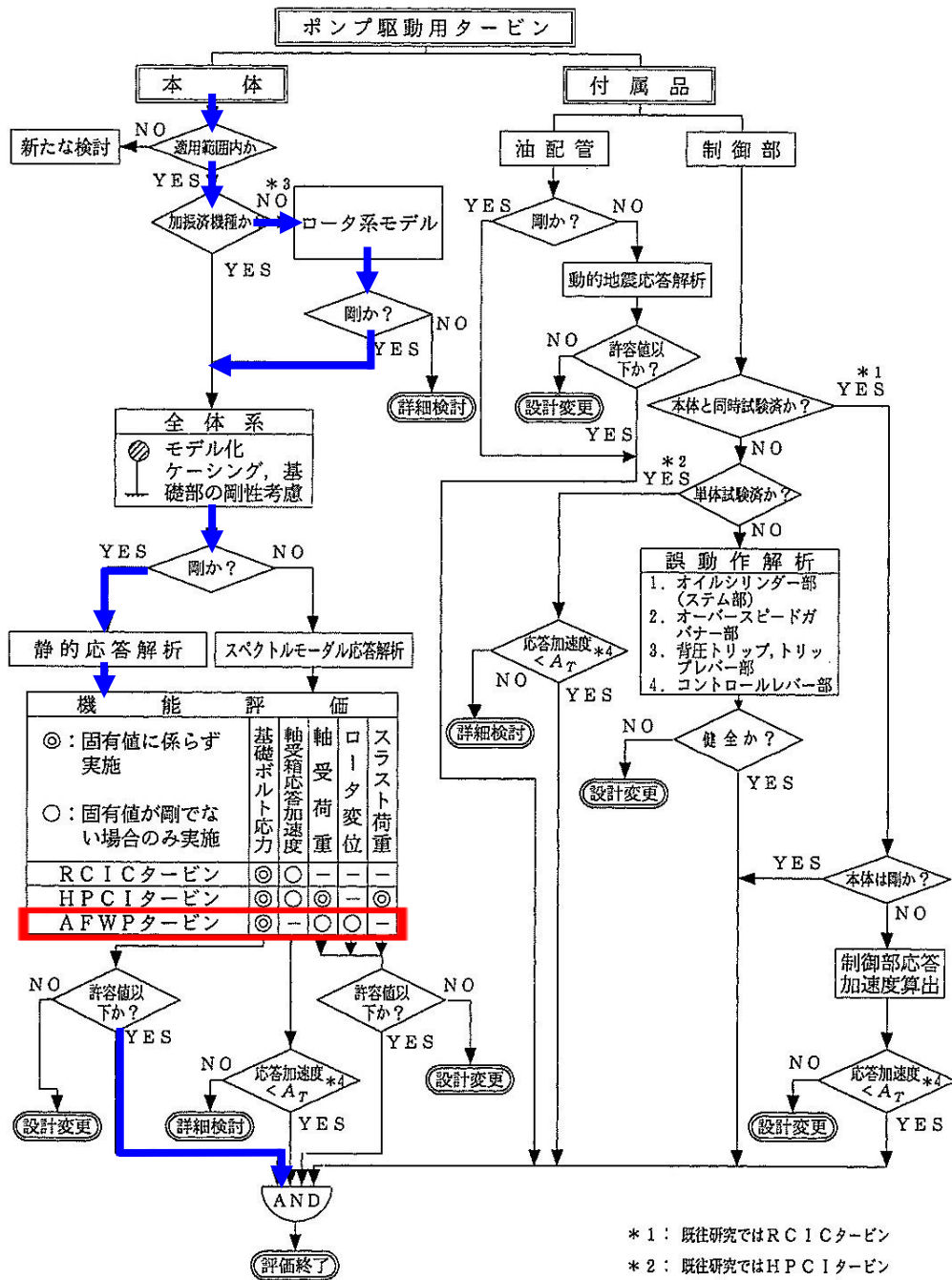
別紙 1-22 図 ポンプ駆動用タービンの評価手順 (JEAG 4601-1991 追補版)
