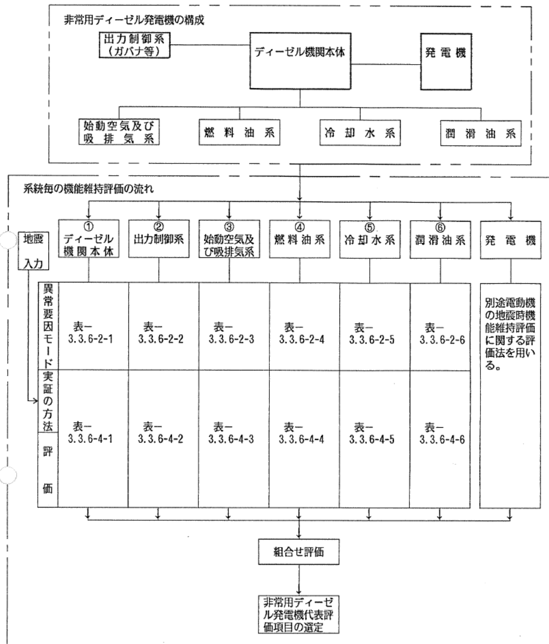
別紙 1-14 図 非常用ディーゼル発電機の構成と機能維持評価の流れ (耐特委)
