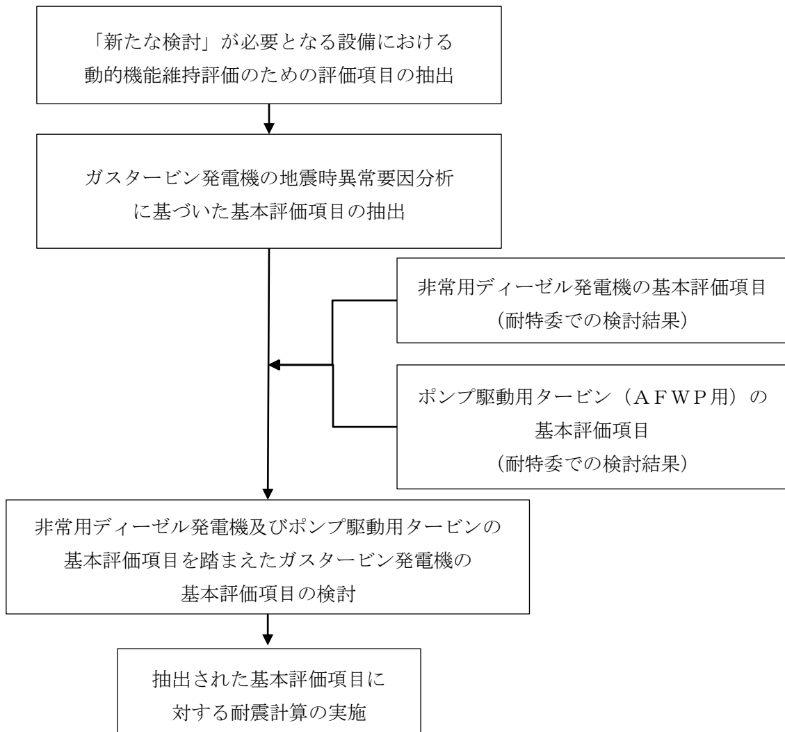
別紙1-5図 動的機能維持評価のための基本評価項目の抽出フロー
