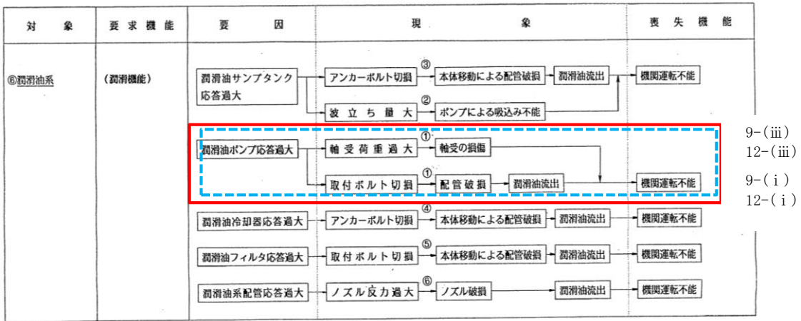
別紙 1-19 図 非常用ディーゼル発電機の異常要因分析図 (冷却水系)
