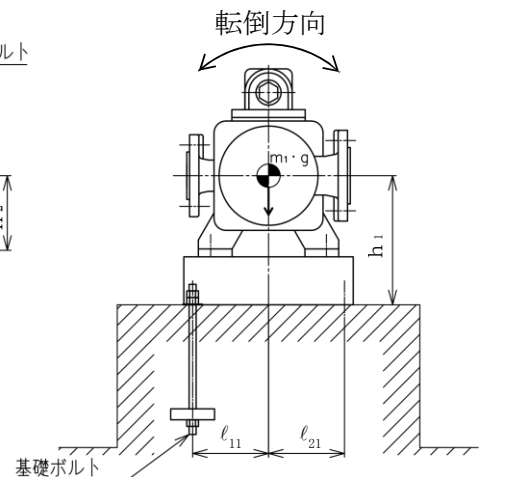
B~B 矢視図 (基礎ボルト) (l_{11} \leq l_{21})
