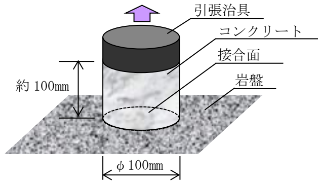
図 4-6 試験体の概要 (直接引張試験)
