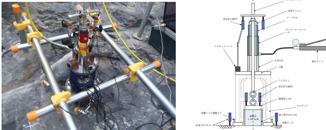
図 4-8 付着力試験装置の概要 (直接引張試験)
