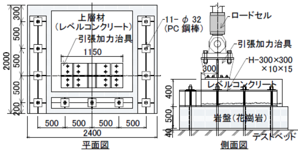
図3-8 加力方法
