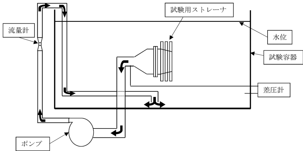
図 3-3 試験概要図
